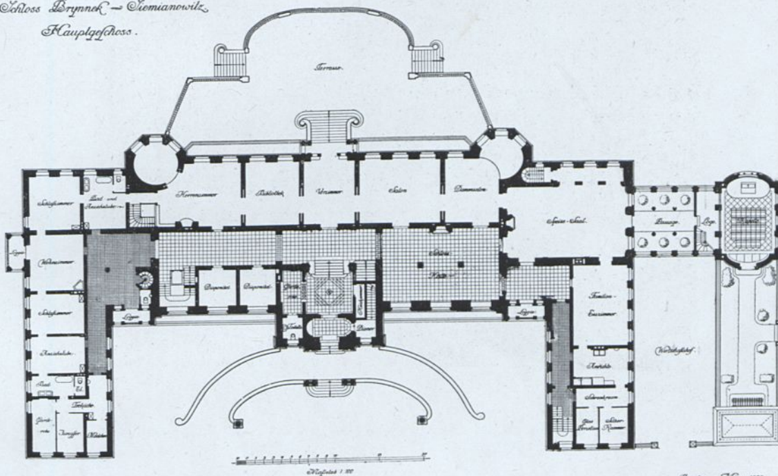
GRUNDRISS DES HAUPTGESCHOSSES
