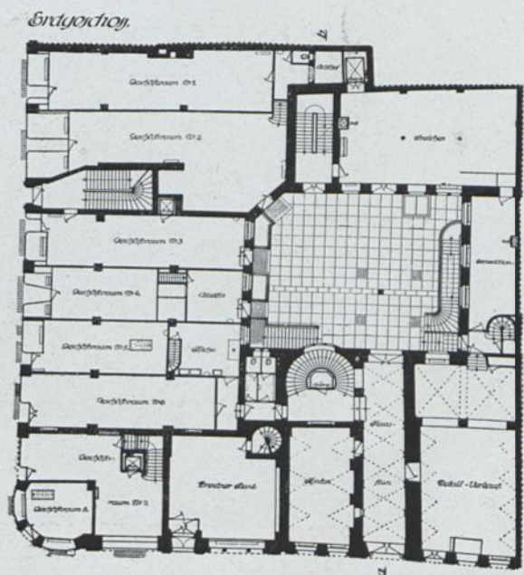
GRUNDRISS NACH DEM UMBAU
