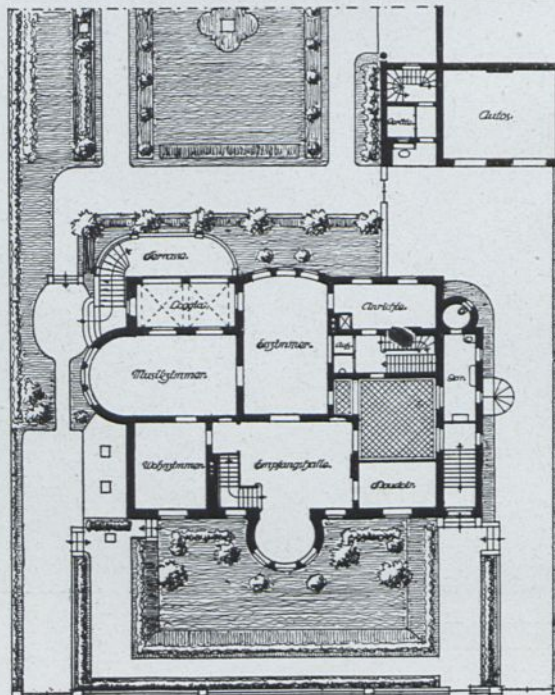
GRUNDRISS VOM HAUPTGESCHOSS
