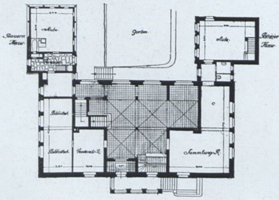
HAUPTGESCHOSS
