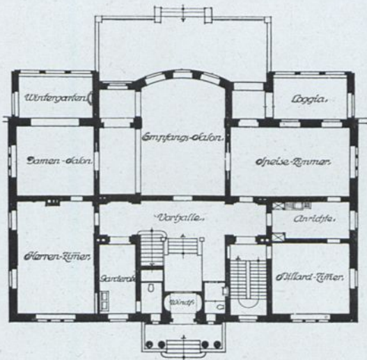
HAUPTGESCHOSS
