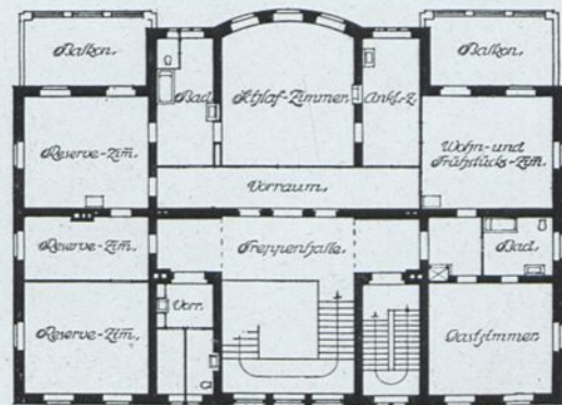
OBERGESCHOSS
