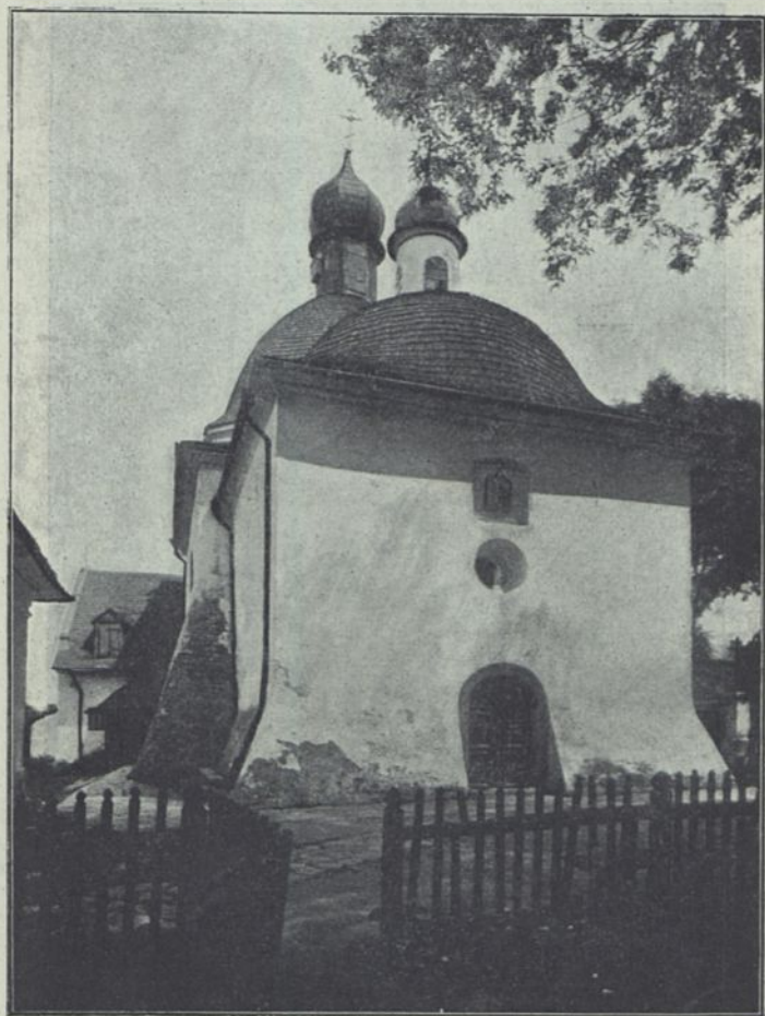
Fig. 16. Cerkiewka św. Mikołaja w Gródku Jagiellońskim. Przykład dodatni krycia gontem budowli murowanych.
