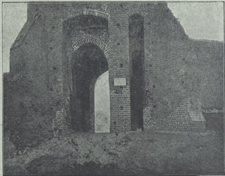
Fig. 18. Fragment ruin zamku Czerskiego. Przykład dodatni naprawy znaczniejszych uszkodzeń murów.
