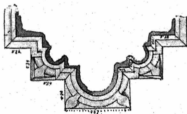
Fig. 4. Filar pośredni od strony nawy bocznej.
