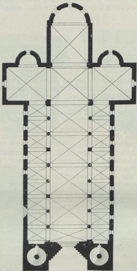
Fig. 274. Grundriß des Domes zu Goslar.
