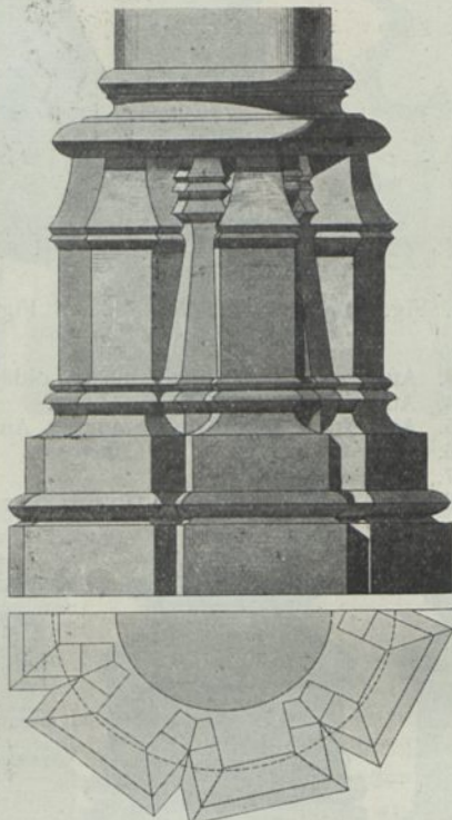
Fig. 212. Vom südlichen Kreuzflügel der Zisterzienserabtei Maulbronn.
