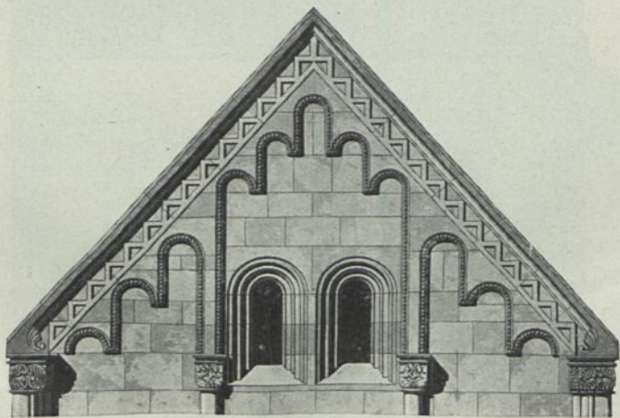
Fig. 89. Giebel von der Walderichskapelle zu Murrhardt.
