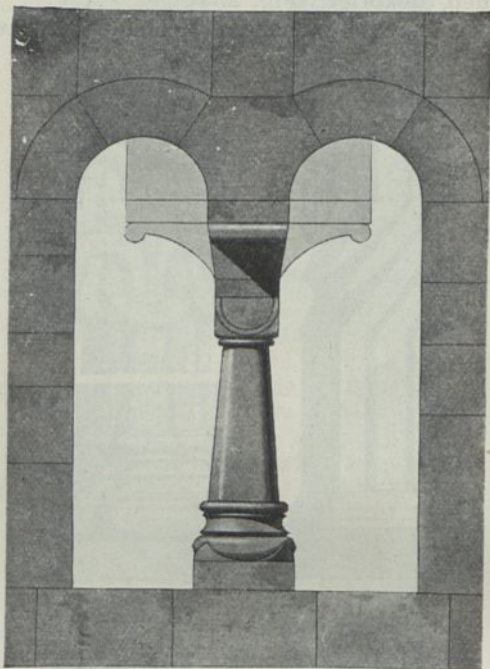
Fig. 237. Turmfenster der Kirche zu Nufringen (Württemberg).
