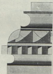
Fig. 9. Hauptgesims vom Neumünster in Würzburg.
