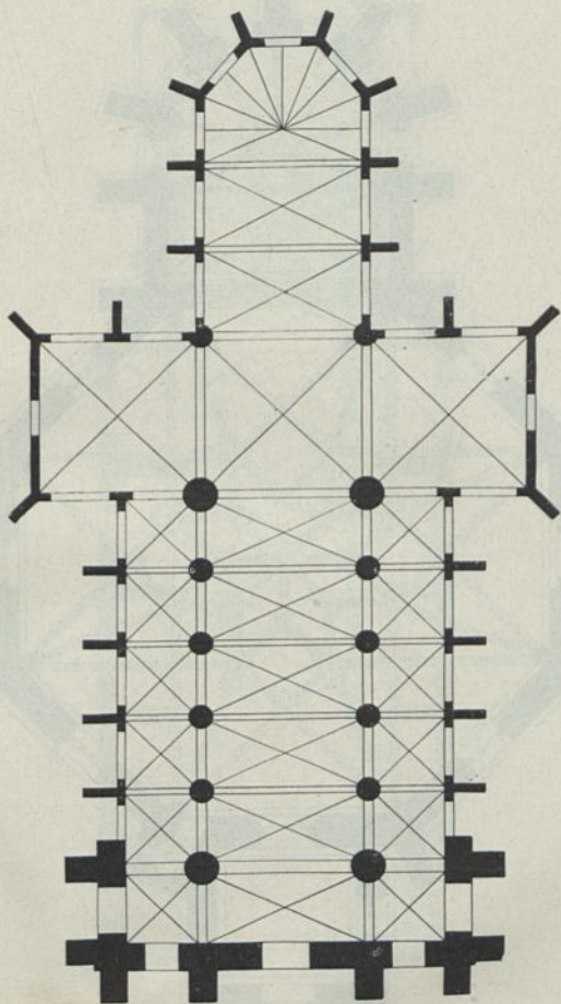
Fig. 276. Schema des gotischen Kirchenbaues.
