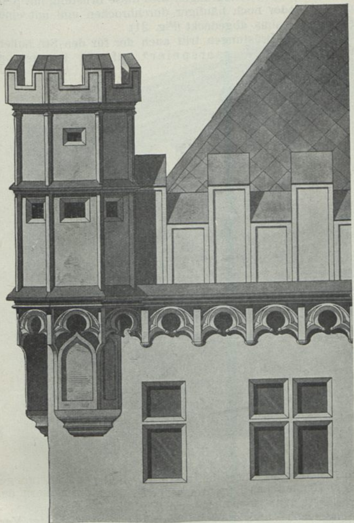
Fig. 20. Vom steinernen Haus zu Frankfurt a. Main.
