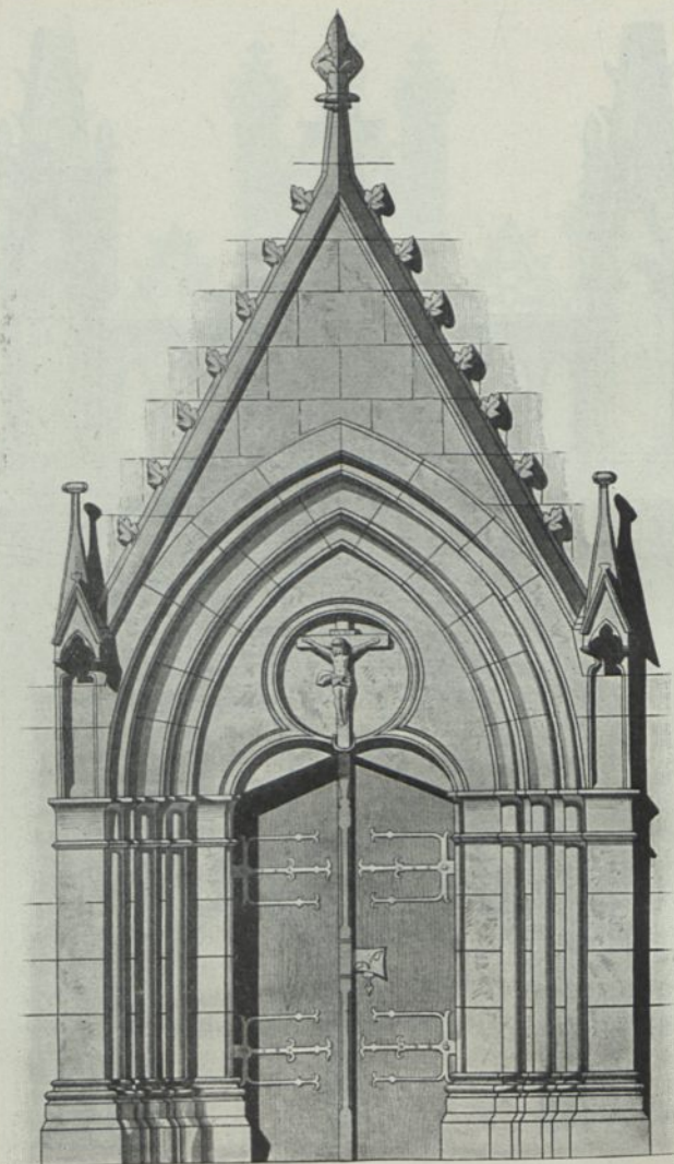
Fig. 97. Wimperg über dem Portal der Kirche zu Wolfhagen.
