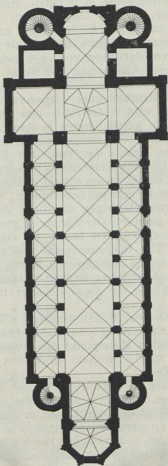
Fig. 275. Grundriß des Domès zu Worms.
