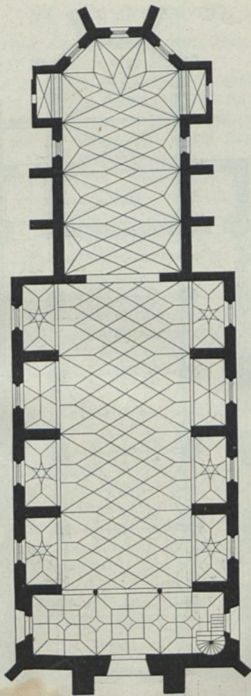
Fig. 278. Grundriß der Stadtkirche zu Schwaigern in Württemberg.
