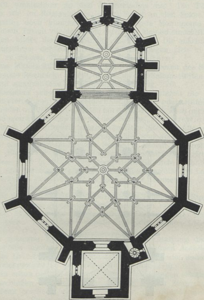
Fig. 277. Grundriß der Karlsbofokirche zu Prag.
