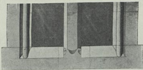
Fig. 128. Fensterbank vom Freiburger Münster.
