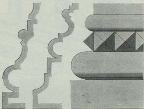
Fig. 23. Von St. Jakob in Regensburg.
