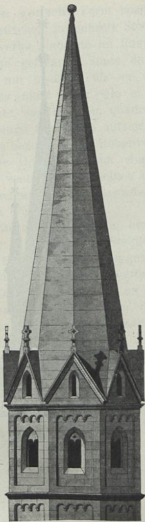
Fig. 104. Turmhelm von St. Maria zu Gelnhausen.
