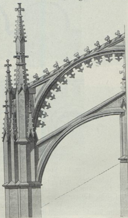
Fig. 41. Von der Barbarakirche zu Kuttenberg (Böhmen).
