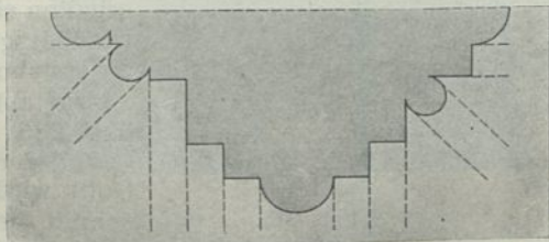
Fig. 219. Schema des entwickelten romanischen Pfeilers.
