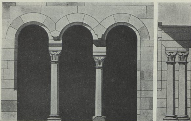
Fig. 131. Turmfenster der Stiftskirche zu Oberstenfeld (Württemberg).
