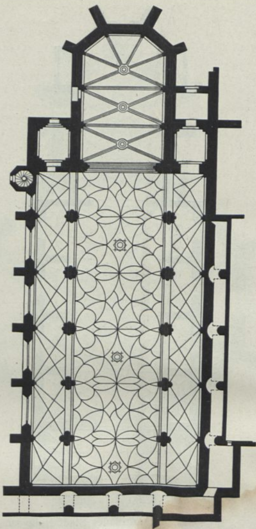
Fig. 279. Grundriß der Kirche zu Göß in Steiermark.
