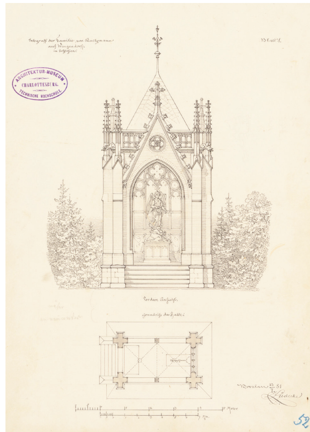
II. 3. Elewacja frontowa i rzut mauzoleum – druga wersja projektu Lüdeckego z 1881 r. (źródło: TUBAM Inv. Nr. 6044)
