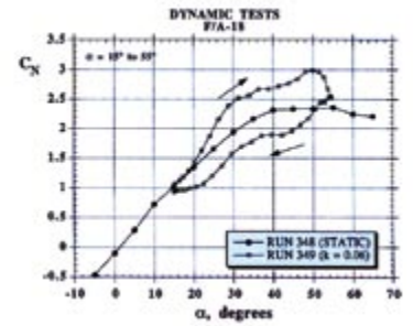
Współczynnik sił normalnej modelu samolotu F/A-18
