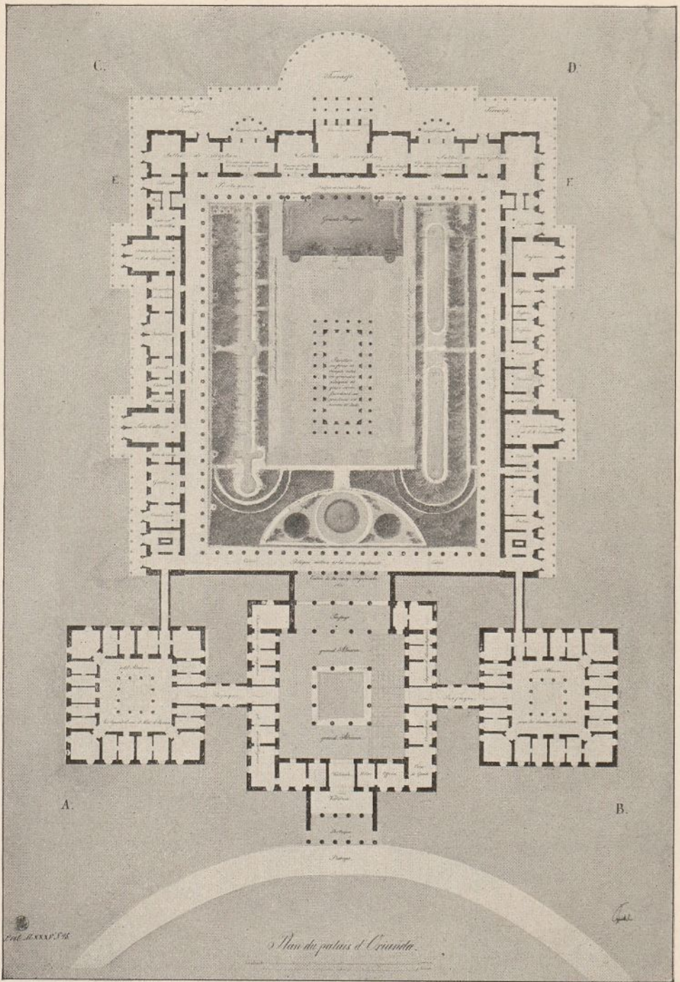
Abb. 121. Entwurf zu dem Schloß Orianda auf der Krim für die Kaiserin von Rußland. Grundriß. 1838. (Aquarell).
