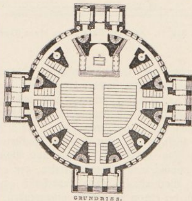
Abb. 75. Viertes Entwurf zu einer Kirche für die Dranienburger Vorstadt in Berlin. Grundriß. 1828.
