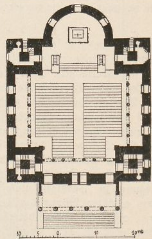
Abb. 92. Die Nicolaitirche in Potsdam. Grundriß. 1830.
