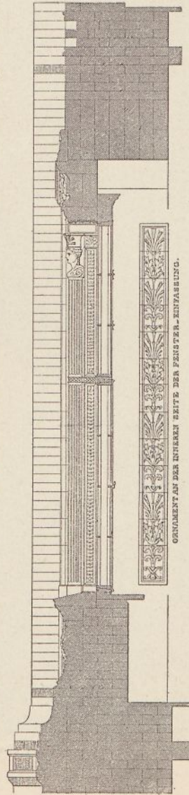
Abb. 99. Die Bauakademie in Berlin. Ansicht und Profil eines Fensters des ersten Hauptgeschosses. 1831.
