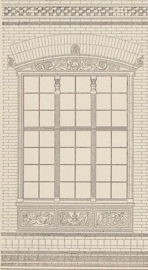
Abb. 99. Die Bauakademie in Berlin. Ansicht und Profil eines Fensters des ersten Hauptgeschosses. 1831.
