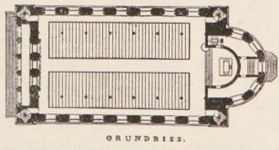
Abb. 74. Dritter Entwurf zu einer Kirche für die Dranienburger Vorstadt in Berlin. Grundriß. 1828.
