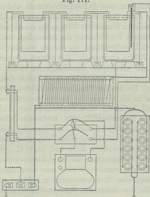
Versuchsanordnung zur Prüfung von Accumulatoren.
