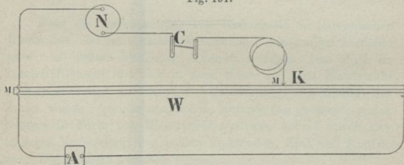
Schema für Spannungsmessung.
