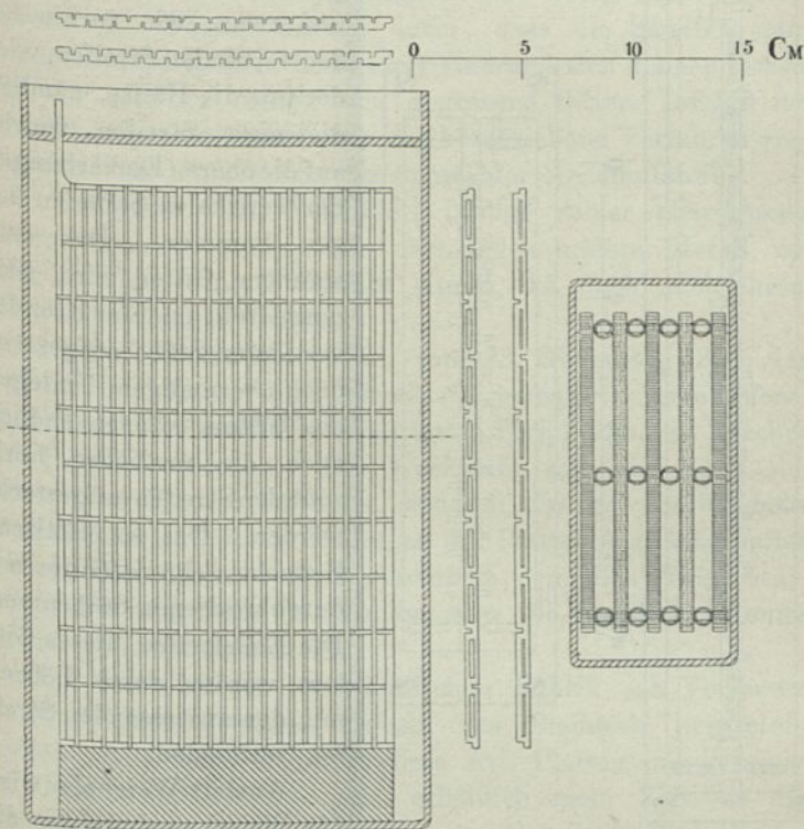
Gestanzte Bleistreifen und Kompositgitter mit durchbrochenen Stäben.
