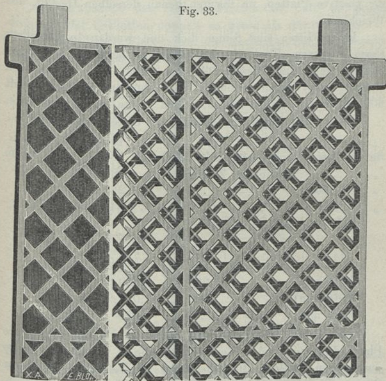
Gitter von C. Wilh. Kayser & Co., Berlin (natürl. Grösse).
