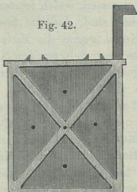
Platten der Berliner Accumulatoren-Fabrik.
