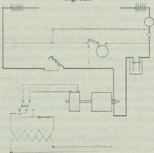
Schalt-schema für Wechselstrom.
