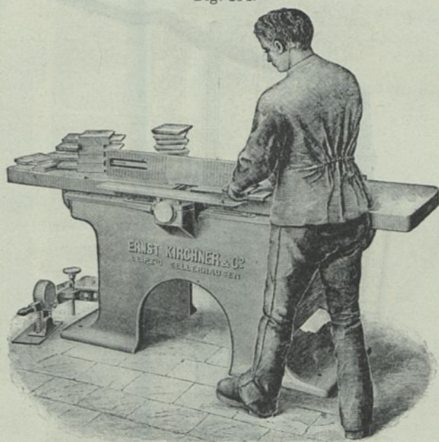
Hobel- und Abrichtmaschine. (Kirchner &amp; Co., Leipzig.)
