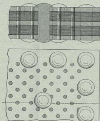
Main-Platte.
