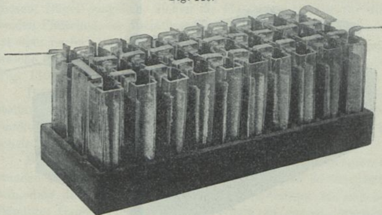
Messbatterie mit 30 Volt Spannung.
