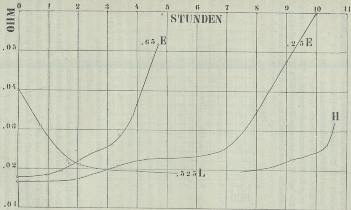
Widerstandskurven von Nernst-Hagen.
