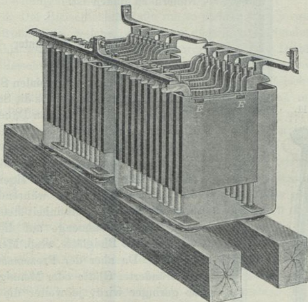
Anschluss der Platten an Bleileisten.
