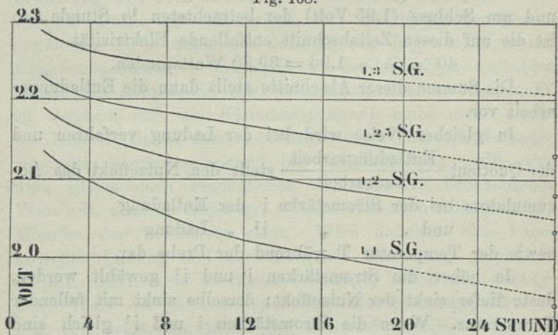
Abfall der elektromot. Kraft beim vollgeladenen Accumulator.
