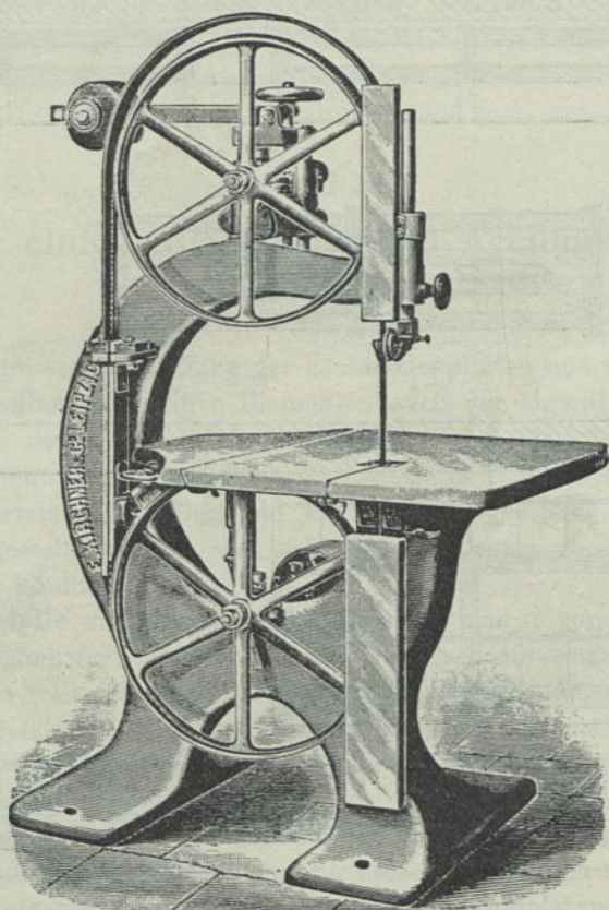
Bandsäge. (Kirchner &amp; Co., Leipzig.)
