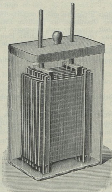
Accumulator der Watt-Accumulatoren-Werke, Berlin.
