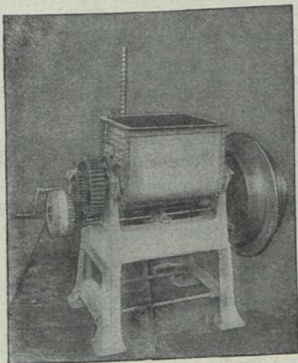
Misch- und Knetmaschine mit umkippbarem Mischtrog von Werner & Pfeleiderer.
