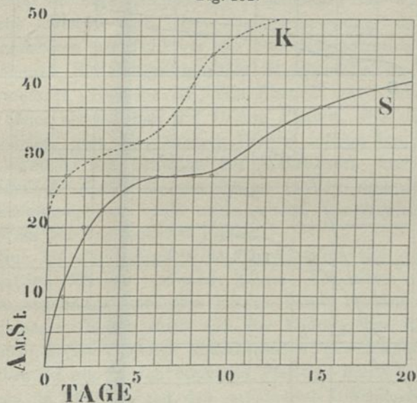
Kapazität von Superoxydschichten.
