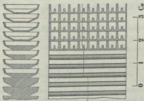
Schema der Schulze-Platte.
