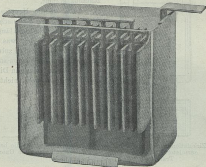
Accumulator mit symmetrischer Stromführung.
