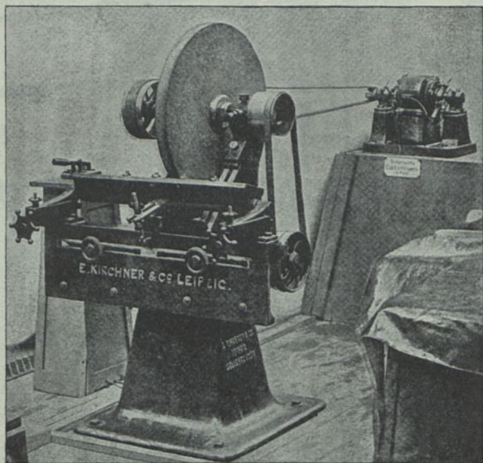
Hobelmesser-Schärfmaschine (Kirchner &amp; Co., Leipzig).
