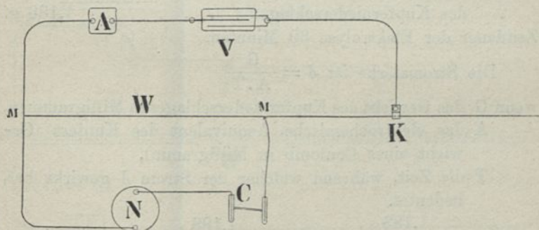
Schema für die Kalibrierung des Messbandes (Ampère).
