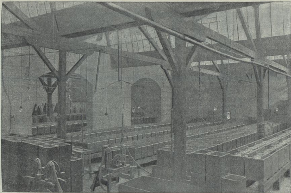
Formierraum der Kölner Accumulatorenwerke G. Hagen, Kalk.
