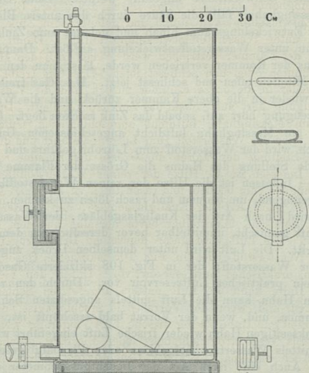
Wasserstoffentwickler.
