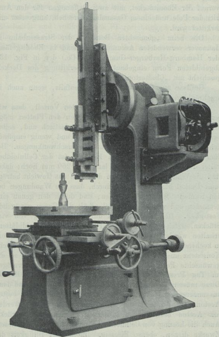
Hobelmaschine (Maschinenfabrik Oerlikon).
