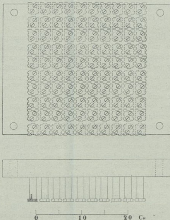
Untersicht und Seitenansicht des Stempels.
