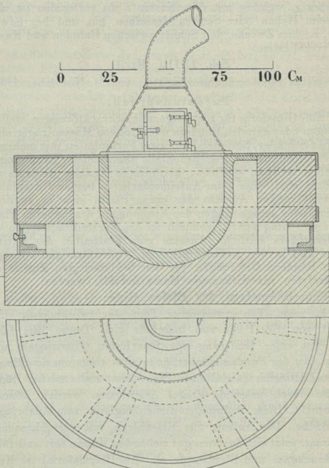
Bleischmelzöfen.
