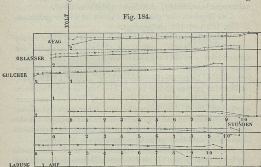
Elektromotorische Kräfte und Klemmenspannungen an den einzelnen Elektroden bei 7 Ampère Ladung.
