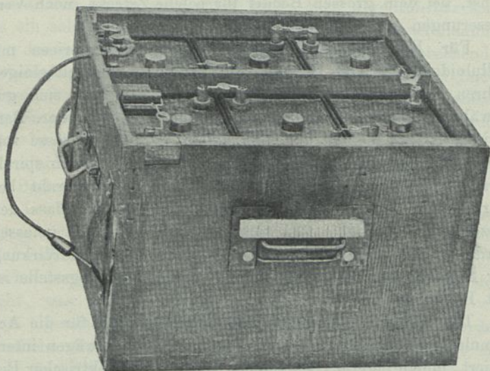
Batterie für Eisenbahnwagenbeleuchtung.
