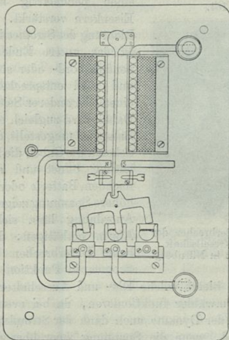
Automat (nach Dietrich-Hospitalier.)
