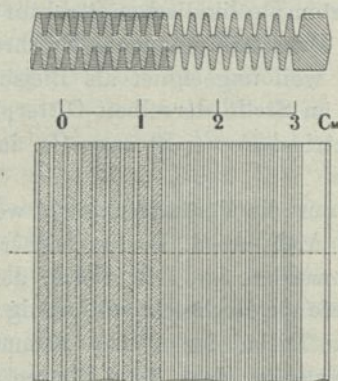
A.-F.-A.-G.-Platte (1891).
