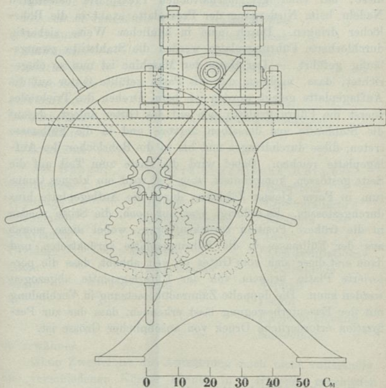
Perforiermaschine. Vorderansicht.
