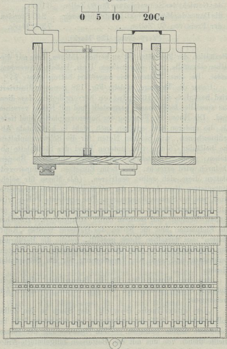
Accumulator A 17 der Kölner Accumulatorenwerke.
