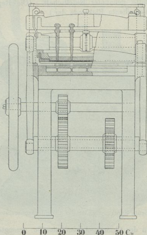
Perforiermaschine. Seitenansicht und Querschnitt.
