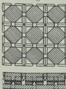
Teil-Querschnitte durch beide Gussformhälften.
