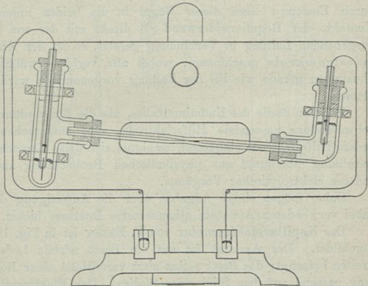
Kapillar-Elektrometer von F. Exner, Wien.
