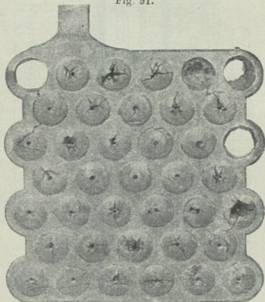
Ausgediente Superoxydplatte der Chloride-Accumulator-Co.
