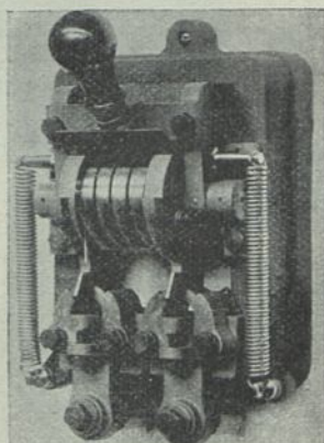
Automatischer Unterbrecher der Elektrizitätsgesellschaft vormals Schuckert & Co., Nürnberg.
