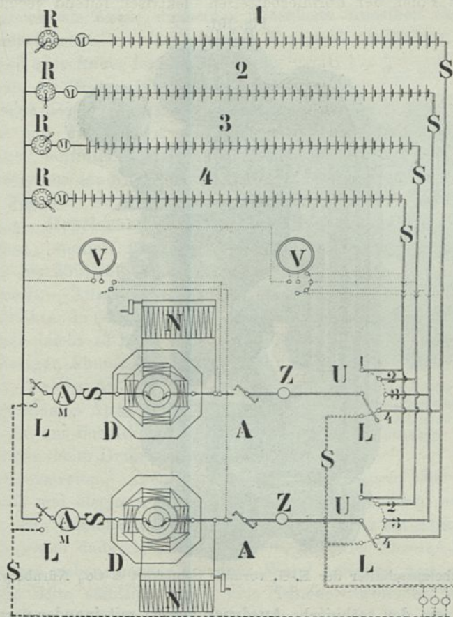
Schaltungsschema.
