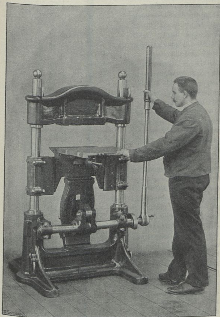
Kniehebelpresse von K. Krause, Leipzig.
