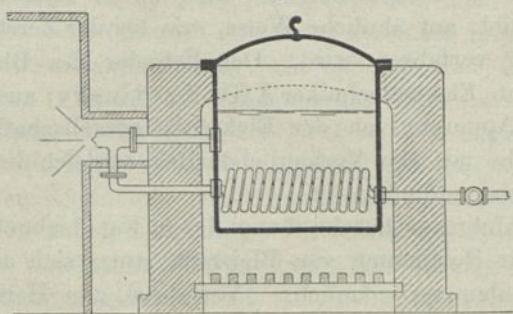
Bleistaubapparat.
