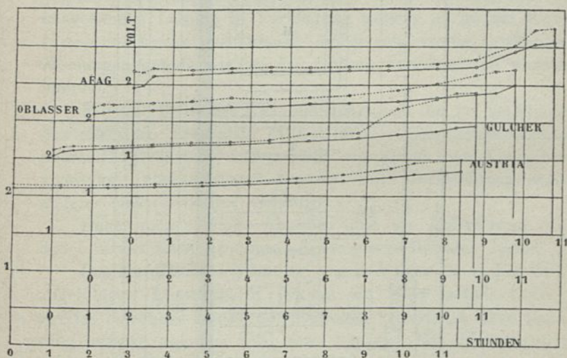
Elektromotorische Kraft und Klemmenspannungen der Elemente bei 7 Ampère Ladung.
