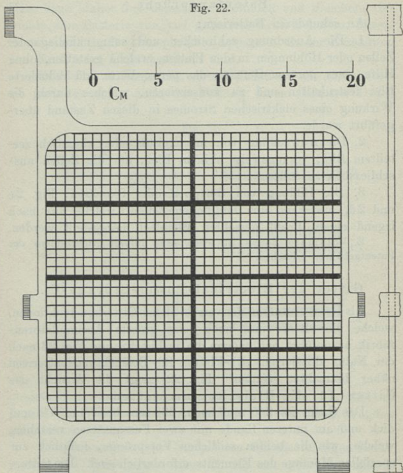
Bleischwammgitter der E.-P.-S.-Co. (1887.)
