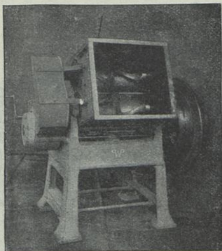
Misch- und Knetmaschine mit umklipbarem Mischtrog von Werner & Pfeiderer.
