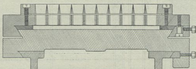
Querschnitt durch den Pastapparat nach der Breite.
