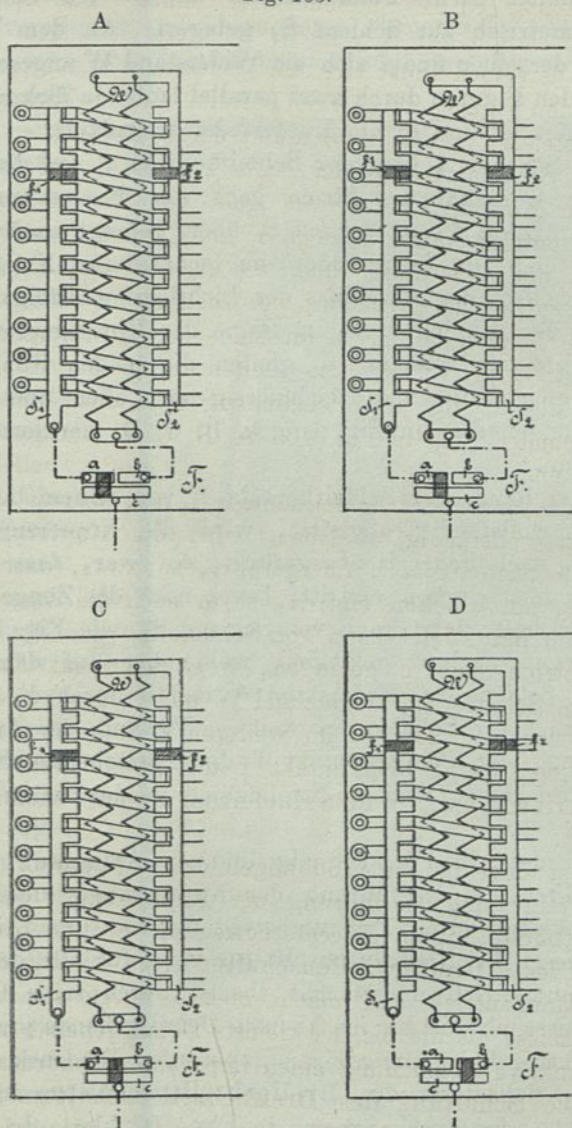
Spezielschema des Funkenlöschers.
