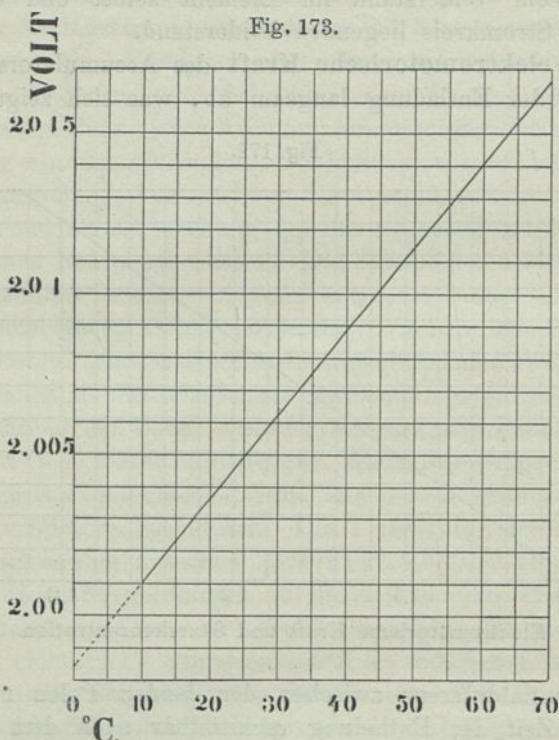
Elektromotorische Kraft und Temperatur.
