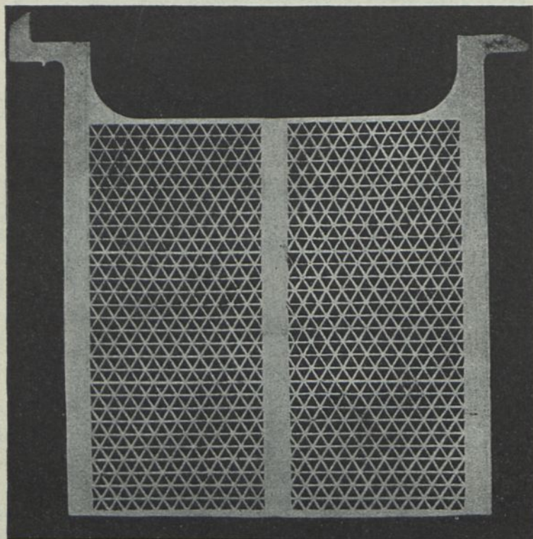
Dreieckgitter mit Hohlkehlen zur Führung der Glasrohre.
