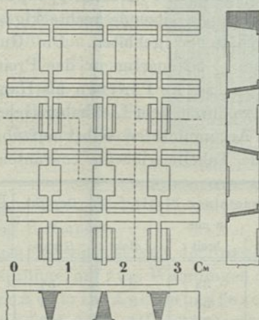
Gitter von Hladik, Grunewaldt &amp; Co., Berlin.
