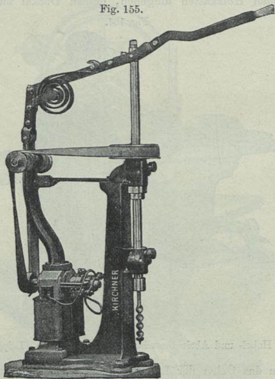
Bohrmaschine. (Kirchner &amp; Co., Leipzig.)
