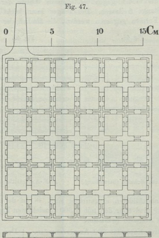
Superoxydgitter von W. &amp; R. Baden (bei Wien.)
