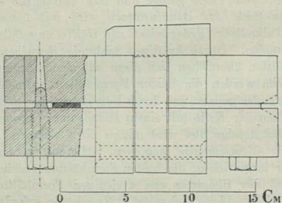
Gussform, Seitenansicht.
