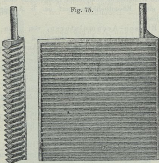
Winkler-Platte.
