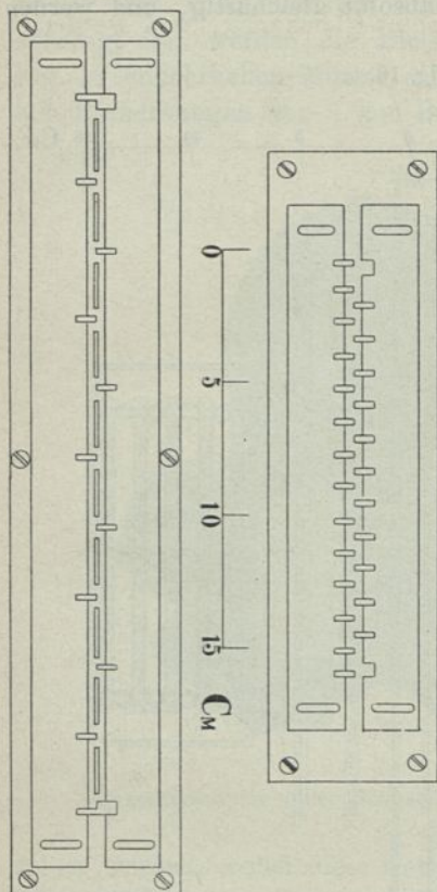
Matrizen für Schnitte.
