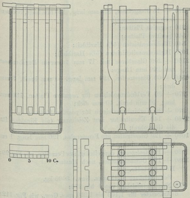
Element mit symmetrischer Stromführung.
