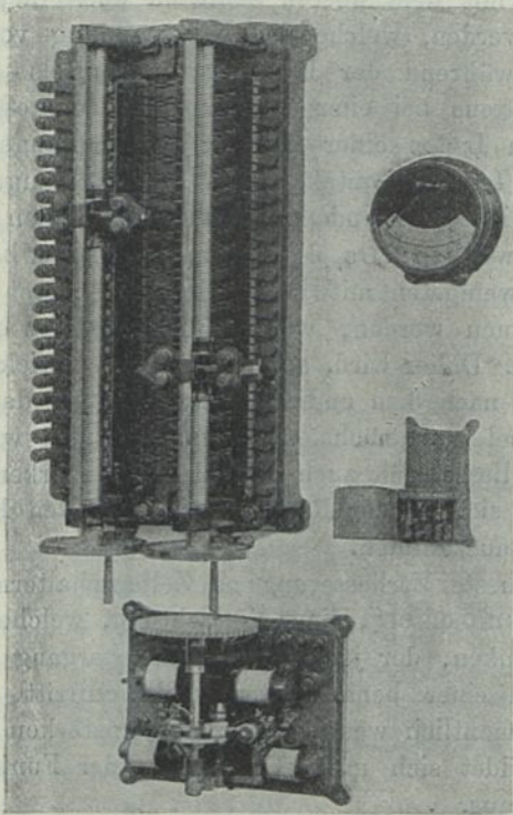
Doppelzellenschalter mit selbstthätigem Antrieb der Elektrizitäts-Gesellschaft vorm. Schuckert & Co. in Nürnberg.
