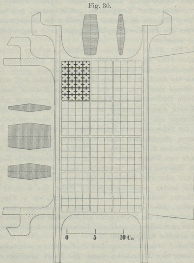
Spanisches Gitter.
