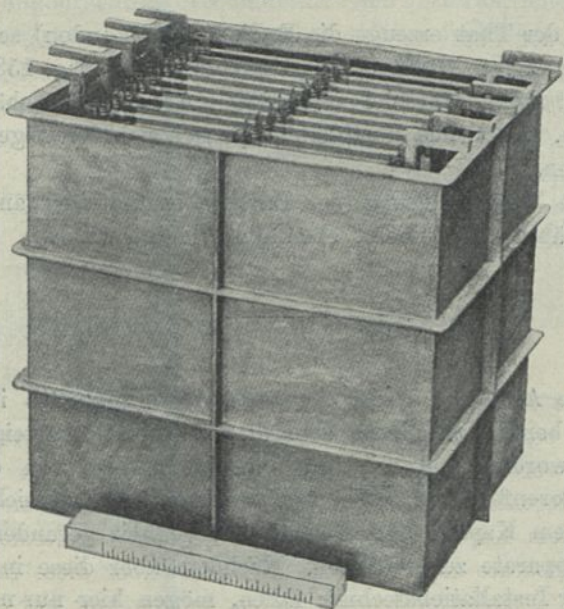
Accumulator mit Hartbleigefäss.
