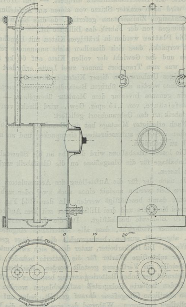
Wasserstoff-Apparat für Transport.
