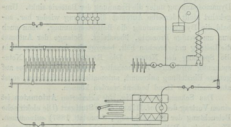
Schaltungsschema.
