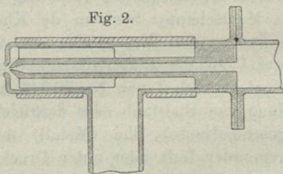
Düse.
