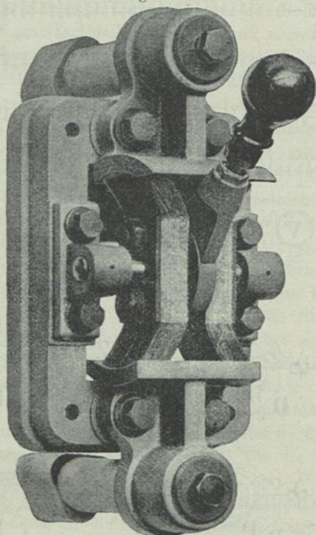
Hebelausschalter der E.-G. vormals Schuckert & Co., Nürnberg.
