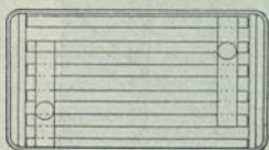
Zirkulationseinrichtung für Accumulatoren in elektrischen Tramwagen.
