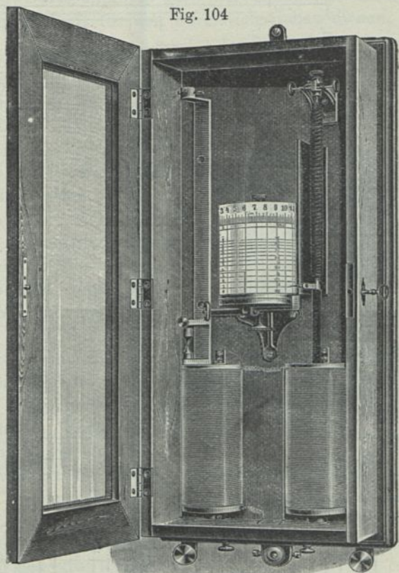
Registrierender Spannungsmesser von Hartmann & Braun, Bockenheim-Frankfurt.
