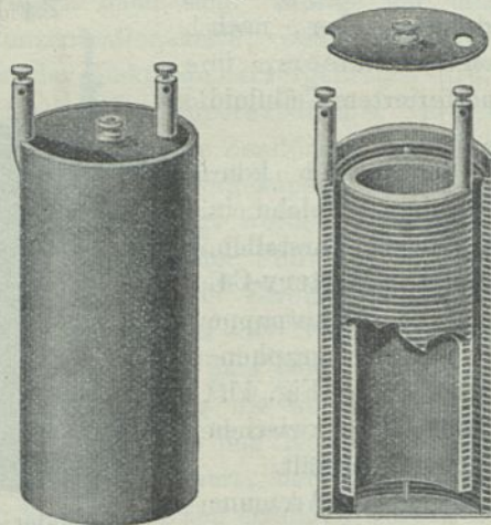
Konzentrischer Accumulator.
