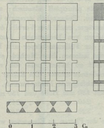
Gitter der Kölner Accumulatoren-Werke.
