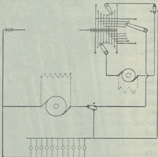
Schaltschema.
