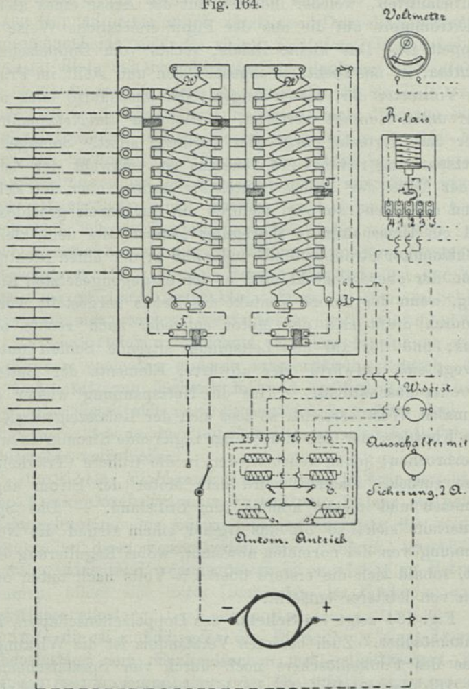
Schema des Doppelzellenschalters mit Funkenlöscher der Elektrizitäts-Gesellschaft vorm. Schuckert & Co. in Nürnberg.
