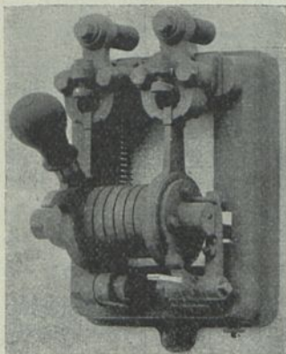
Starkstrom-Unterbrecher der Elektrizitäts-Gesellschaft vorm. Schuckert in Nürnberg.
