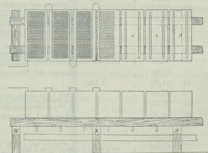
Anordnung der Formiergefäße.
