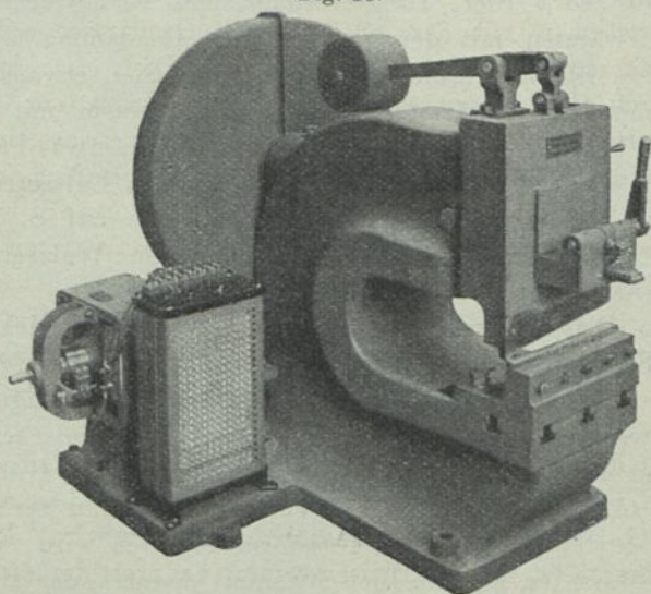
Exzenterpresse (oder Stanze). Maschinenfabrik Oerlikon.
