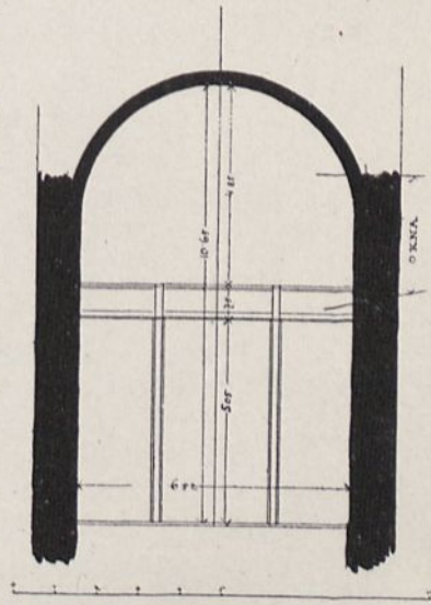
Fig. 189. Zwierzyniec. Kościół ś. Salwatora; przekrój pionowy poprzeczny.
