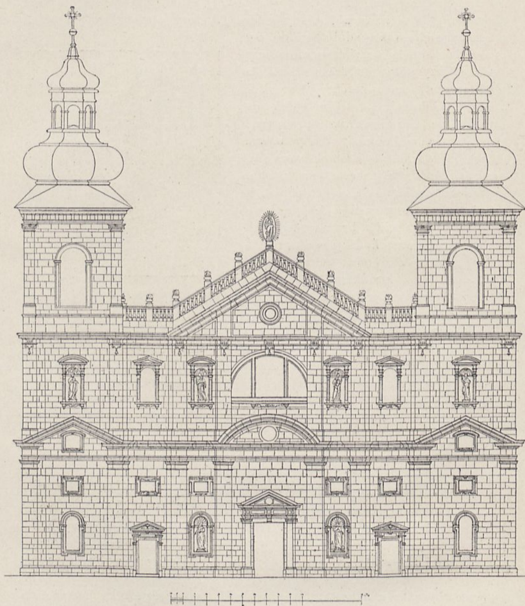
Fig. 6. Bielany. Elewacja fasady kościoła.
