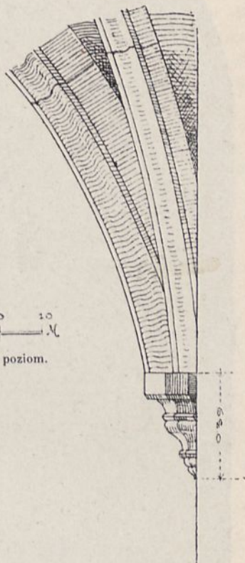
Fig. 40. Bolechowice. Spływ nózek żeber w zakrystyi.
