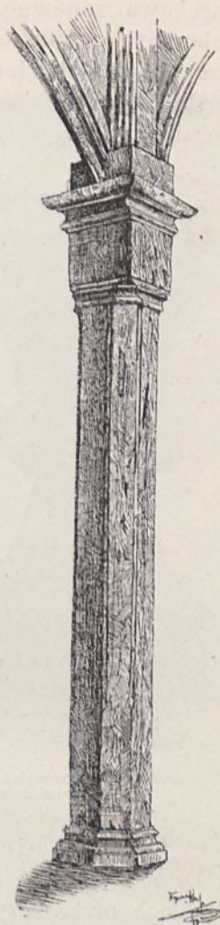
Fig. 87. Mogiła. Widok słupa drewnianego w kościele paraf.
