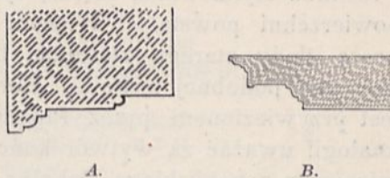
Fig. 74. Karniowice. Szczegóły odrzwi kaplicy. A. Przekrój węgarku, B. Przekrój karczamu.
