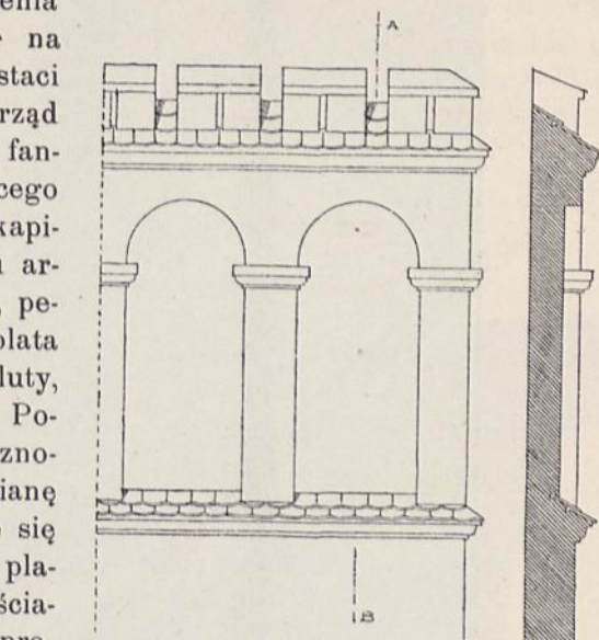
Fig. 48. Branice. Szczegół attyki lamusa.
