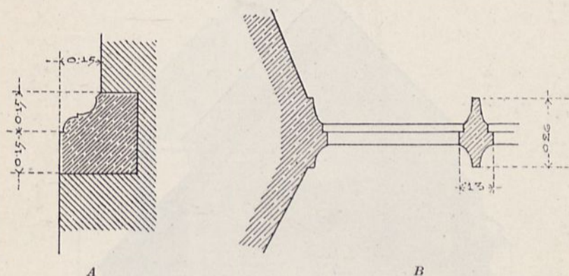
Fig. 145. Raciborowice. A Profil cokołu nawy i kruchty południowej. B Rzut poziomy okna kościelnego.
