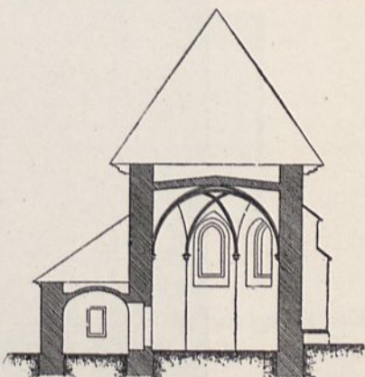
Fig. 176. Zielonki. Przekrój przez prezbiterium kościoła.
