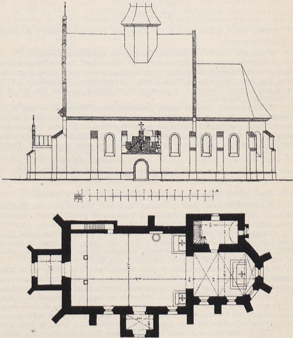
Fig. 175. Zielonki. Przekrój podłużny i rzut poziomy kościoła.
