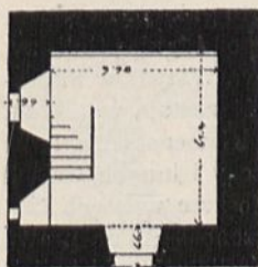
Fig. 155. Raciborowice. Rzut poziomy mурwanej części dzwonnicy.
