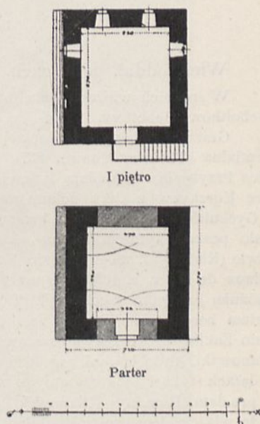
Fig. 68. Garlica murowana. Rzut poziomy parteru i I piętra lamusa.
