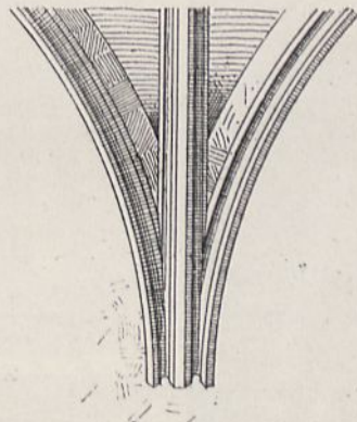
Fig. 164. Ruszcza. System spływu żeber w nawie bocznej kościoła paraf.
