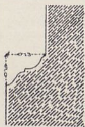
Fig. 56. Czernichów. Okrój cokołu kościoła.
