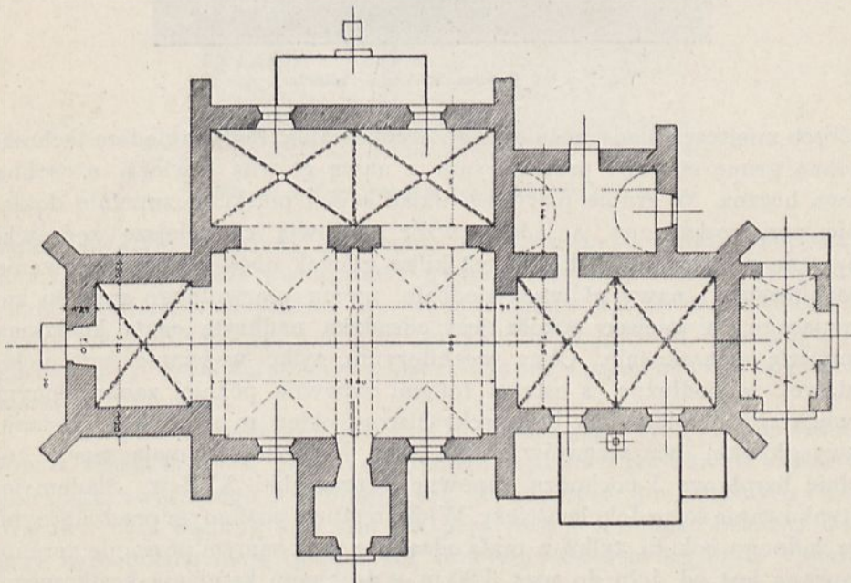
Fig. 156. Ruszcza. Przekrój podłużny i rzut poziomy kościoła. Skala służy do wszystkich zdjęć elewacji i przekroju tego budynku.
