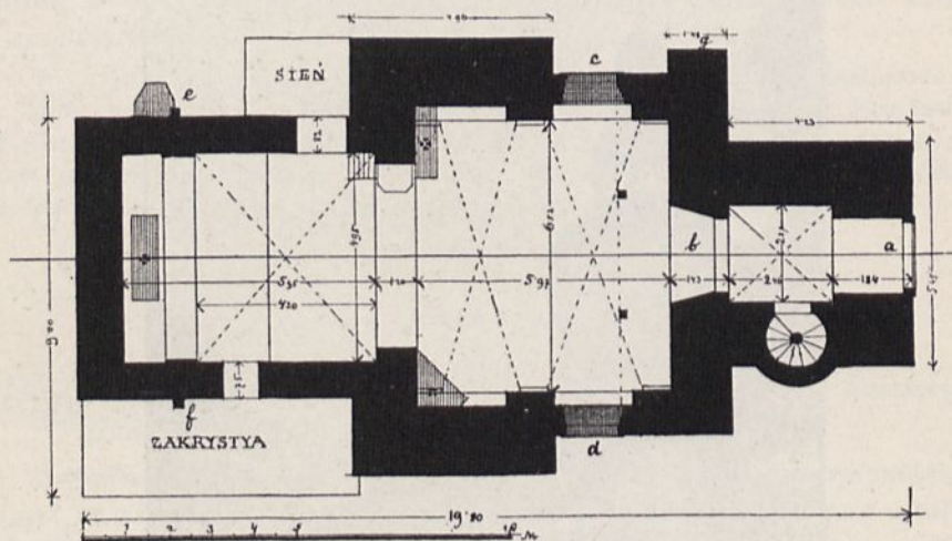
Fig. 187. Zwierzyniec. Kościół ś. Salvatora; rzut poziomy.
