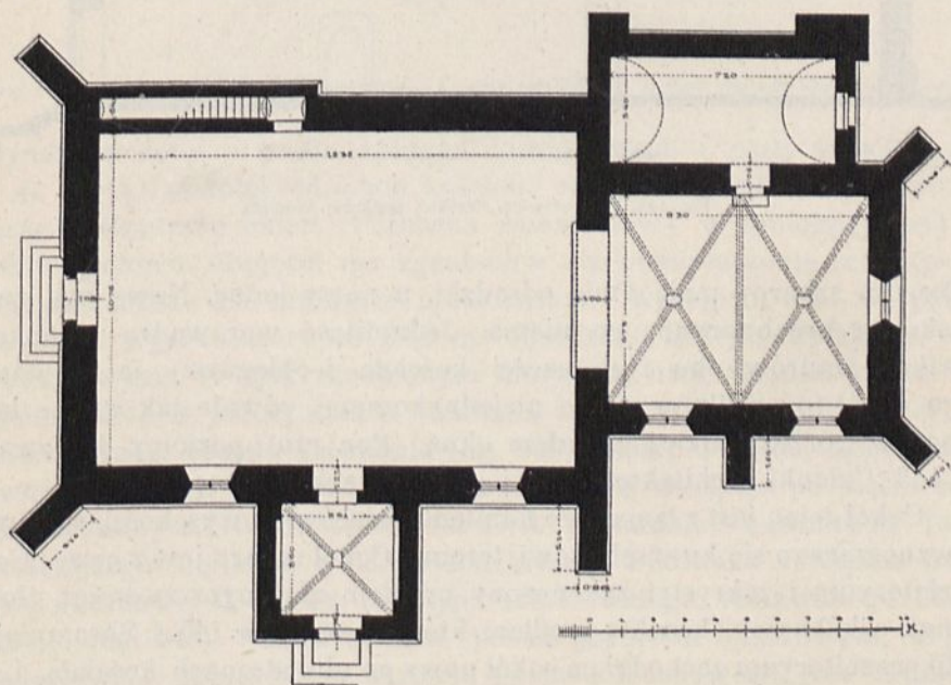
Fig. 143. Raciborowice. Elewacya fasady bocznej i rzut poziomy kościoła. (Skala służy do wszystkich zdjęć architektonicznych całości kościoła).
