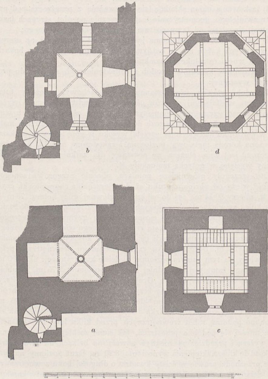
Fig. 2. Rzuty poziome: a przyziemia, b II piętra, c V piętra, d IX piętra.
