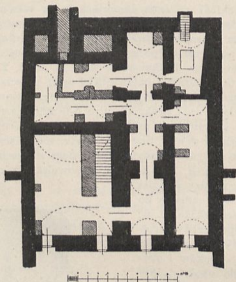
Fig. 2. Balice. Stare piwnice pod pałacem, rzut poziomy.
