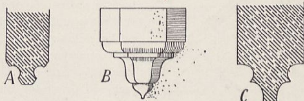
Fig. 117. Mogiła. Szczegóły architektoniczne z klasztoru. A okroj żebra, B konsola z krużganku; C okroj żebra kaplicy i pietra.
