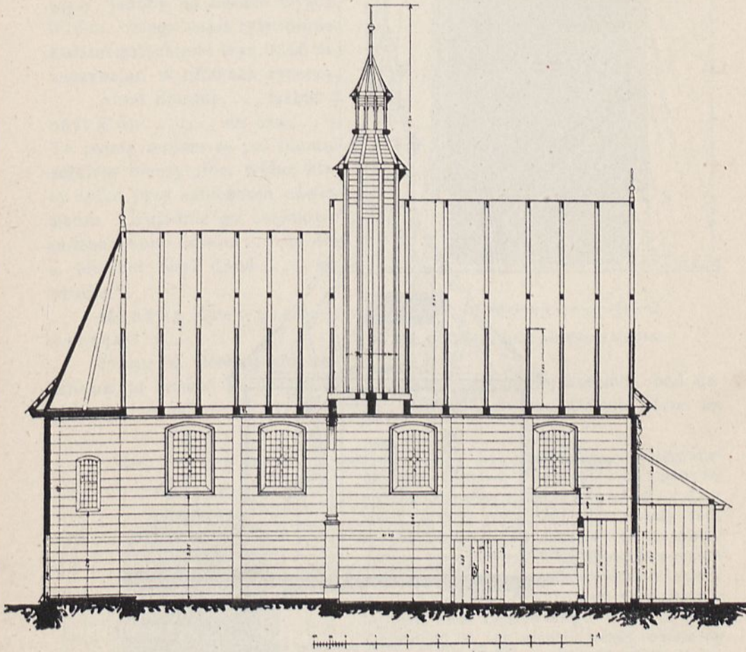
Fig. 59. Czulice. Przekrój podłużny kościoła.
