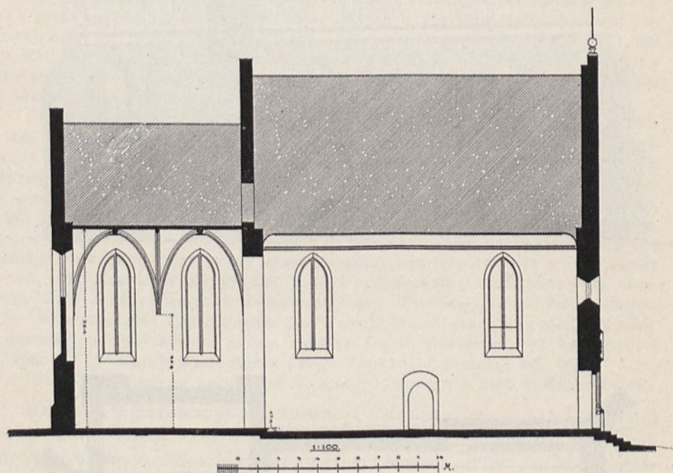
Fig. 144. Raciborowice. Przekrój podłużny kościoła.
