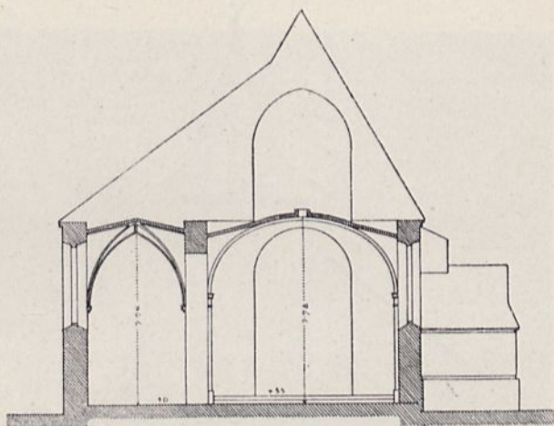
Fig. 159. Ruszcza. Przekrój poprzeczny przez nawy kościoła.
