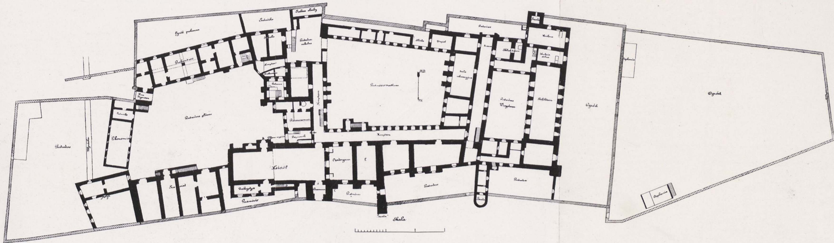
Tabl. XI. Zwierzyniec. Rzut poziomy przyziemia klasztoru Zwierzynieckiego z kościołem, zabudowaniami gospodarskimi i ogrodem.
