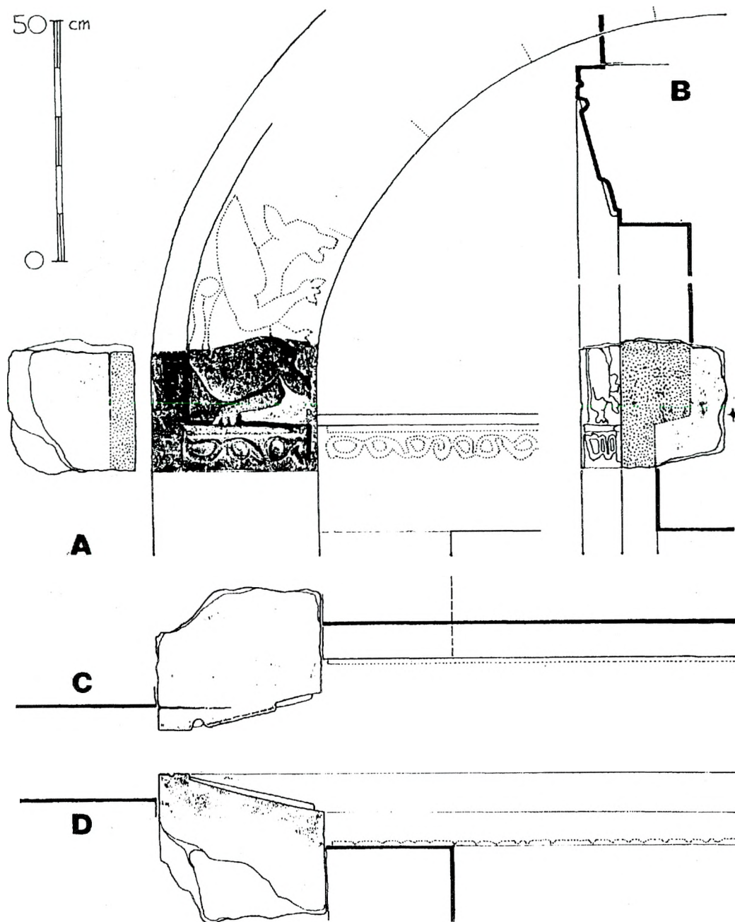
Ryc. 14. Katedra wrocławska. Studium rekonstrukcji form portalu, na podstawie śladów na zachowanej nasadzie archiwolty: A i B – widoki boczne, C – z góry, D – z dołu (oprac. E. Małachowicz)
