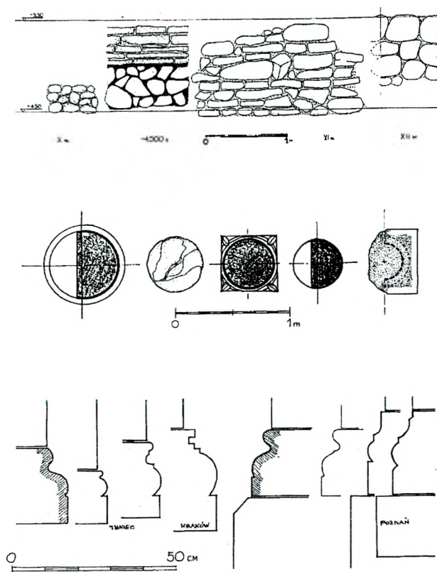
Ryc. 4. Katedra wrocławska. Wątki murów, fragmenty kolumn oraz profile baz i cokołów z XI w. (wrocławskie zakreskowane) (oprac. E. Małachowicz)
