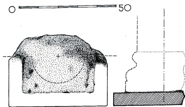
Ryc. 6. Katedra wrocławska. Płyta z odciskiem bazy przyściennej krypty z poł. XI w. (oprac. E. Małachowicz)
