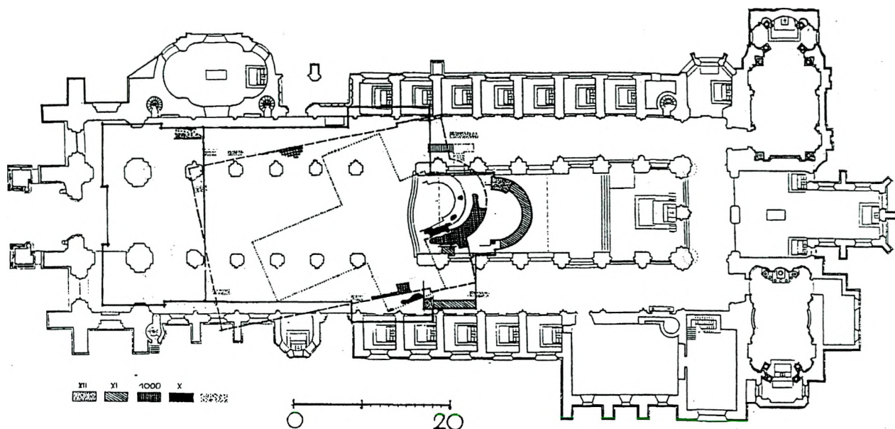
Ryc. 1. Katedra wrocławska. Plan z oznaczeniem zarysów kolejnych budowli z XII, XI, pocz. XI i X w. oraz śladów badań sonarowych (oprac. E. Małachowicz)
