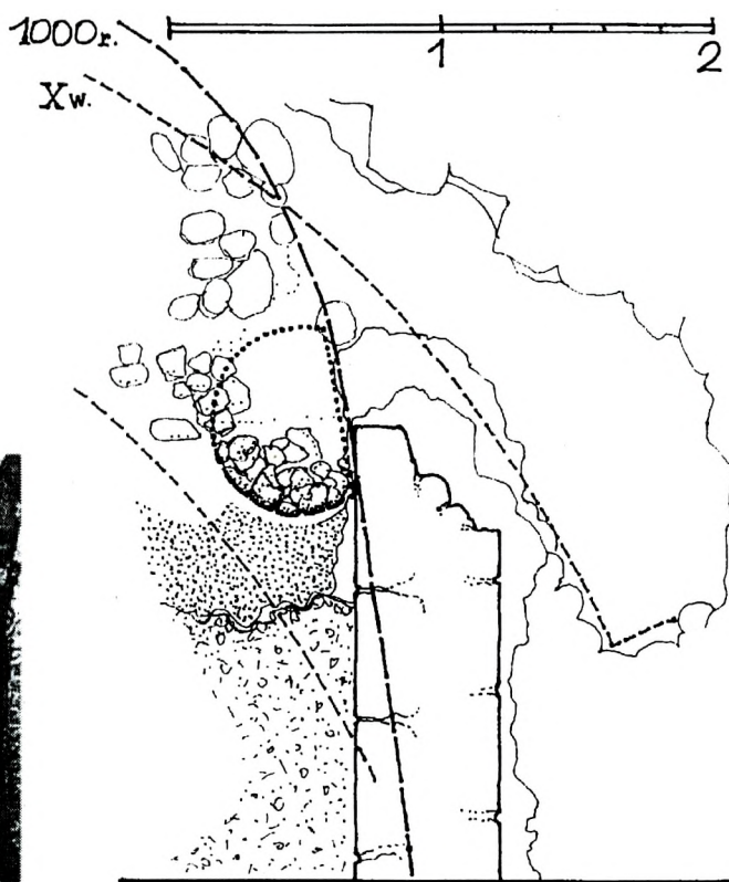
Ryc. 12. Katedra wrocławska. Szkic fragmentu relikwów krypty pierwszej katedry z fundamentem bazy przyścienniej i resztką warstwy posadzkowej oraz widokiem późniejszej nicco krypty w Brevnowie
