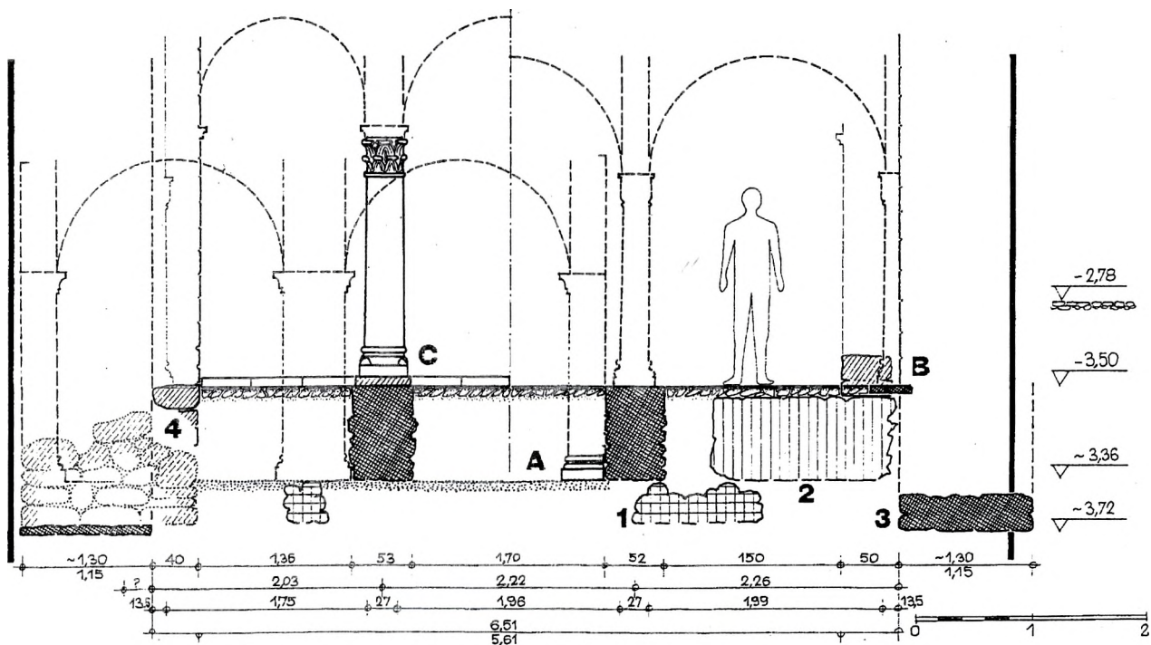
Ryc. 3. Katedra wrocławska. Przekrój podziemia ze schematem usytuowania pionowych odkrytych relikwów: 1 – X w.; 2 – pocz. XI w.; 3 – 2 poł. XI w.; 3 – XII w. oraz rekonstrukcje przekrojów trzech kolejnych krypt: A – pocz. XI w.; B – 2 poł. XI w.; C – XII w. z oznaczeniem zachowanych relikwów (oprac. E. Małachowicz)
