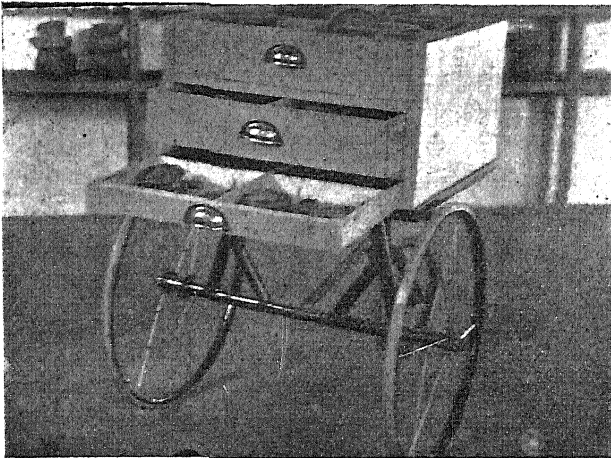
Rys. 5. Skrzynka z rozebranymi wodomierzami na podwoziu.
