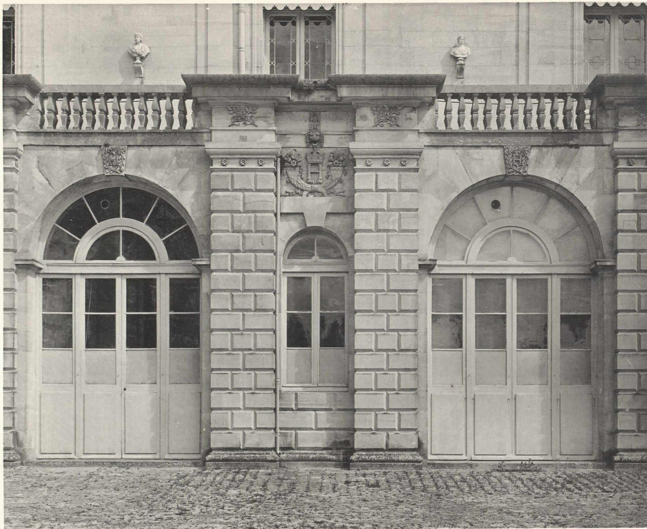
PALAIS DE FONTAINEBLEAU COUR DES FONTAINES, FAÇADE DE LA GALERIE DE FRANÇOIS I ER .
