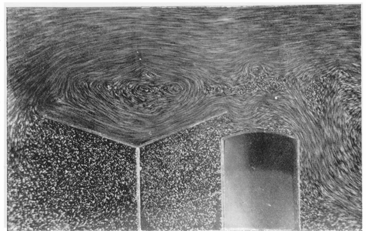
Fot. 6. Napór wiatru na halę dworcową przy obecności wagonu po stronie zawietrznej.
