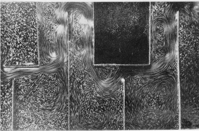
Fot. 7. Przeptyw cieczy przez uszczelnienie labiryntowe.
