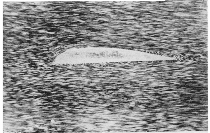
Fot. 10. Optyw profilu lotniczego t. zw. „zdrowy“ (bez oderwania).
