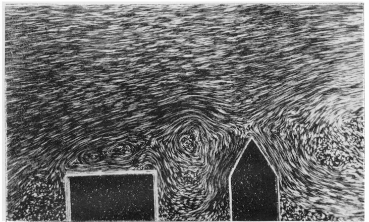
Fot. 5. Wpływ sąsiedztwa dwu budynków na opływ powietrza.
