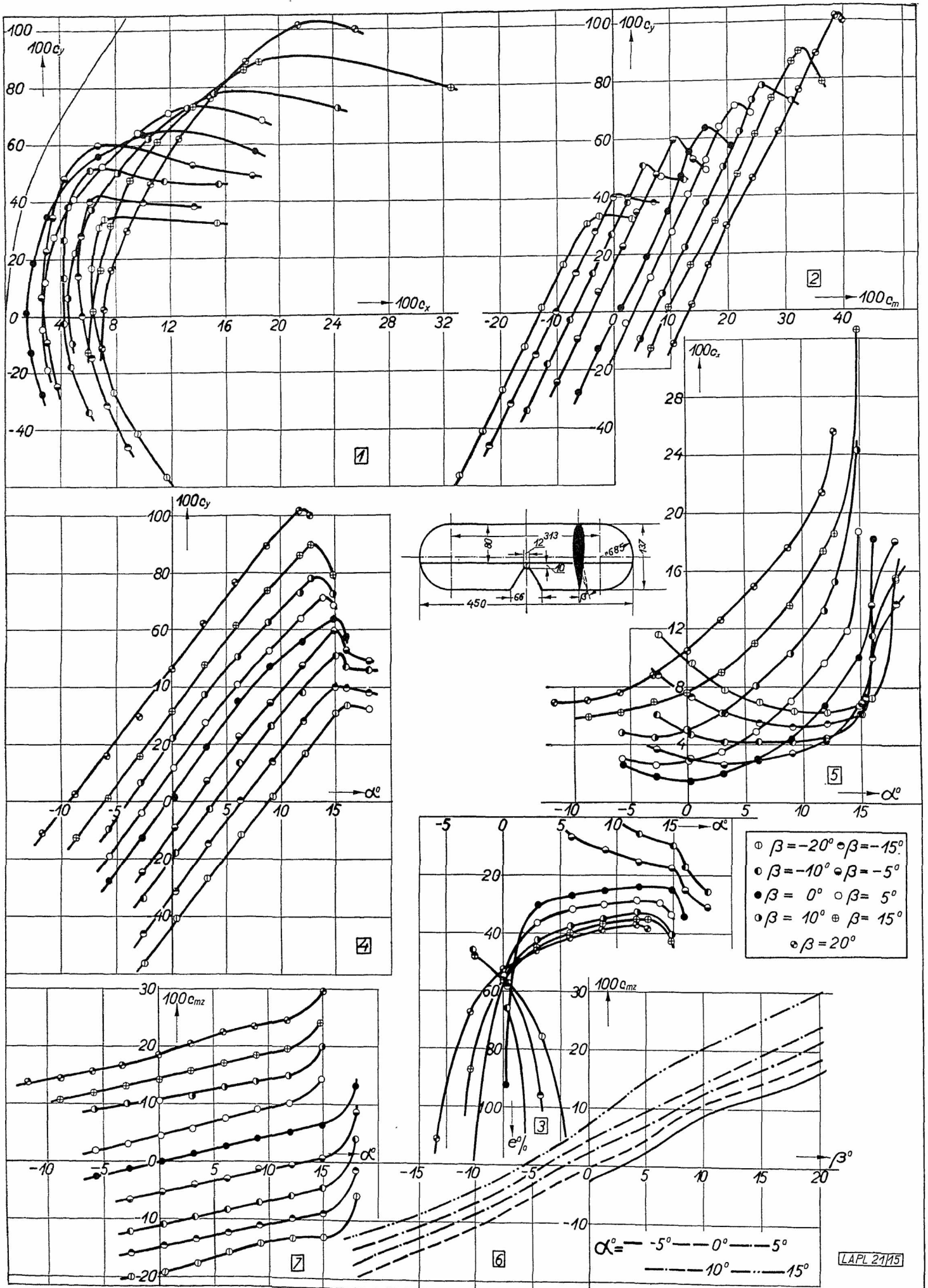
Ryc. 3. Wykresy dla usterzenia poziomego o profilu G 409 o obrysie prostokątnym zaokrąglonym.
