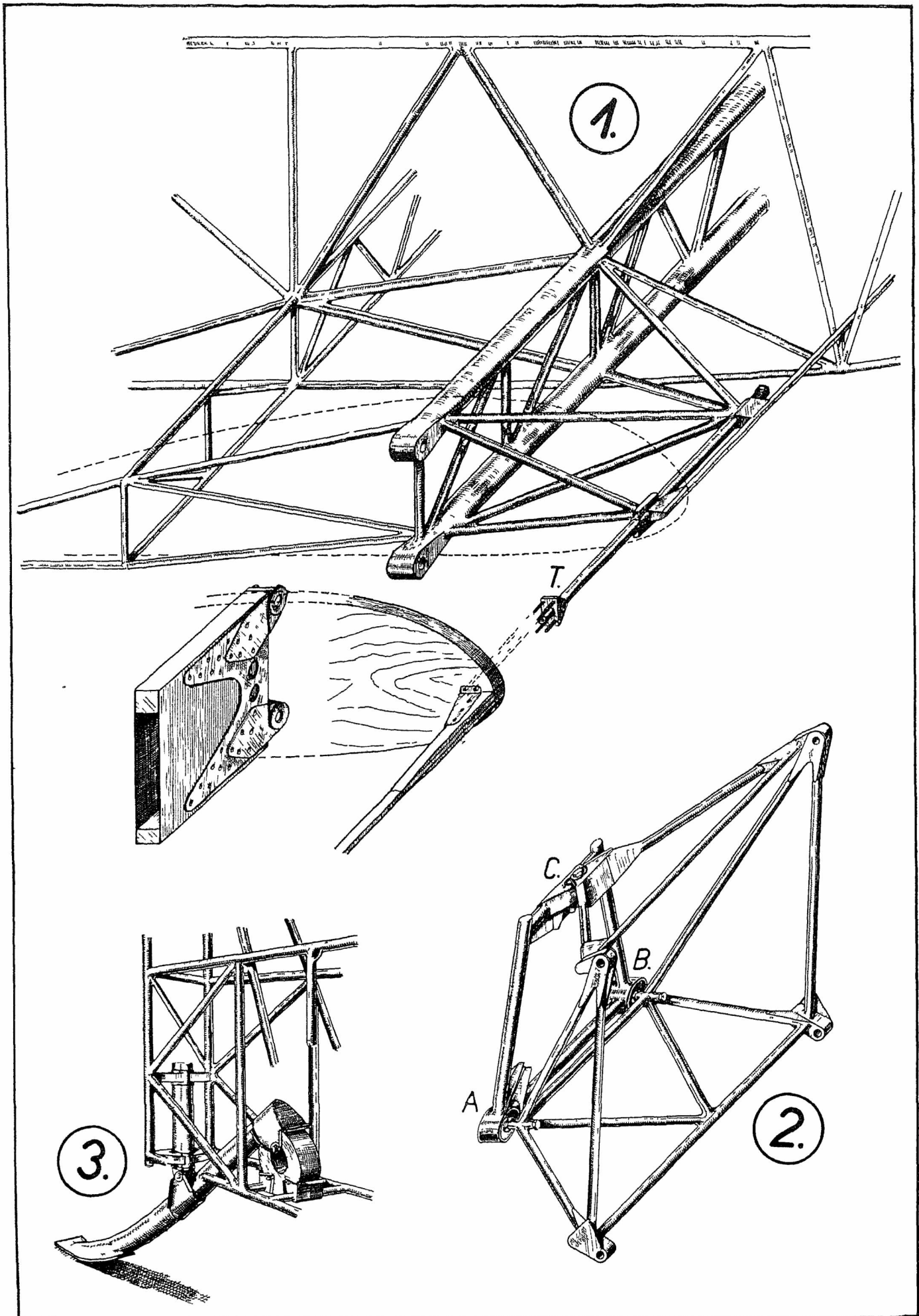
Ryc 8 Niektóre szczegóły konstrukcyjne samolotu N4-4 bis 1 Centralne więzanie kadłuba i połączenie wolnonośnego, jedno-dźwigarowego płata z kadłubem 2 Łoże silnikowe. 3 Płozą ogonową.
