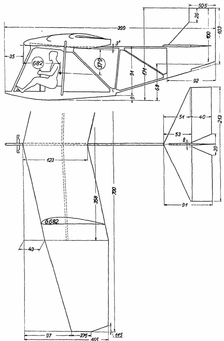
Ryc. 1. Model szybowca szkolnego CW VIII.
