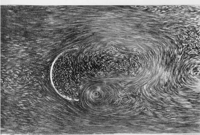
Fot. 8. Optyw półwalca zwróconego stroną wypukłą do płynącej strugi
