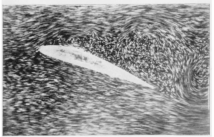
Fot. 11. Optyw profilu lotniczego z oderwaniem z powodu zbyt dużego kąta natarcia.
