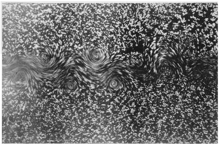
Fot. 12. Droga wirowa Kármán'a.
