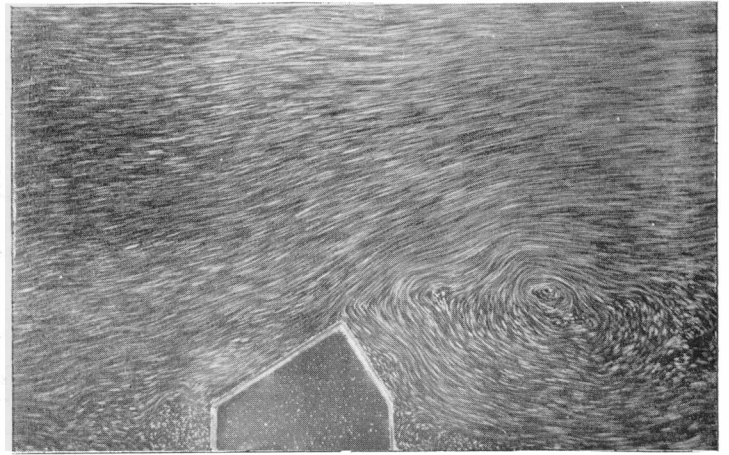
Fot. 4. Napór wiatru na budynek wolnostojący.
