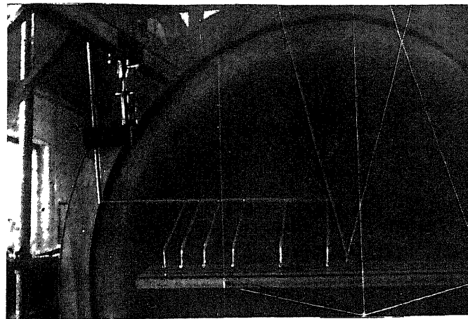
Fot. 2. Zawieszane sondy wielokrotnej w tunelu aerodynamicznym dla pomiaru rozkładu ciśnień wzdłuż płata.
