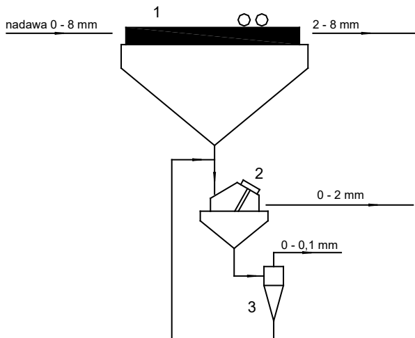
Rys. 2. Schemat płukania kruszyw łamanych
