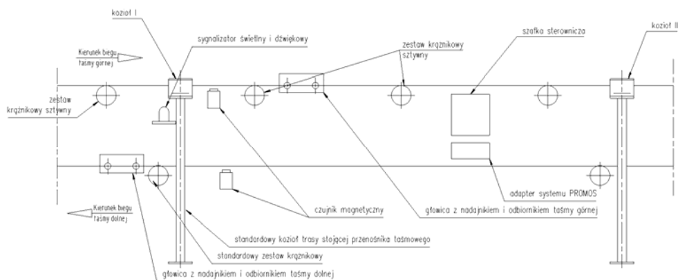
Rys. 3. Schemat bramki kontrolnej
