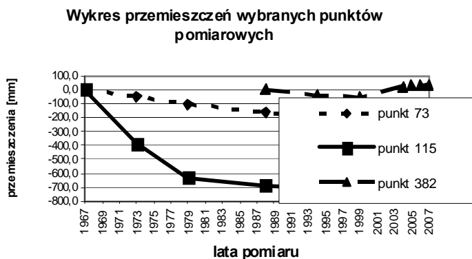
Rys. 6. Wykres przedstawiający zmiany położenia punktów w latach 1967–2007 Fig. 6. Graph of points deformation in years 1967–2007
