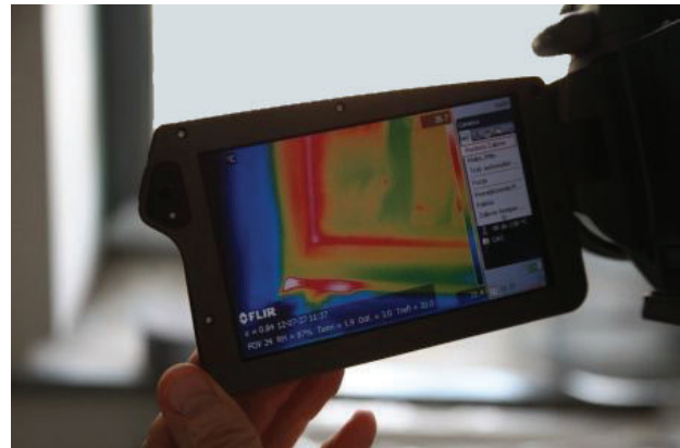
Il. 7. Monitorowanie przecieków przy użyciu kamery termowizyjnej Fig. 7. Monitoring leakages with the use of a thermal imaging camera
