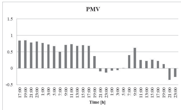
Il. 10. Wskaźnik PMV – użytkownicy odpoczywający
