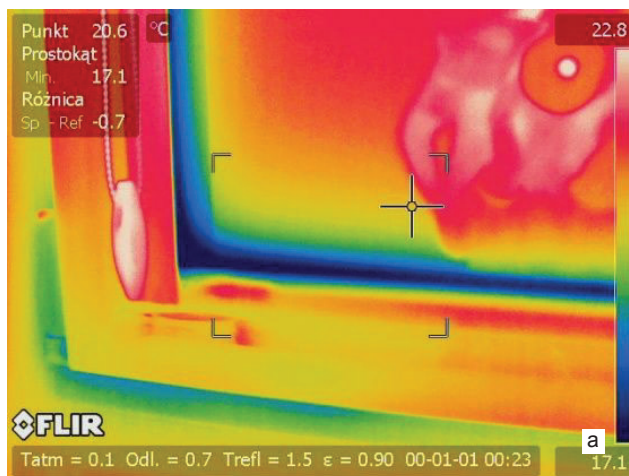
II. 3. Skroplona wilgoć w połączeniu układu szybowego z ramą: a) termogram oraz b) zdjęcie rzeczywiste
