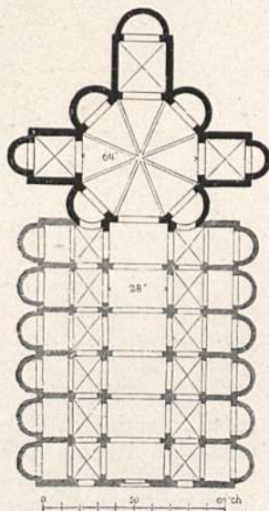
Abb. 116. S. Maria della Passione zu Mailand.
