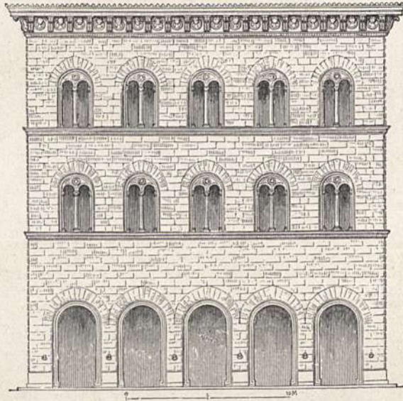
Abb. 26. Pal. Spannocchi zu Siena.
