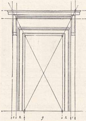
Abb. 73. Türumrahmung. (Nach A. Thiersch.)
