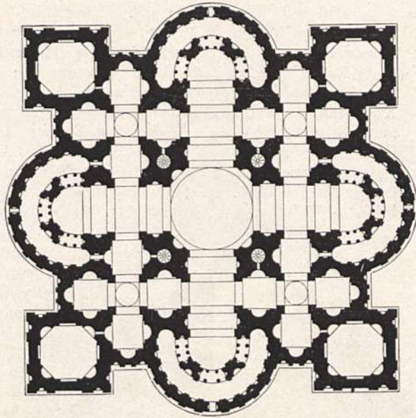
Abb. 105. St. Peter. Peruzzis Grundriß.
