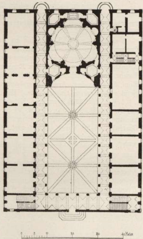
Abb. 186. Sapienza zu Rom. Grundriß. (Nach Gurlitt.)
