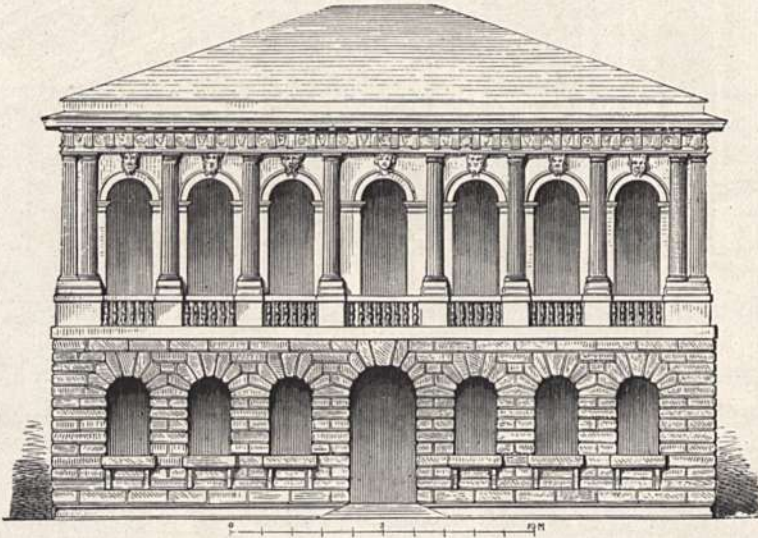
Abb. 203. Pal. Pompei zu Verona.
