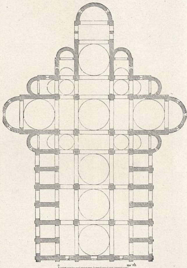
Abb. 165. S. Giustina zu Padua. (L.)
