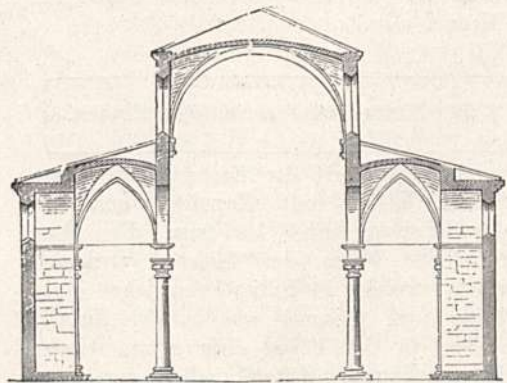
Abb. 143. Servi zu Siena. Querschnitt. (L.)
