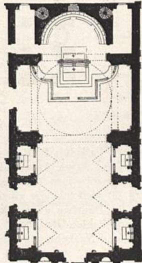
Abb. 155. S. Maria de' Monti. (Nach Letarouilly.)
