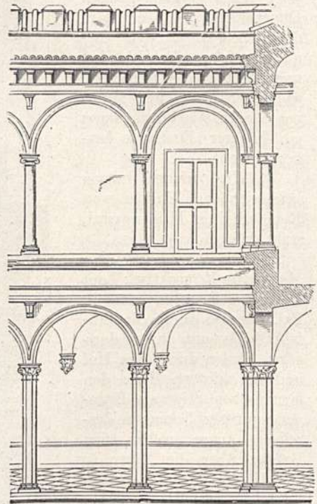
Abb. 213. Ehemaliger kleiner Pal. di Venezia zu Rom. Hof. (Nohl.)
