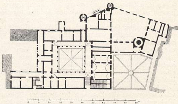
Abb. 197. Palazzo ducale zu Urbino. Grundriß.
