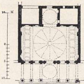
Abb. 87. Capp. Pazzi zu Florenz. Grundriß. (Nach Paulus.)
