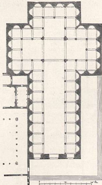
Abb. 140. S. Spirito zu Florenz. Grundriß.
