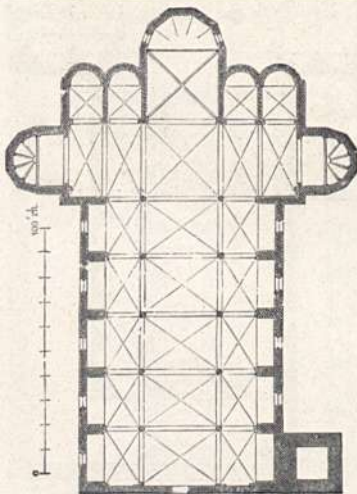
Abb. 142. Servi zu Siena. Grundriß. (L.)
