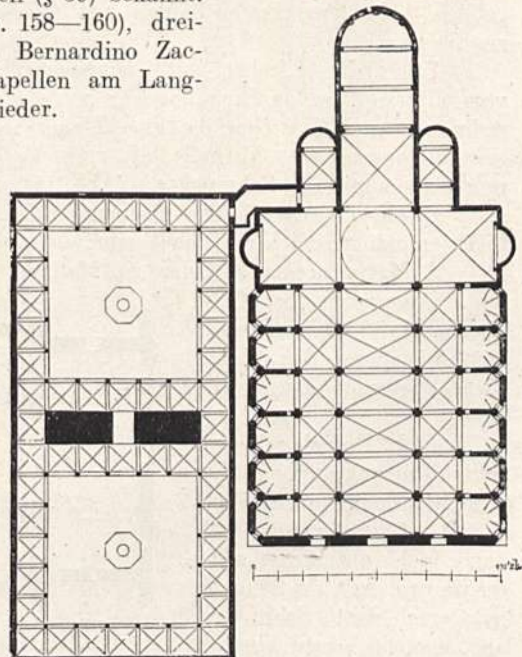
Abb. 158. S. Giovanni zu Parma. (L.)
