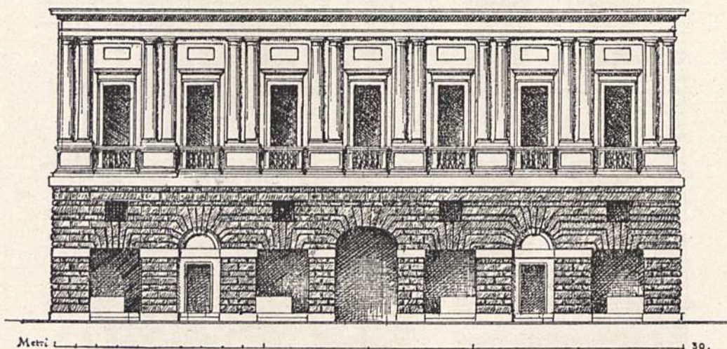
Abb. 208. Pal. Vidoni-Caffarelli zu Rom. (Nach Geymüller.)
