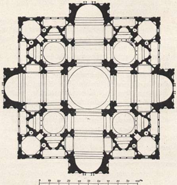
Abb. 104. St. Peter. Bramantes erster Grundriß.
