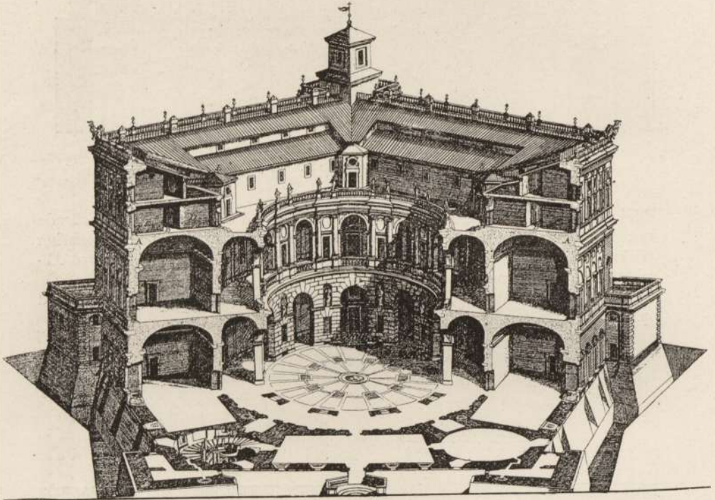
Abb. 259. Schloß Caprarola. (Nach Gurlitt.)
