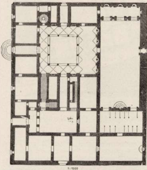
Abb. 192. Pal. Riccardi zu Florenz. Grundriß.
