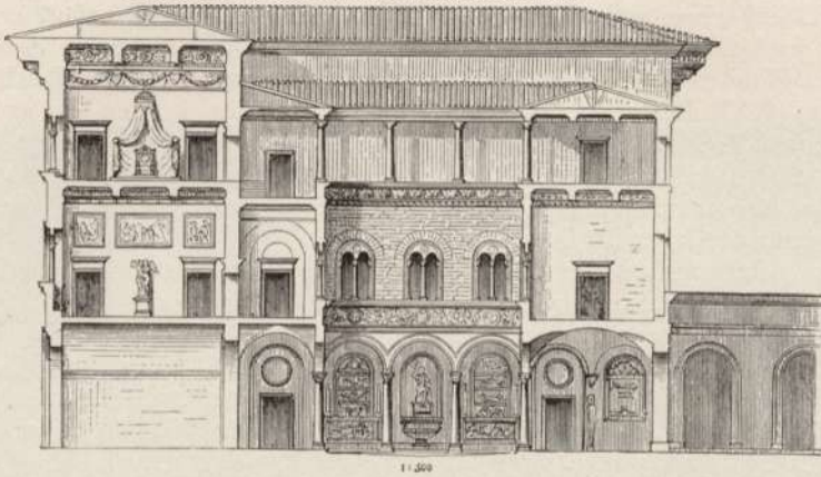
Abb. 191. Pal. Riccardi zu Florenz. Durchschnitt.
