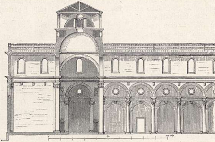
Abb. 137. S. Lorenzo zu Florenz. Längenschnitt.
