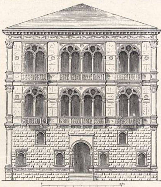
Abb. 39. Pal. Corner-Spinelli zu Venedig.
