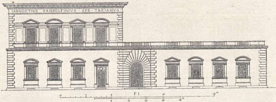
Abb. 204. Pal. Pandolfini zu Florenz. (Nach Bühlmann.)
