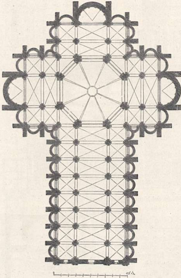
Abb. 156. Dom zu Pavia.
