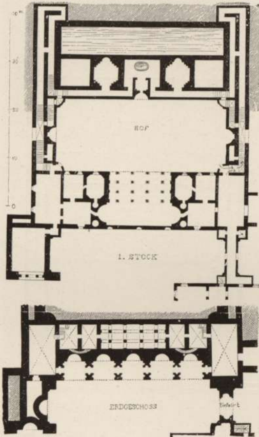
Abb. 256. Monte Imperiale bei Pesaro.
