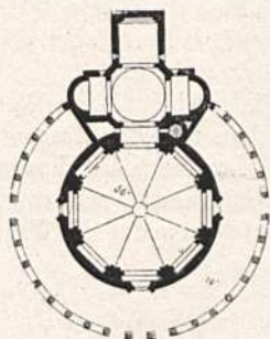
Abb. 114. Madonna di Campagna bei Verona. (L.)
