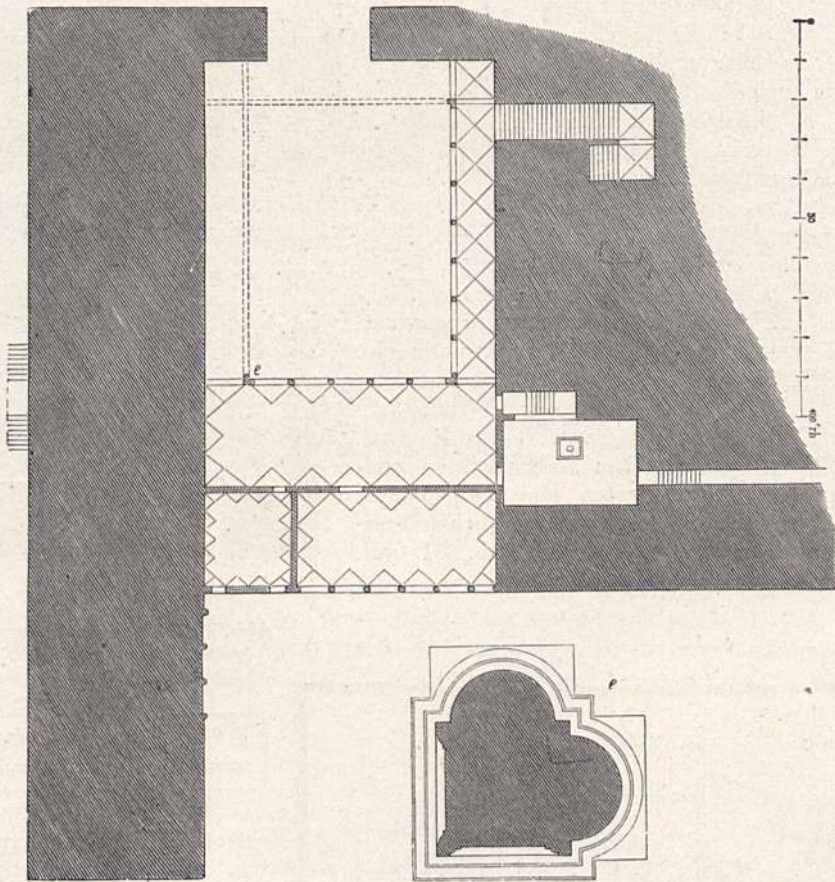
Abb. 201. Pal. Serofa zu Ferrara. (L.)
