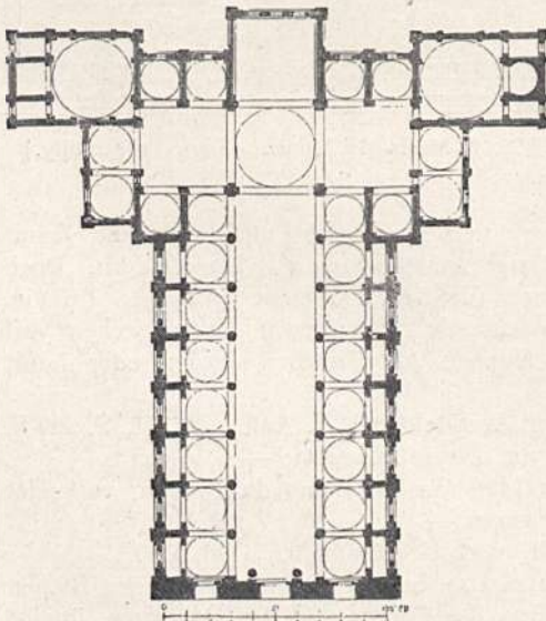
Abb. 138. S. Lorenzo zu Florenz. Grundriß.
