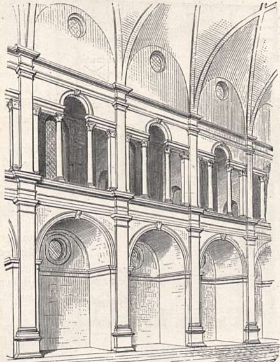
Abb. 150. S. Maurizio (monastero maggiore) zu Mailand. (Lasius.)
