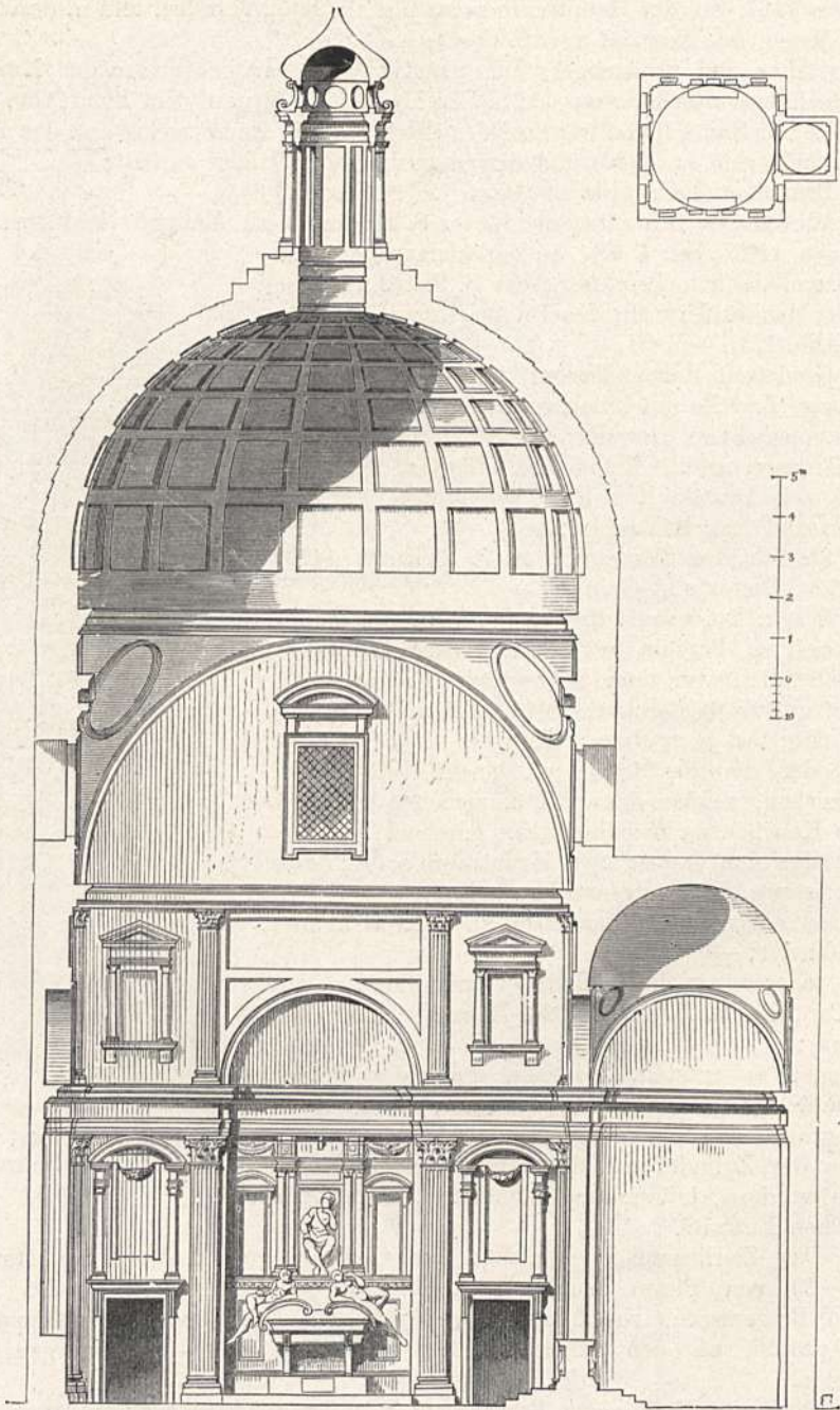
Abb. 178. Mediceische Kapelle an S. Lorenzo zu Florenz.
