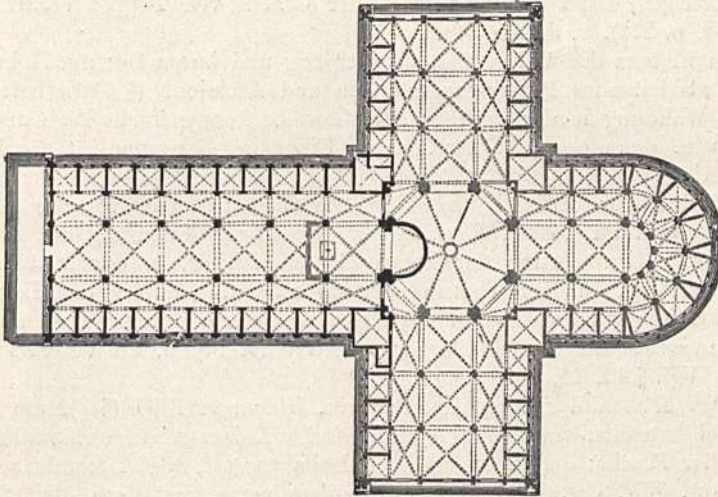
Abb. 9. Grundriß von S. Petronio zu Bologna.
