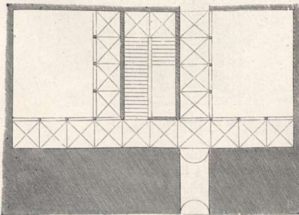
Abb. 200. Pal. Fantuzzi zu Bologna. (L.) Burekhardt, Italien. Renaissance. 6. Aufl.
