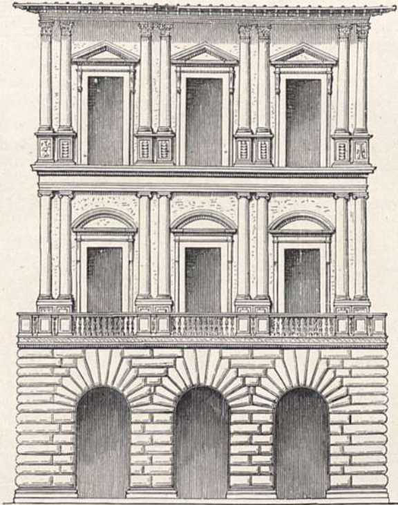
Abb. 58. Pal. Uguccioni zu Florenz.
