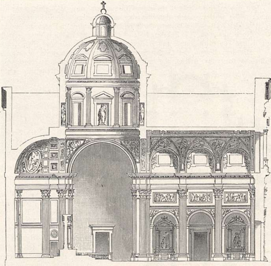
Abb. 154. S. Maria de' Monti. (Nach Letarouilly.)
