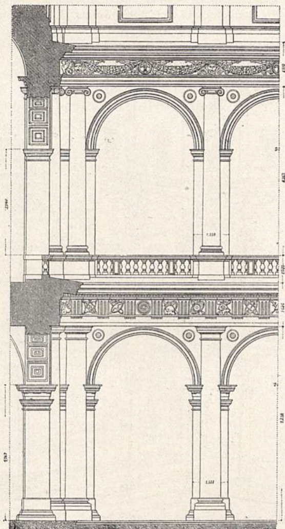
Abb. 211. Pal. Farnese zu Rom. Hofarkaden. (Nach Bühlmann.)
