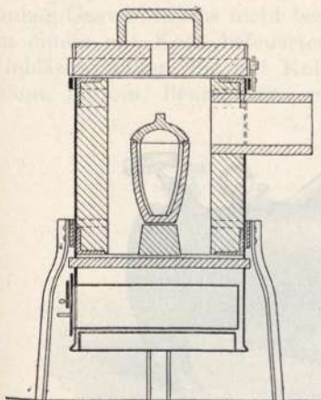
Fig. 74. Kokswindofen der deutschen Scheideanstalt.
