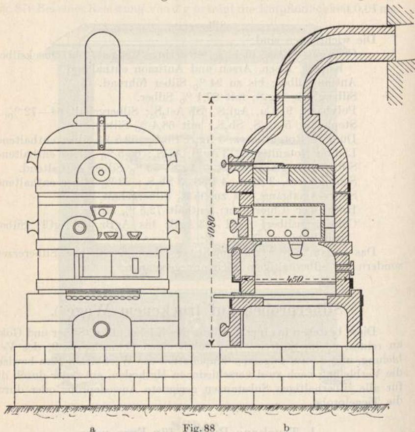
Fig. 88 Transportabler Freiburger Muffelofen für Steinkohlen- und Koksfeuerung von der Kgl. Sächs. Schamottefabrik Muldenhütten b. Freiberg.
