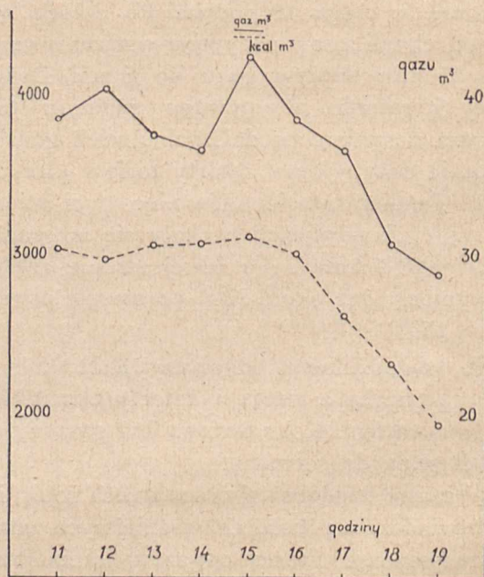
Rys. 4. Wykres ciepła spalania gazu i ilości gazu w poszczególnych okresach odgazowywania.
