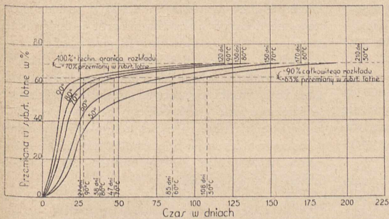
Rys. 6. Wykres przemiany mułu w substancje lotne zależnie od temperatury i czasu fermentacji.
