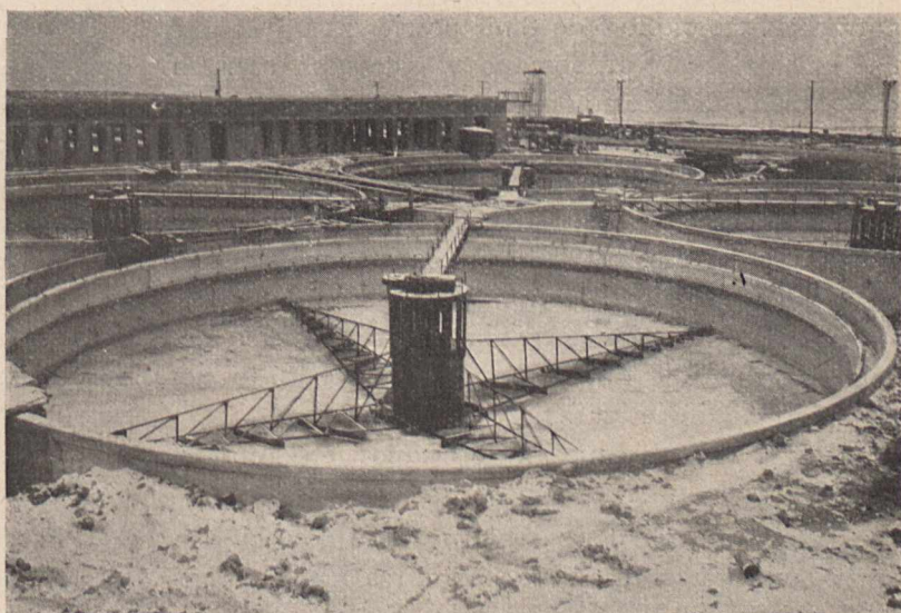
Rys. 3. Oczyszczalnia okrągła systemu Dorr.
