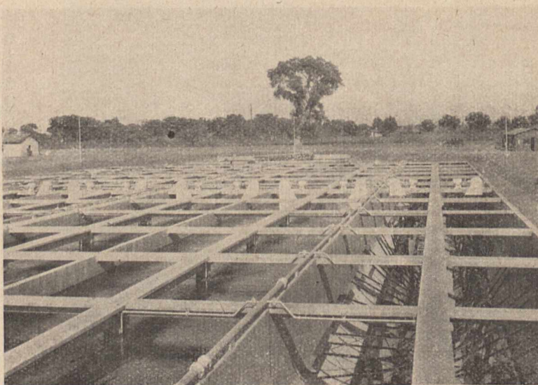
Rys. 4. Komory do napowietrzania systemu Dorrco.
