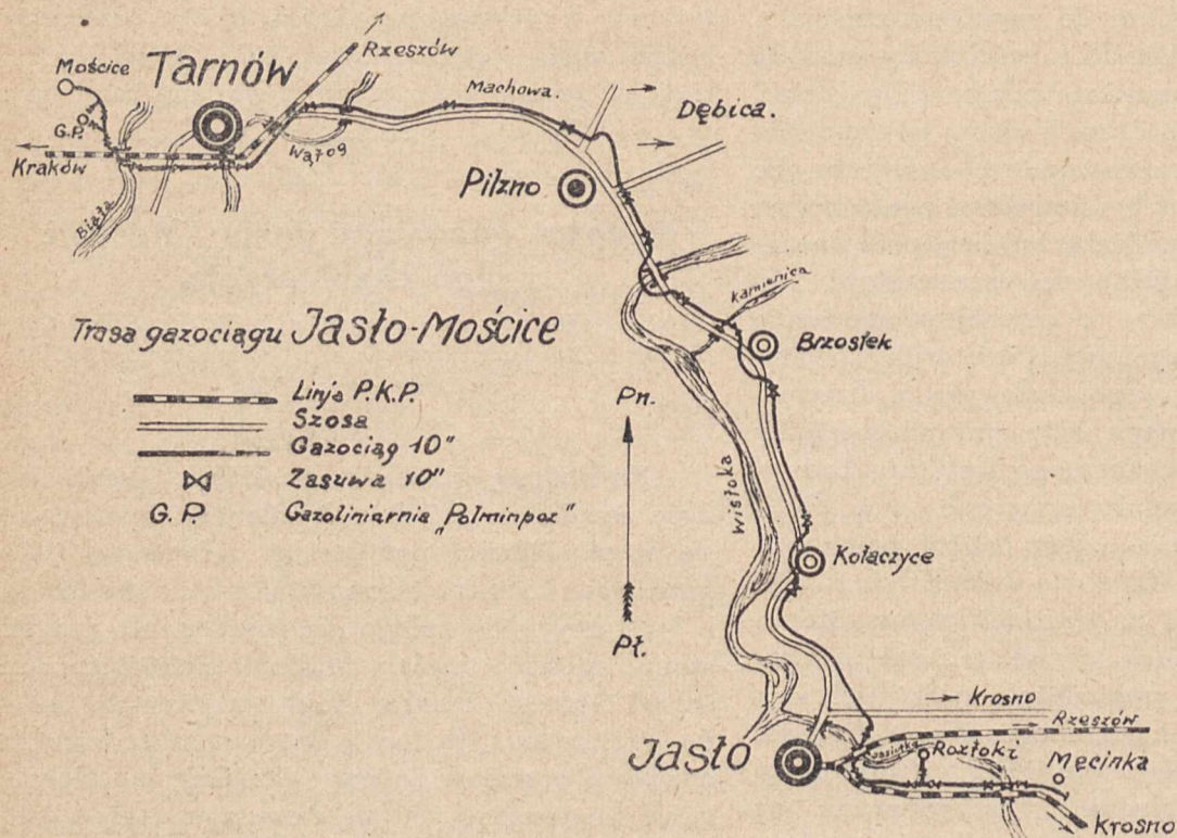
Rys. 1. Trasa gazociągu Jasto-Mościce.
