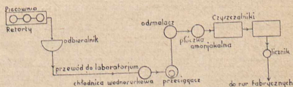
Rys. 1. Schemat procesu odgazowywania torfu i oczyszczania gazu.
