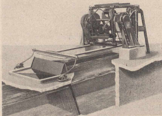
Rys. 1. Kraty Dorcco z automatycznym oczyszczaniem.
