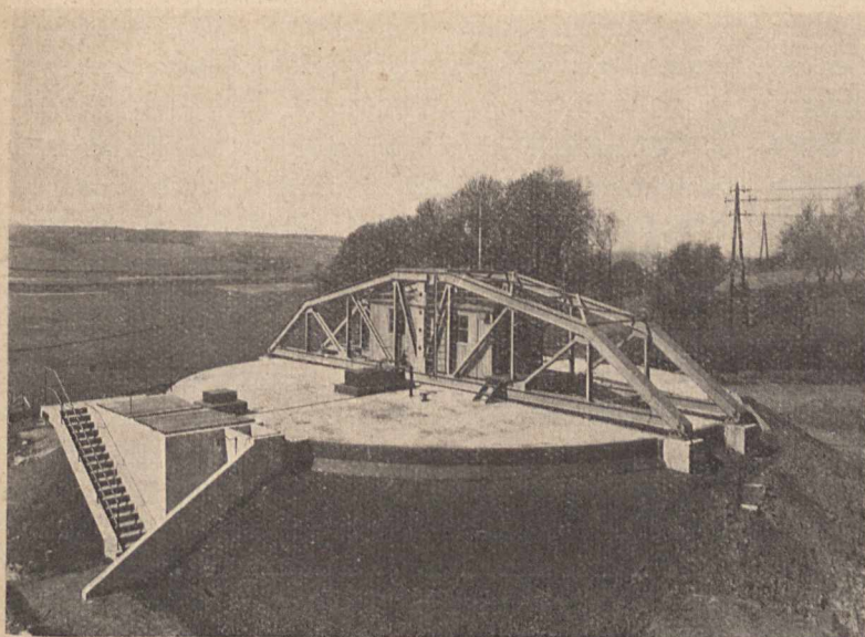
Rys. 5. Komora fermentacyjna.
