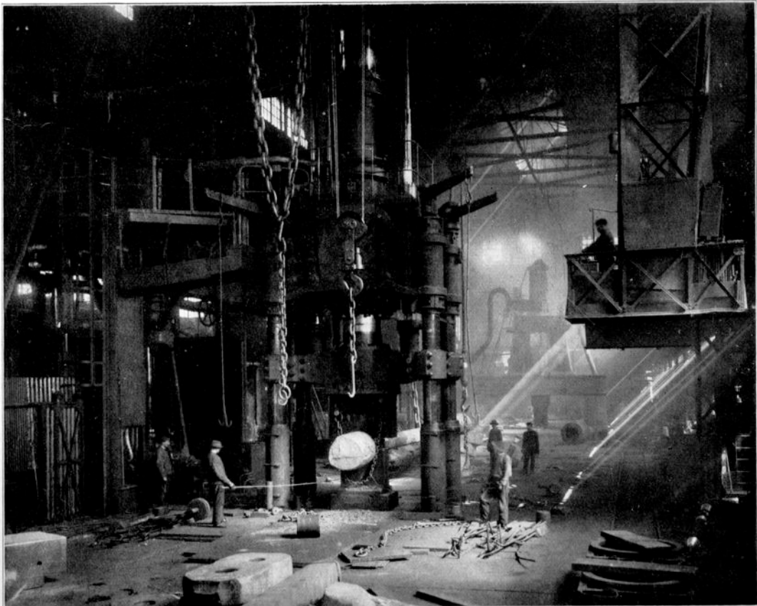
2500 Tons-Schmiedepresse im Borsigwerk O.-S.
