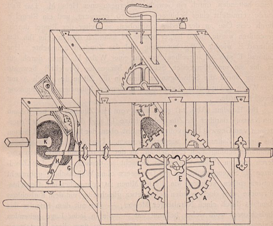
Abb. 78. Die Antwerpener Zünduhr nach Johann von Nassau.
