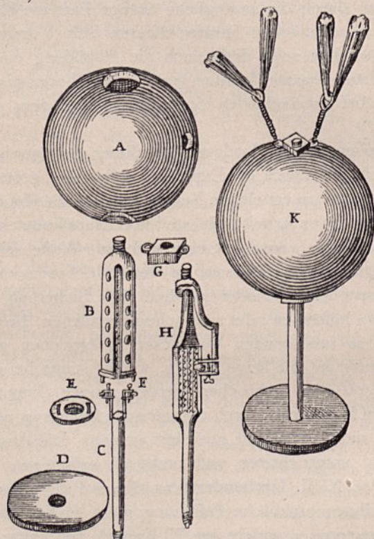
Abb. 86. Handgranaten mit Fallzündung.
