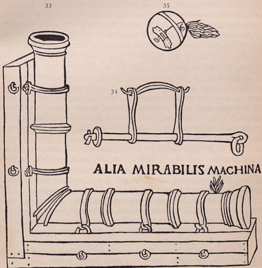
Abb. 33—35. Geschütz und Bombe.
