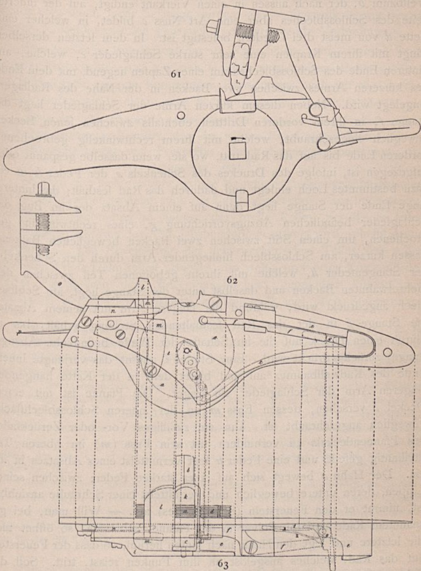
Abb. 61—63. Radschloss.
