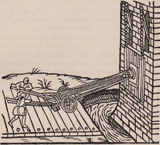
Abb. 88. Spierenpetarde.
