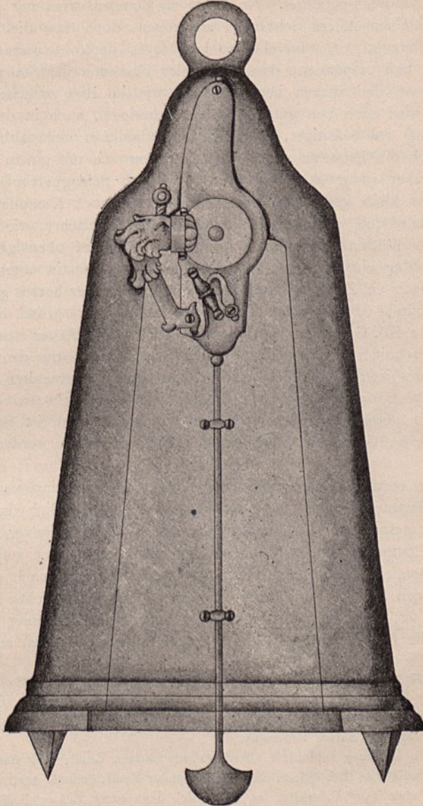
Abb. 87. Fallpetarde mit Fallzündung.
