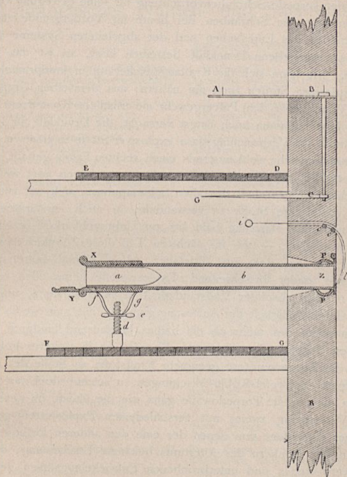
Abb. 92. Raketen-Torpedo nach Montgéry.
