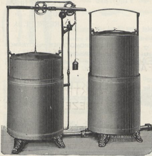
Hydraulisches Gebläse (siehe Seite 132 dieses Buches).
