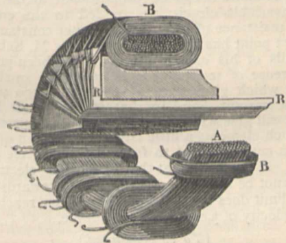
FIG. 6.—Gramme Armature.
