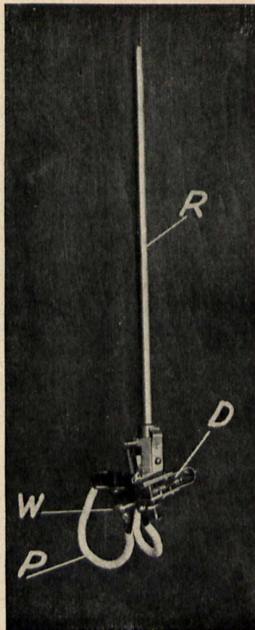
Rys. 31. Samoczynny regulator temperatury warnika (wykonanie krajowe). R—rurka mosiężna wydłużająca się pod wpływem ciepła z umieszczonym wewnątrz niej prętem inwarym, — układ dźwigni, W — wyłącznik rtęciowy przechylny, P — przewody doprowadzające prąd do wyłącznika.
