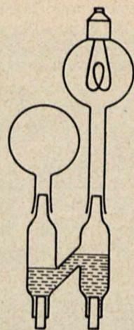
Rys. 32. Wyłącznik rtęciowy sterowany ciśnieniem gazu.
