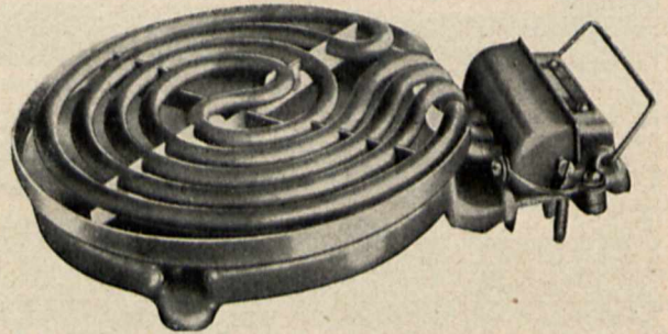
Rys. 19. Kuchenka elektryczna z rurkowym elementem grzejnym (wykonanie zagraniczne) 29 ).
