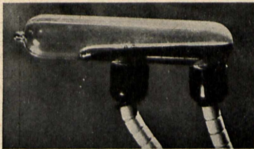
Rys. 29. Wyłącznik rtęciowy przechylny.
