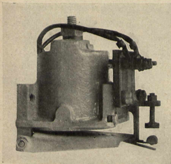
Rys. 22. Przekaznik pozycji.
