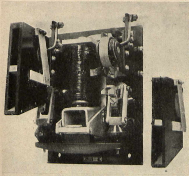
Rys. 19. Kontaktor ogrzewania.
