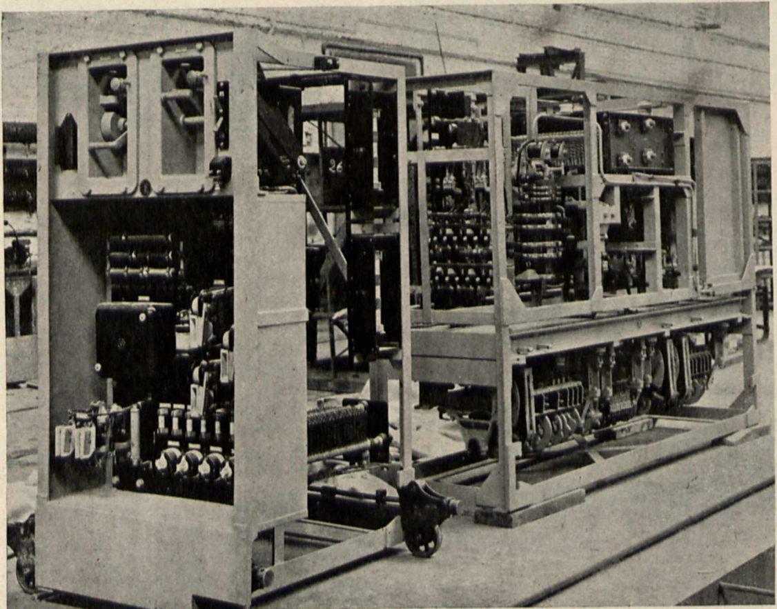
Rys. 24. Zmontowane ramy (główka i pomocnicza) z aparaturą rozrządczą.
