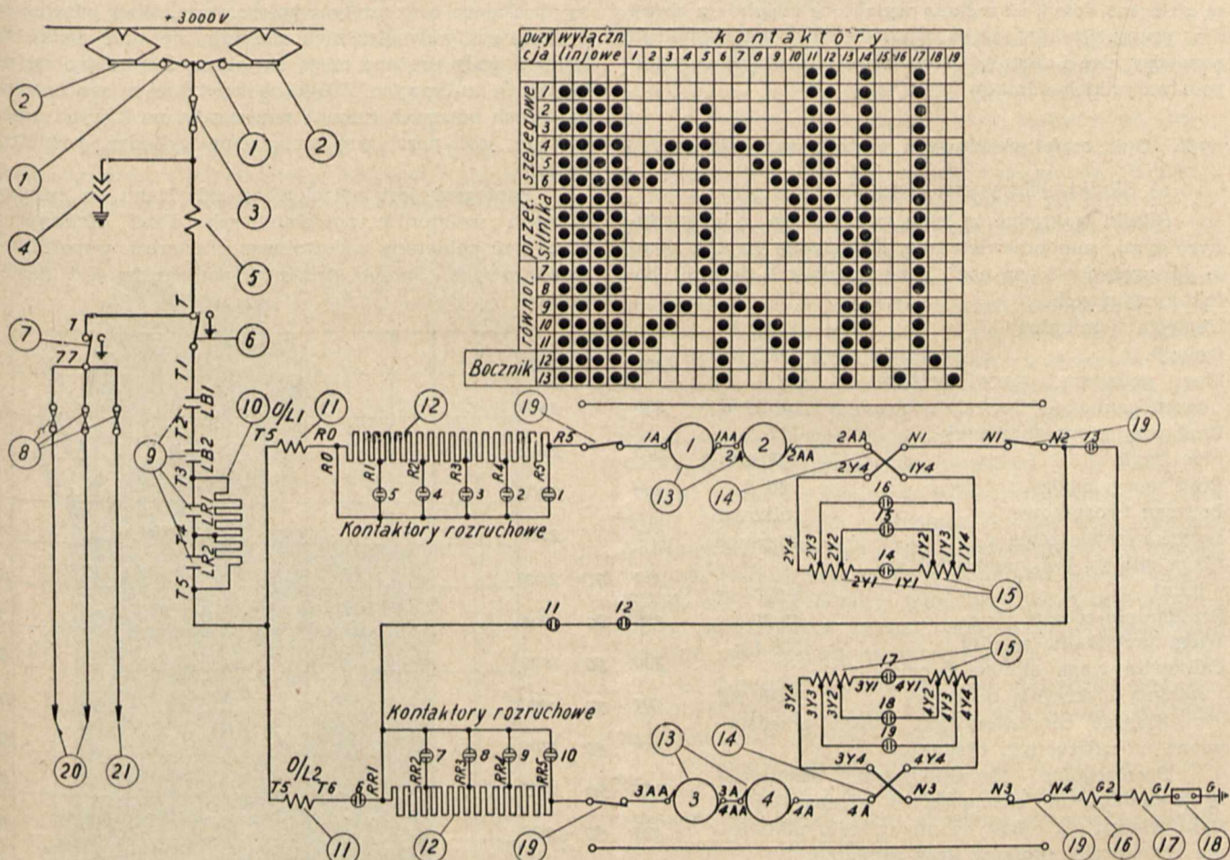
Rys. 2. Obwód zasadniczy.
