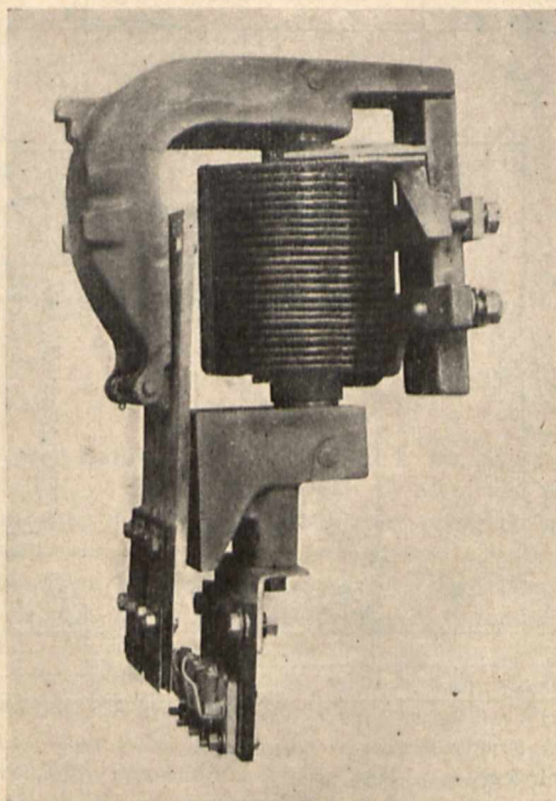
Rys. 9. Przełącznik zanikowy.
