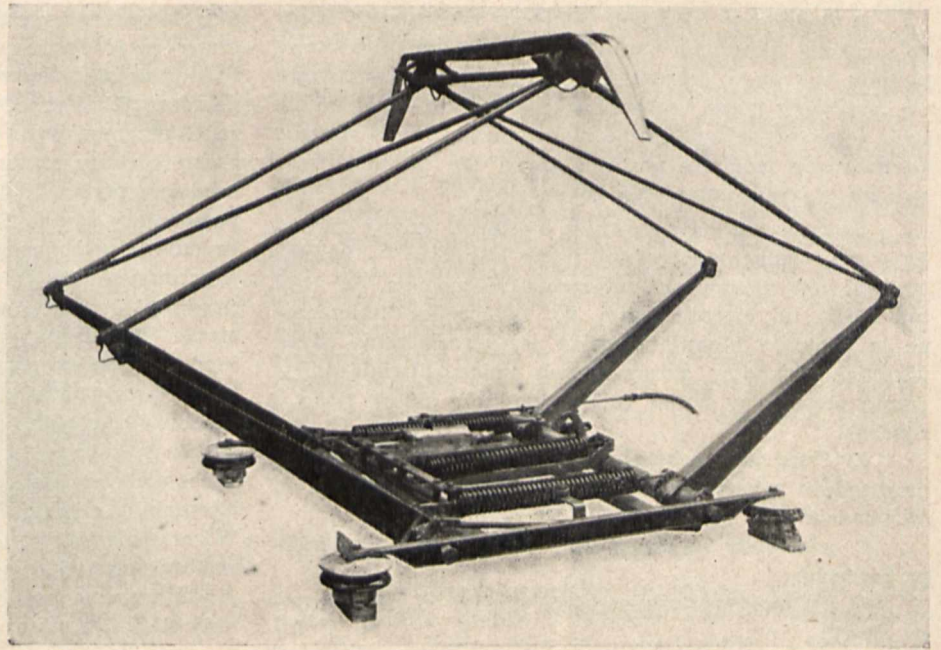
Rys. 5. Pantograf.
