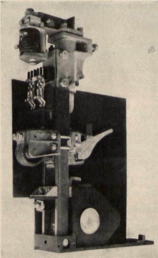
Rys. 6. Wyłącznik liniowy.
