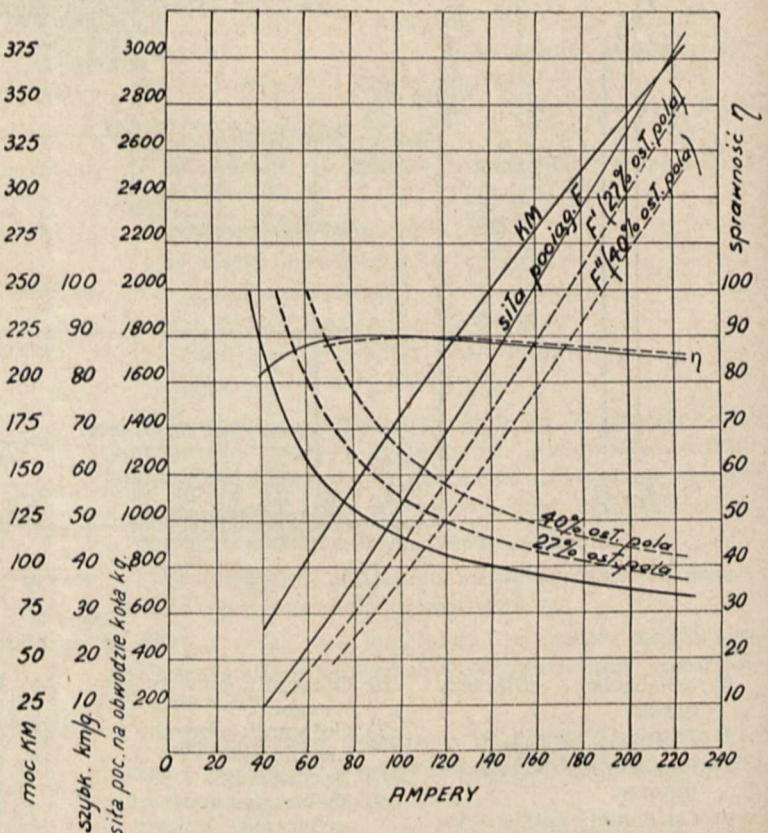
Rys. 4. Charakterystyki silnika trakcyjnego.
