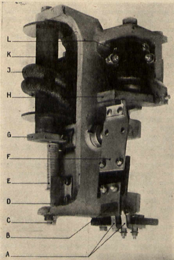
Rys. 7. Przełącznik nadmiarowy.
