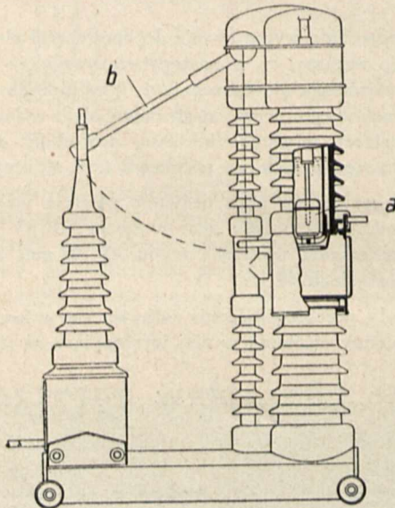
Rys. 6. Wyłącznik strumieniowy R 100, napowietrzny, z odłącznikiem. a) różnicowa komora strumieniowa DAL, b) odłącznik.
