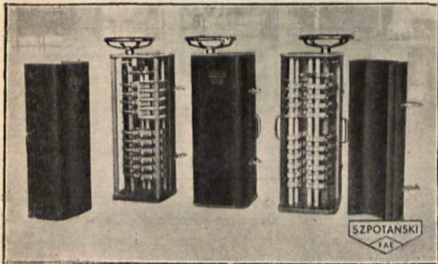
Rys. 1. Nastawniki młoteczkowe typu 937.
