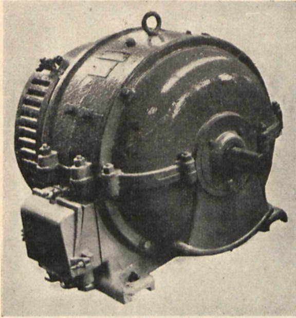
Rys. 2. Maszyna okrętowa o mocy 25 kW, 1 400 obr/min, 120 V.
