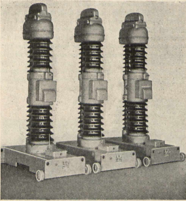
Rys. 5. Wyłącznik strumieniowy R 60, 600 A.
