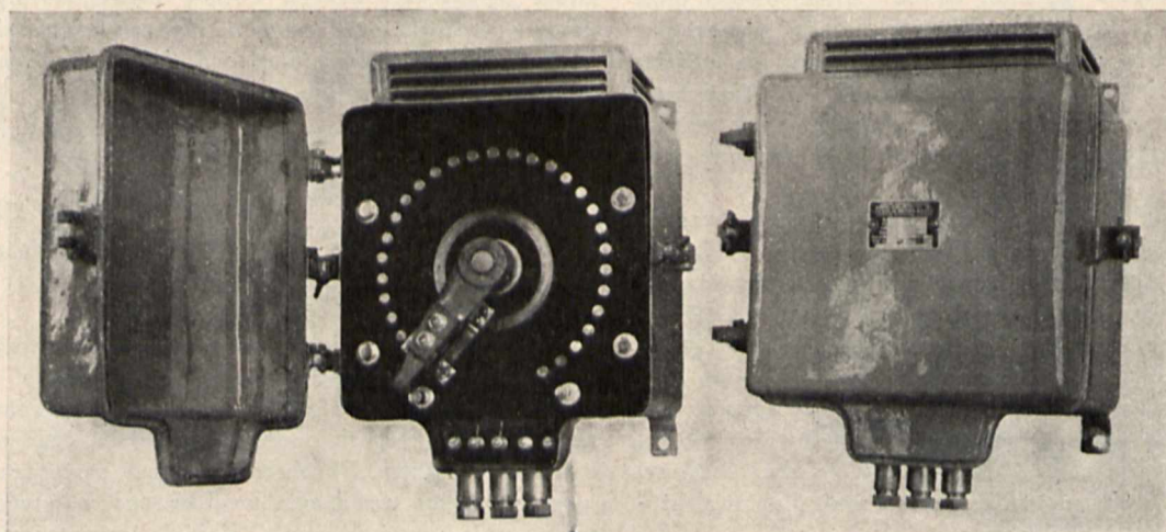
Rys. 1. Regulatory bocznikowe do maszyn okrętowych o mocy 25 kW.
