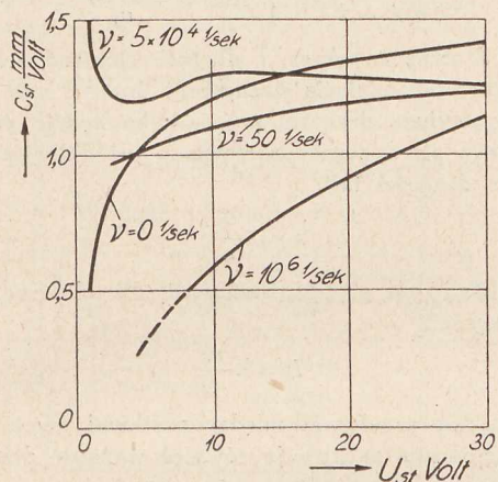
Rys. 9. Zmiany czułości z frekwencją w osc. kat. firmy AEG. wdg. Heimanna.
