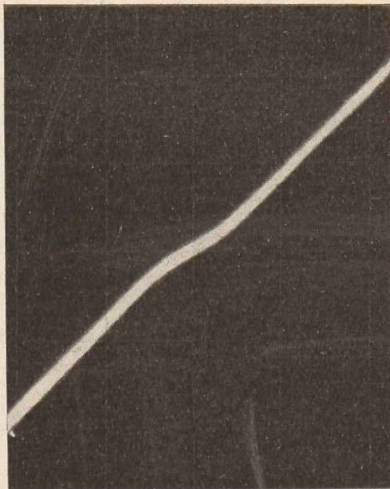
Rys. 7. y = f(U_{st}) jednego ze starszych wykonań oscylografu o napięciu anodowym Ea = 3000 \text{ V} . Według M. v. Ardenne.
