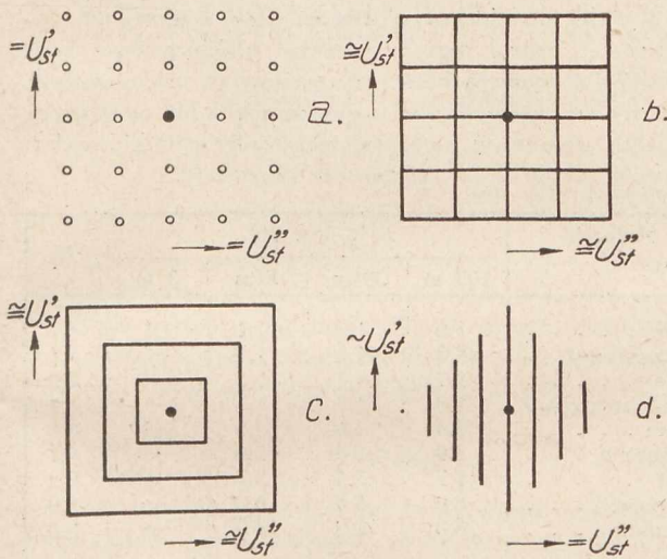
Rys. 21. E_a = 350 \text{ V}; \Delta U_{st} = 8 \text{ V}.
