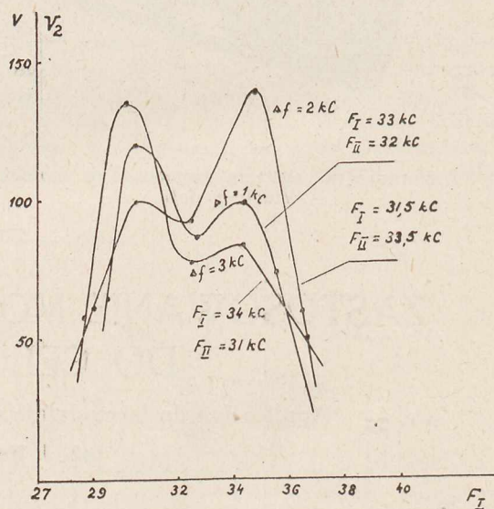
Charakterystyki filtru I
