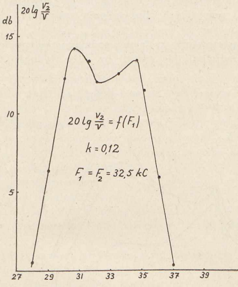
Definitywna charakterystyka filtra I
