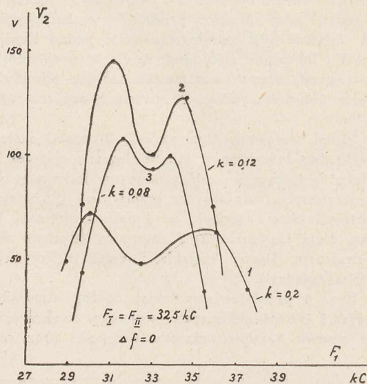
Charakterystyki filtru I
