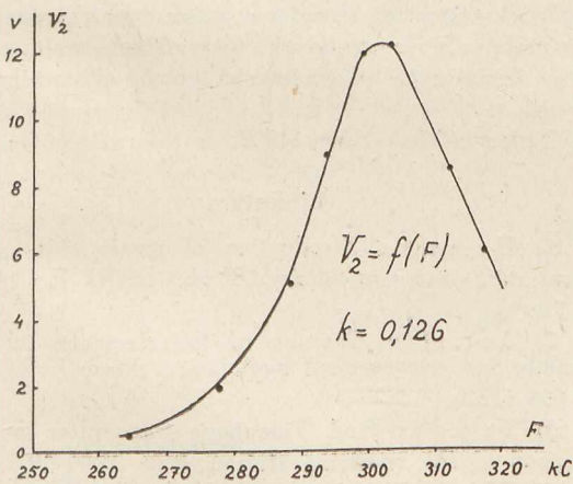
Charakterystyka filtra II
