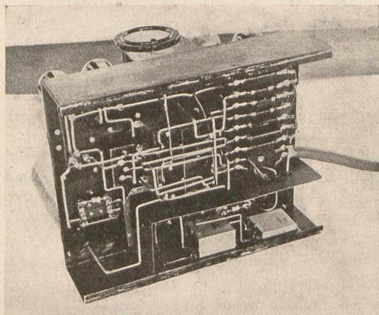
Rys. 6. Atmoradjo graf systemu Lugeon. Typ morski. Widok z dołu.
