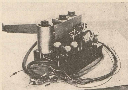
Rys. 5. Atmoradjo graf systemu Lugeon. Typ morski.
