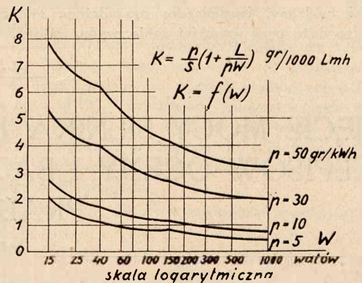
Rys. 12. Zależność kosztu światła (k) od wielkości żarówki (W) przy różnych cenach prądu elektrycznego.
