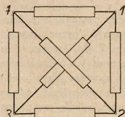
Rys. 9. Wielokąt zupełny o 4 złączach ( z=4 ).
