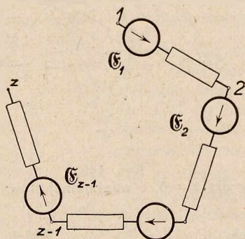
Rys. 13. Drugi sposób włączania w T stransfigurowanych SEM-cznych.
