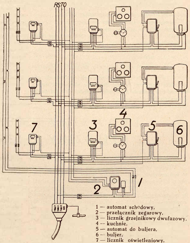
Rys. 5. Schemat instalacji liczników.
