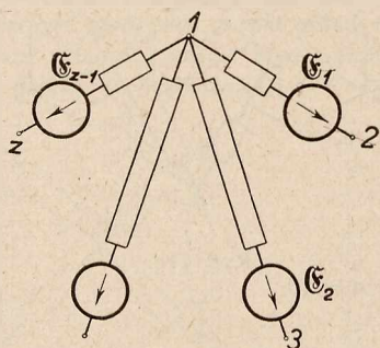
Rys. 12. Pierwszy sposób włączania w T stransfigurowanych SEM-cznych.
