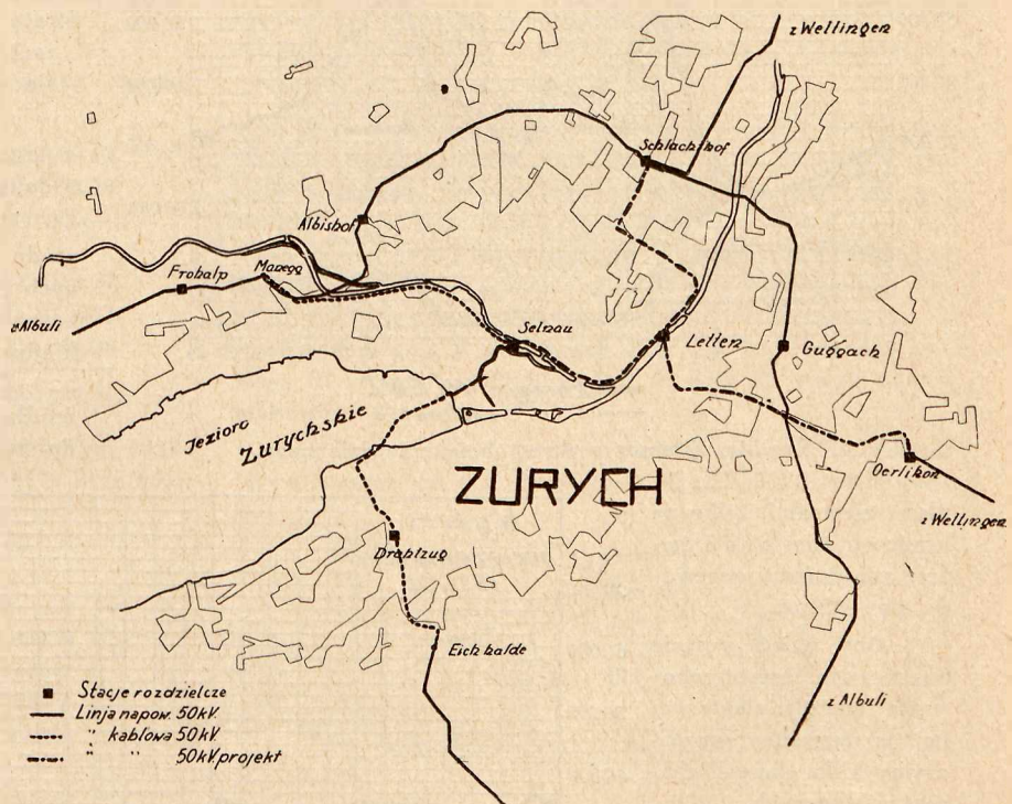
Rys. 3. Dyspozycja okružnej sieci powietrznej i sieci kablowej 50 kV.
