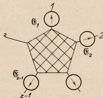
Rys. 14. Trzeci sposób włączania w T stransfigurowanych SEM-cznych.
