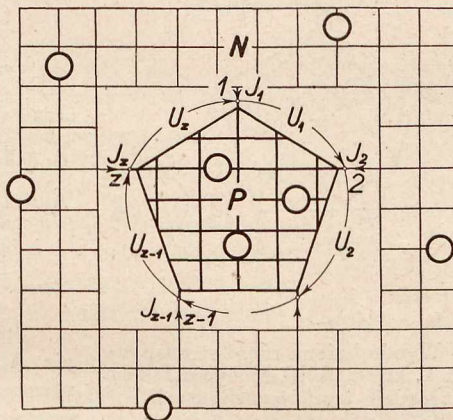
Rys. 1. Obwód pierwotny
