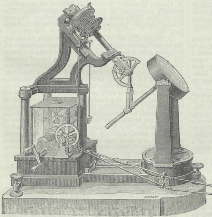
FIG. 1.—The Siderostat.
