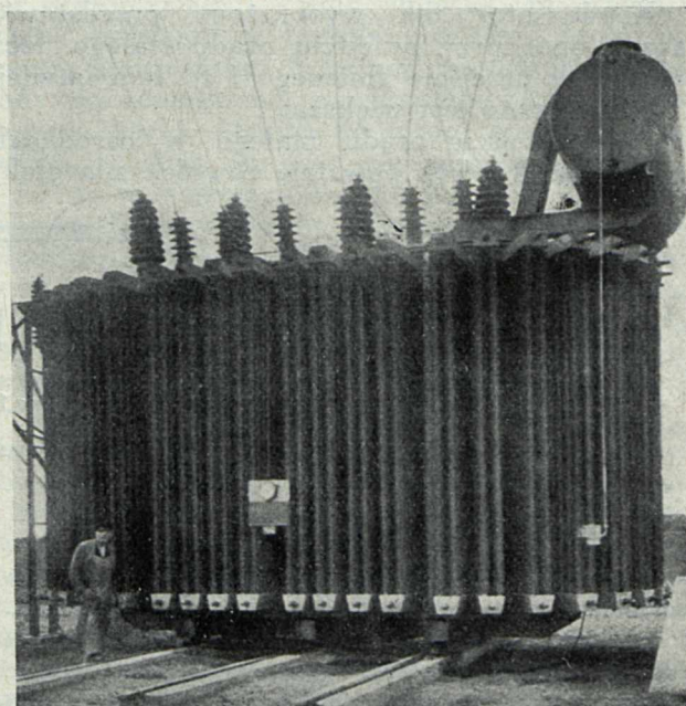
Rys. 2. Trójfazowy transformator olejowy z naturalnym chłodzeniem powietrznym o mocy 45 000 kVA, 126/57,5/52,5 kV (Asea).
