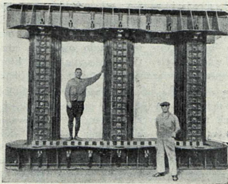
Rys. 3. Rdzeń transformatora o mocy 45 000 kVA (Asea).
