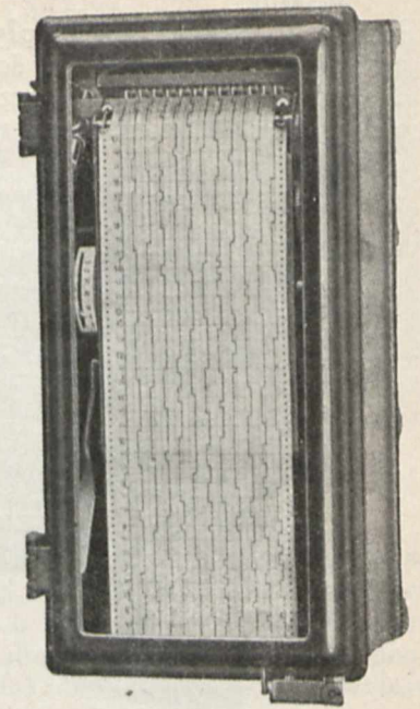
Rys. 5. Przyrząd samopiszący.
