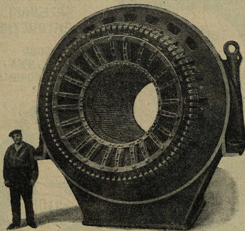
Stator turbogeneratorsa mocy 20 000 KVA, 300 obr/min. wykonany dla wodnej elektrowni w Erwienice
