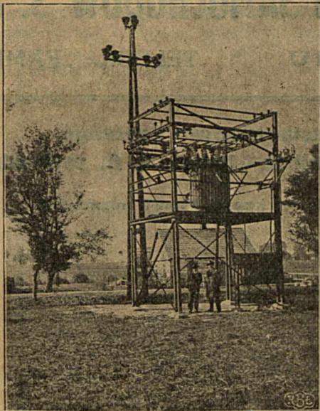
Transformator 160 KVA 33/6,3/0,4 kV.
