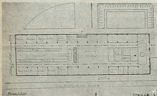
Rys. 2. Plan hali Nr. 1 z oznaczeniem stoisk poszczególnych przedsiębiorstw.
