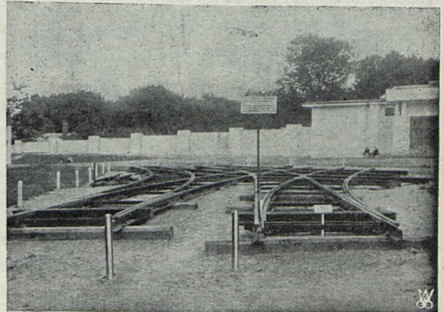
Rys. 10. Rozjazd z szyn Zakładów Ostrowieckich, wykonany przez Tramwaje Warszawskie.
