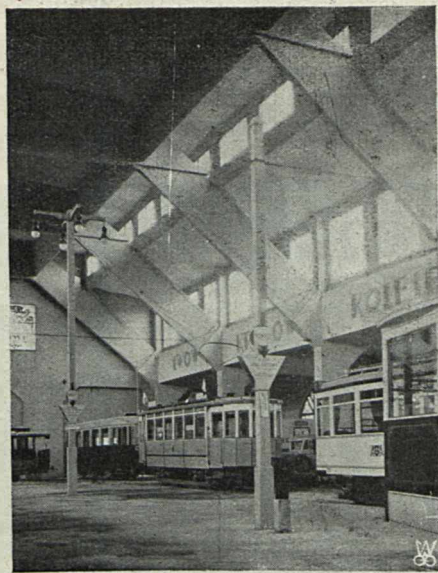
Rys. 5. Słupy stalowo-betonowe Poznańskiej Kolei Elektrycznej.
