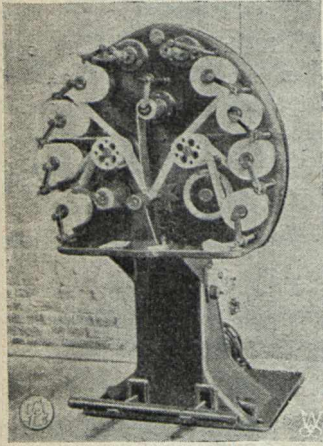
Rys. 5. Maszyna do nawijania ogniw. Zagłębiu Dąbrowskiem:
