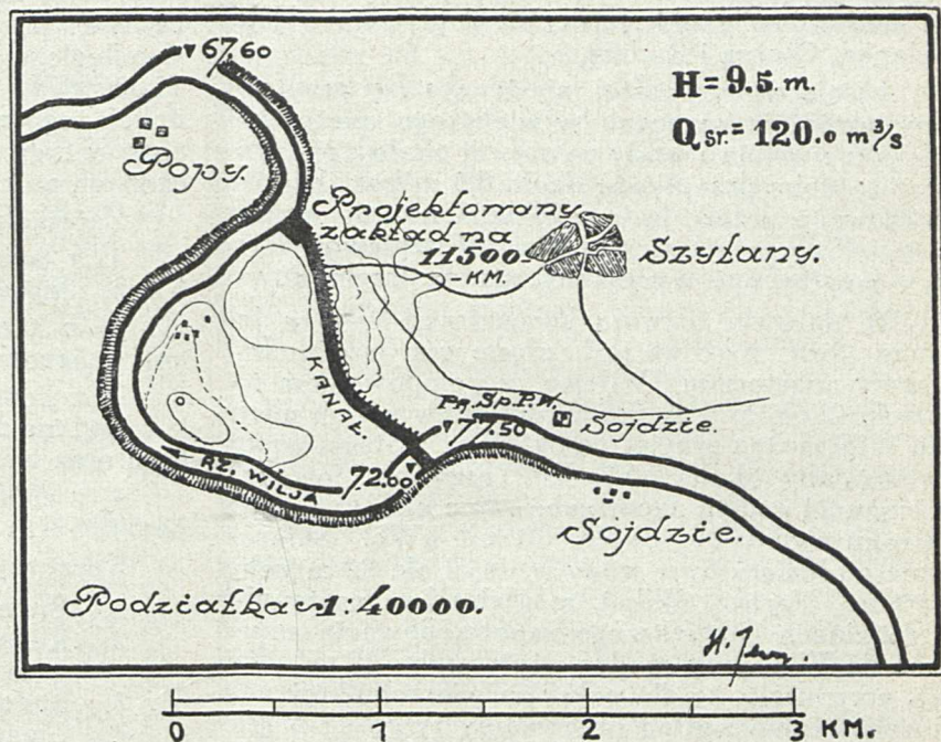
Rys. 7. Schemat zakładu wodnego na Wilejce.
