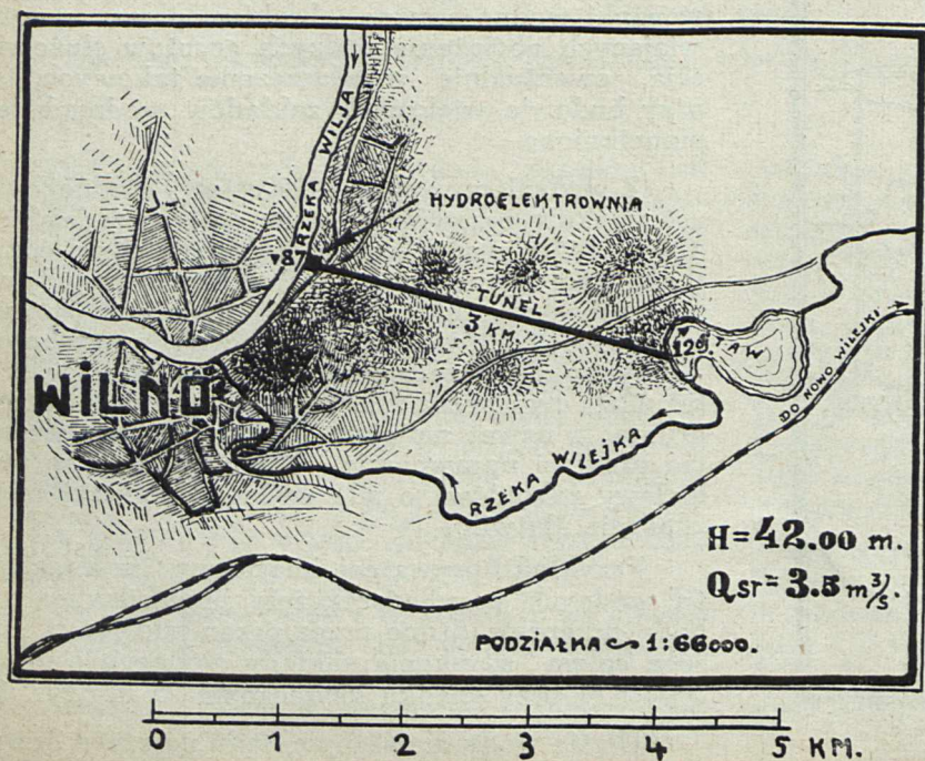
Rys. 3. Schemat wyzyskania rz. Wilji przy Szyłanach.
