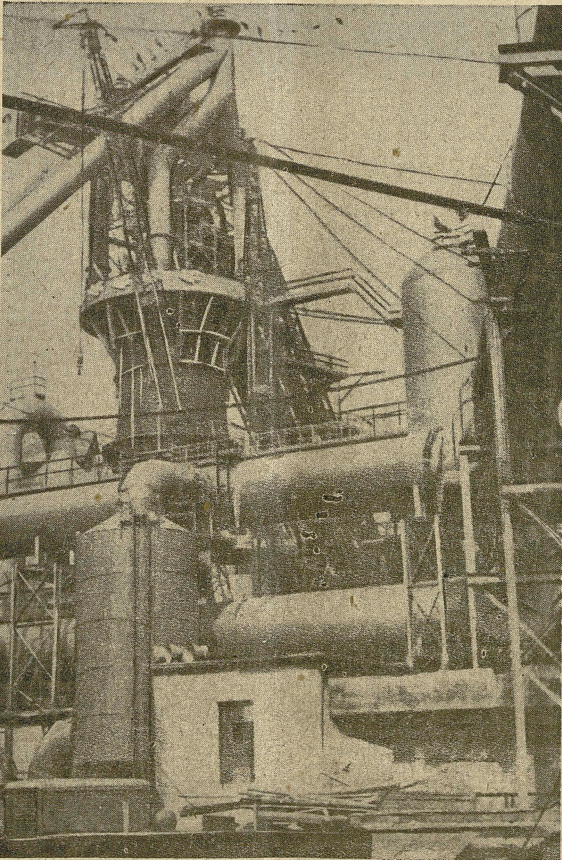
Na 142 dni przed terminem uruchomiony został wielki piec „B” w hucie „Kościszko”
