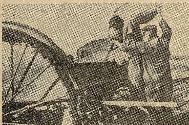
Przygotowanie siewnika do siewu w PGR Rusocin (woj. gdańskie). Foto — WAF.
