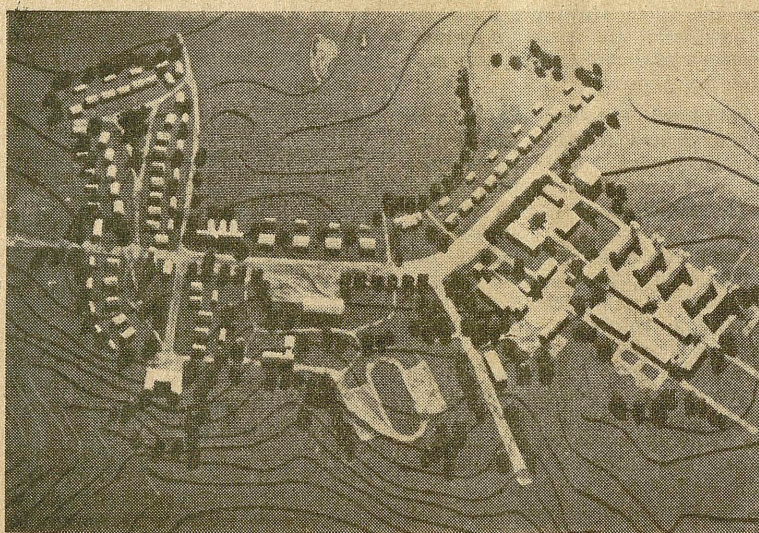
Projekt rozplanowania osiedla przy Państwowym Gospodarstwie Rolnym. Droga komunikacyjna przecina wieś, nie naruszając jej wewnętrznej struktury. Ośrodek produkcyjny i kulturalno-społeczny położone właściwie w stosunku do mieszkań. Osiedle tego typu różni się od wsi spółdzielczych zarówno liczbą działek siedliskowych jak i brakiem przyzgodowych działek rolnych. Osiedle ma charakter skupiony, a więc posiada warunki stosunkowo łatwego urządzenia ulic.
