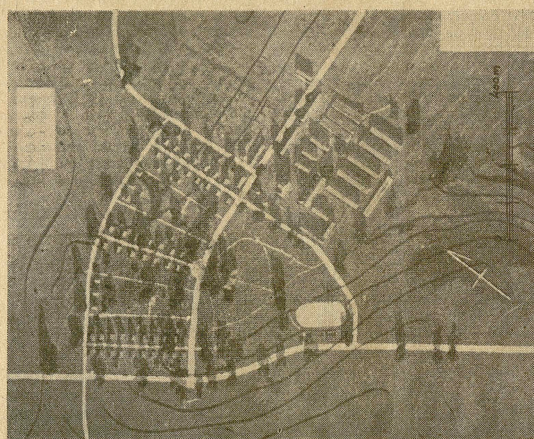
Rozplanowanie osiedla przy Państwowym Gospodarstwie Rolnym. Droga komunikacyjna omija osiedle, a jego połączenie z osiedłem produkcyjnym prowadzi przez ulicę, stanowiącą centrum współżycia zbiorowego wsi. Znaczenia nabiera droga, łącząca ośrodek produkcyjny z szosą poza placem sportowym, przejmując z niego znaczną część gospodarczego ruchu. Wzajemny układ części składowych osiedla służy a ich niezależny rozwój terytorialny możliwy.
