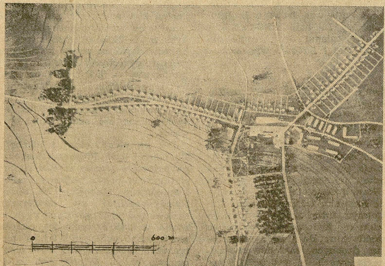
Projekt rozplanowania wsi spółdzielczej. Założenie planu zgodne z naturalnymi warunkami terenu. Droga komunikacyjna wkracza w partii wschodniej w ulicę mieszkaniową. Dobre rozwiązanie centrum wsi i wzajemnego położenia poszczególnych jej elementów. Przyjęcie zasady ścisłej łączności z działkami przyzgodowymi. Pomysłowość w usytuowaniu budynków podnosi plastyczne walory osiedla.
