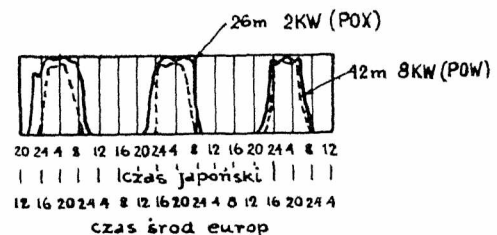
Rys. 8. Trzydniowe próby Nauen—Osaka (9 000 km).
