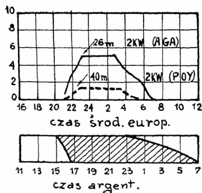
Rys. 7. Nauen—Buenos Aires (12 000 km).
