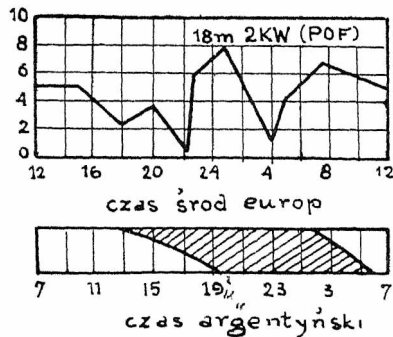
Rys. 11 Próby Nauen—Buenos Aires (12 000 km),
