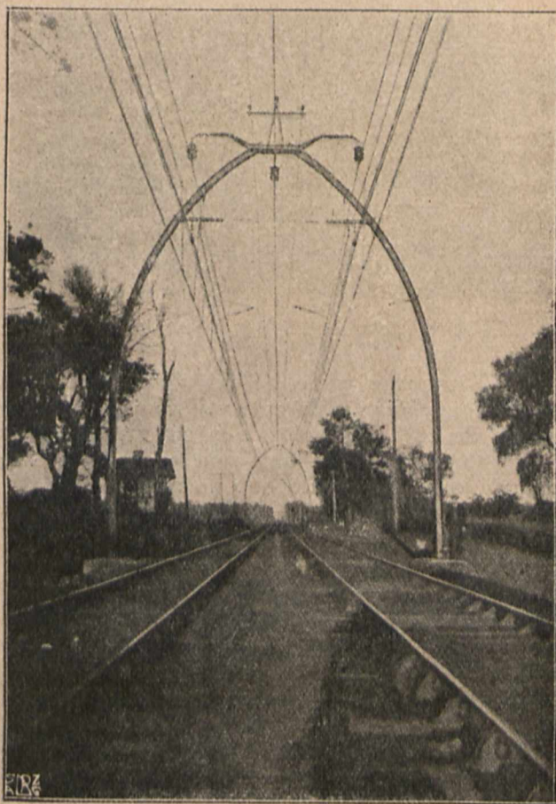
Fig. 8. Bramki profilowe sieci roboczej z linją 60 000 i 10 000 V (T-wa „Midi”).
