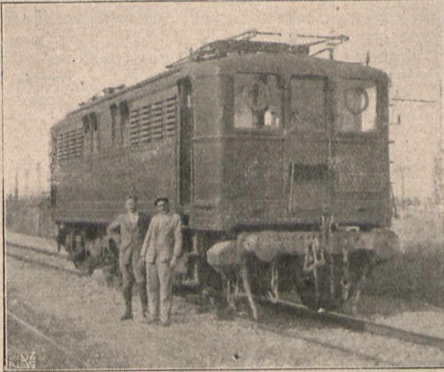
Fig. 9. Lokomotywa BB, T-wa „Midi”.
