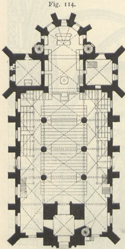
Marien-Kirche zu Wolfenbüttel 174) .
