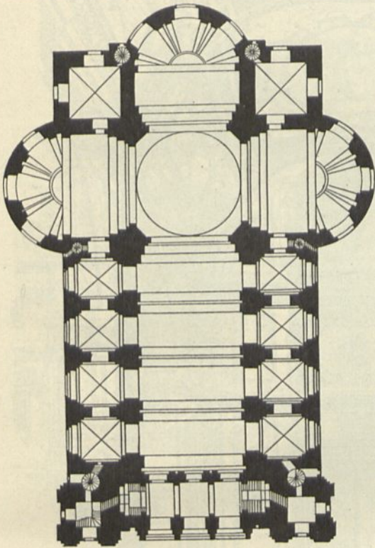
Grundriß des Domes zu Salzburg 157) .
