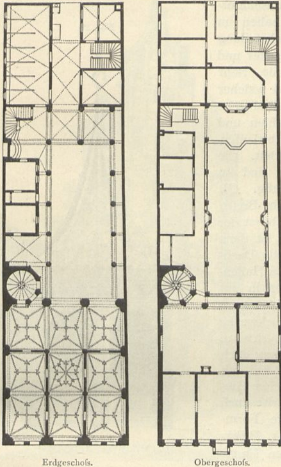
Erdgeschoß. Obergeschoß. Grundrisse des Peller-Hauses zu Nürnberg 53) . \frac{1}{100} w. Gr.
