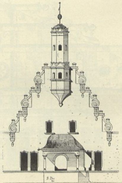
Giebel am Barthelshof zu Leipzig 203) .
