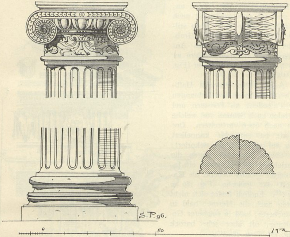
Jonische Säule im Schloß zu Baden 244 .
