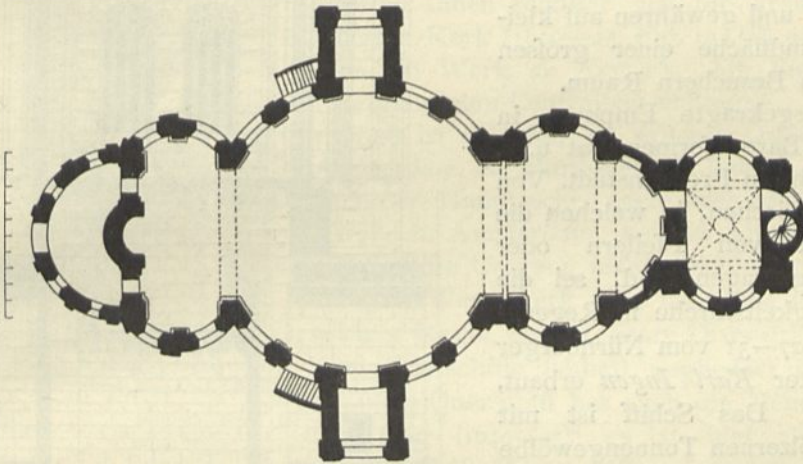
Grundriß.
