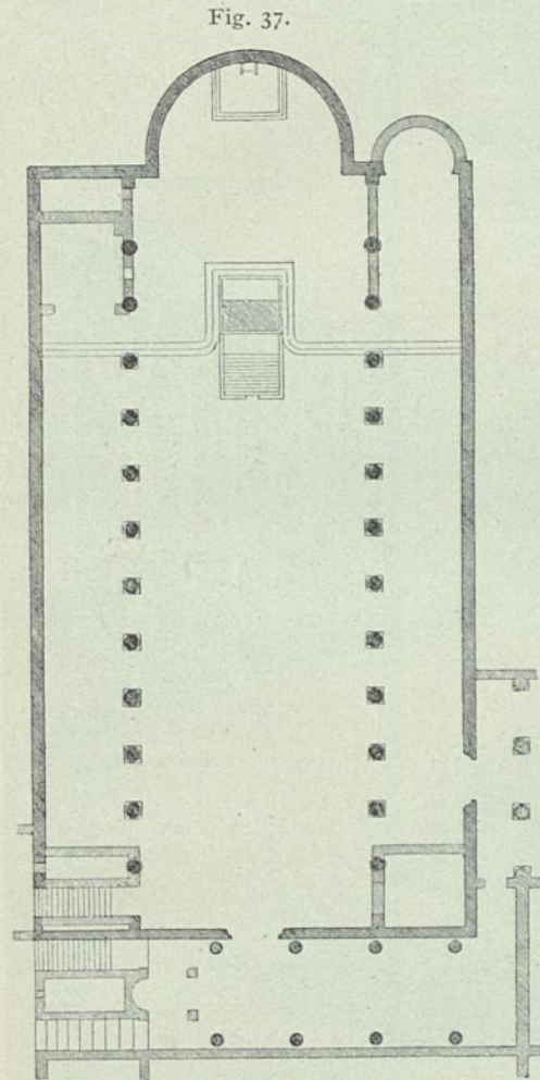
Santa Sabina zu Rom. Grundriß 29 ). — \frac{1}{100} w Gr.
