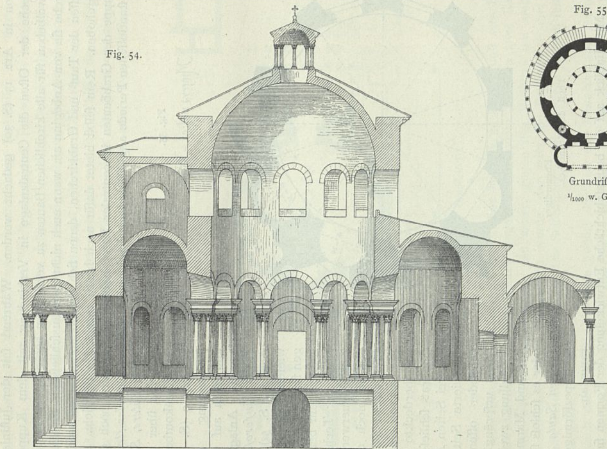
Schnitt. — \frac{1}{250} w. Gr.
