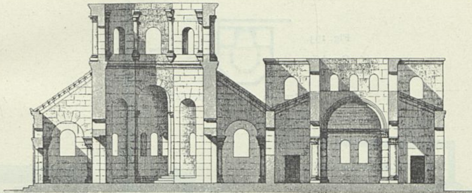
Schnitt nach XY. — \frac{1}{300} w. Gr.
