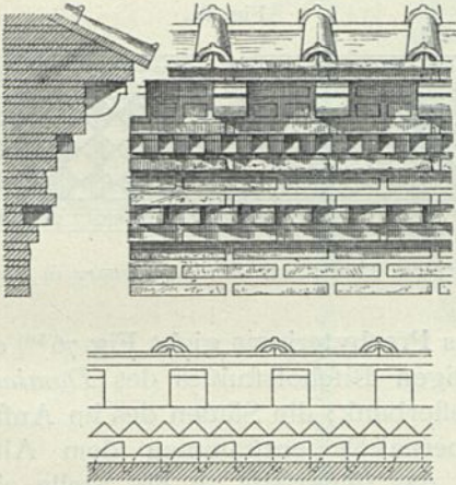
Gefimse von Santo Stefano rotondo zu Rom.
