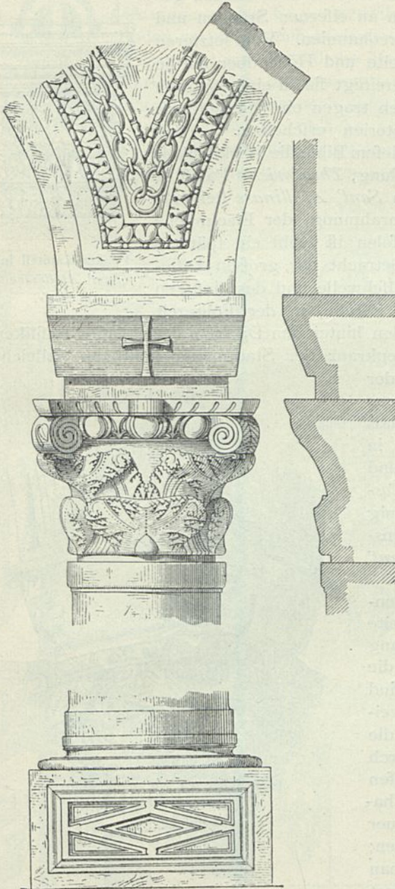
Säulen-Kapitell und -Basis in Sant' Apollinare in Classe.
