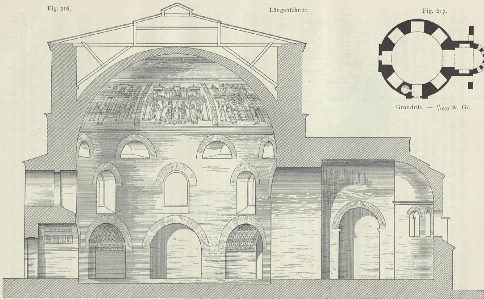
St. Georgs-Kirche zu Theffalonich 82) .
