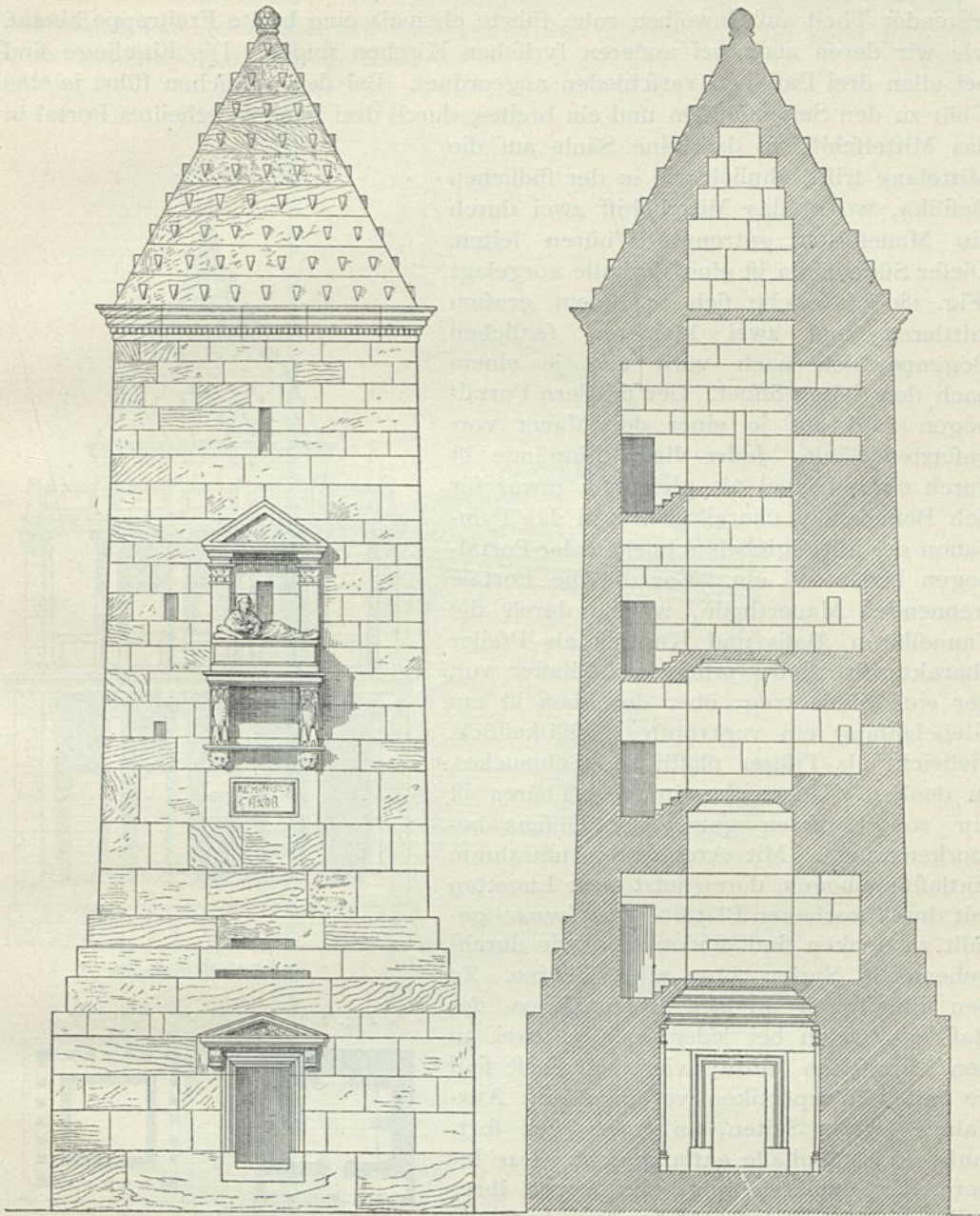
Grab des Jamlichus zu Palmyra 78) . Wiederherstellung. — \frac{1}{200} w. Gr.
