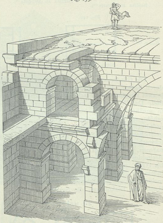
Aufbau.
