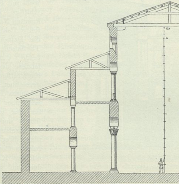
Querchnitt.
