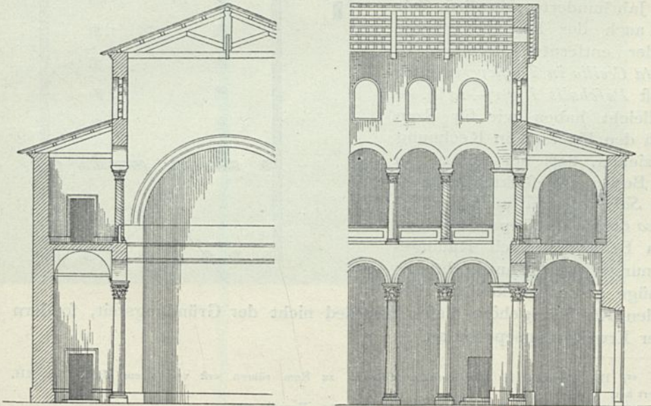
System 31) . — \frac{1}{250} w. Gr. Sant' Agnese bei Rom.
