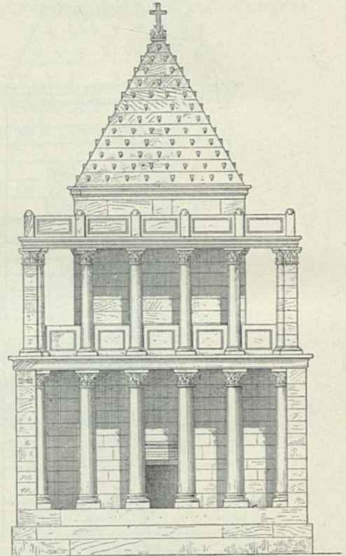
Vorderansicht. — 1/200 w. Gr.
