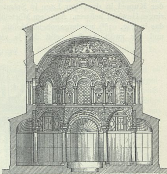
Schnitt 54) .
