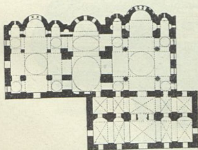
Pantokrator zu Constantinopel. 1/1000 w. Gr.
