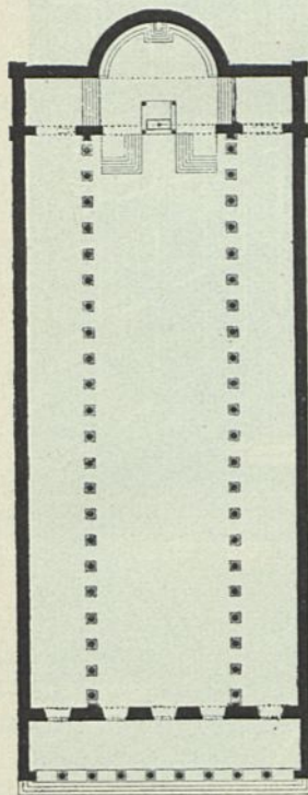
Santa Maria Maggiore zu Rom. Grundriß 27) . — \frac{1}{1000} w. Gr.
