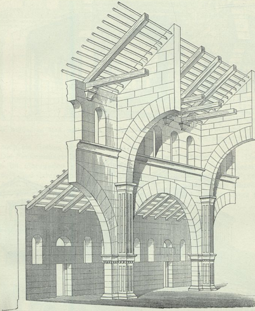
Basilika zu Ruweha. — Aufbau 78) .
