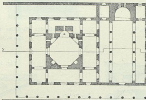
Baptisterium zu Kalat-Sim'an 78 ).
