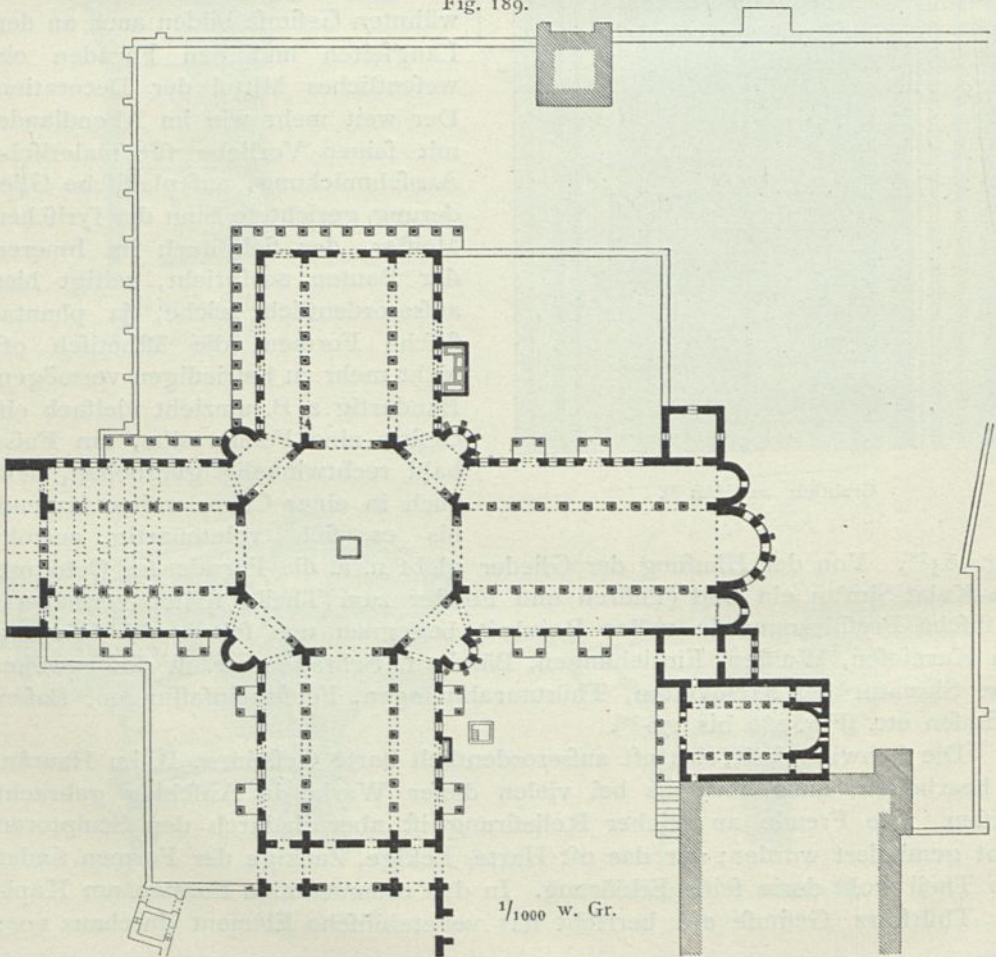
Kirche zu Kalat-Sim'an. — Grundriss 78) .
