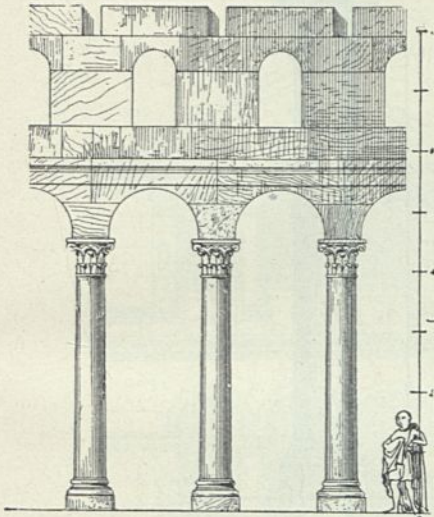
Von der Basilika zu Mudfcheleja 78 ).
