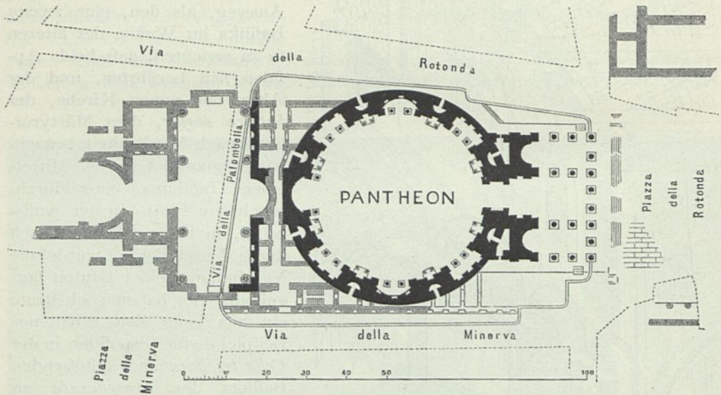
Pantheon zu Rom. — Grundriß 87 ).
