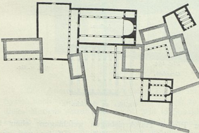
Basilika und Nebenbauten zu Chirbet-Hâfs 78) .
