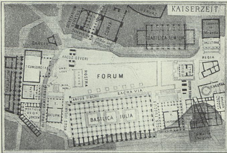
Forum und Basilica Julia zu Rom 18) .
