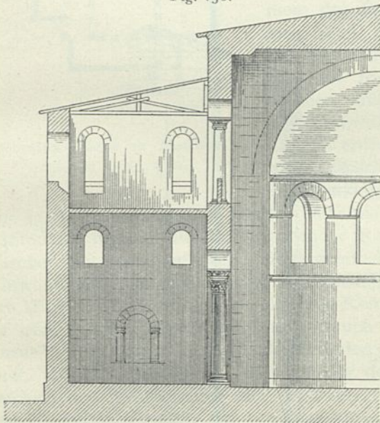
Querschnitt.
