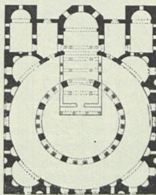
Grundriss. — 1/1000 w. Gr.
