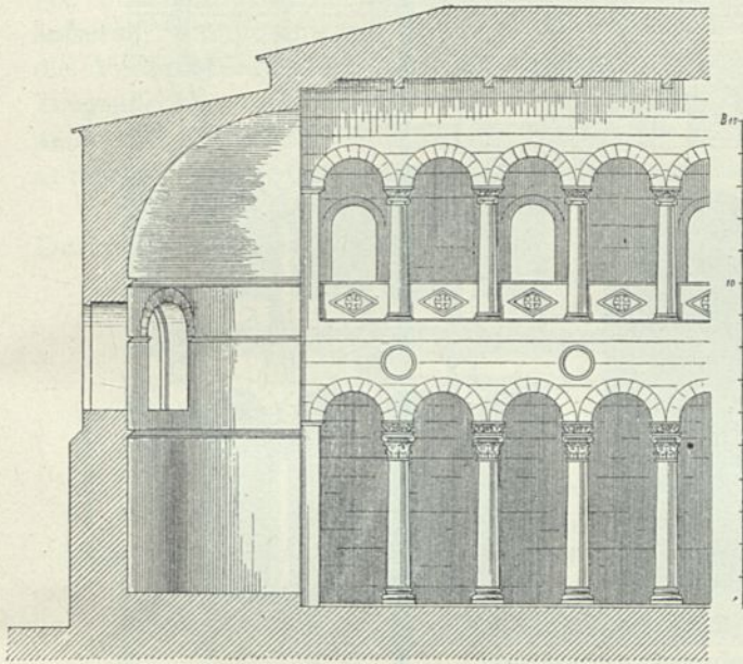
Längenschnitt.
