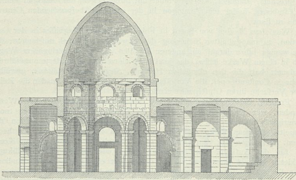
Längenschnitt.
