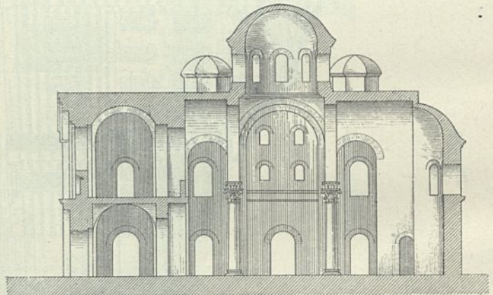
Längenschnitt 89 ).
