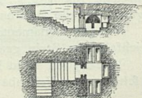
Grab des Malchus zu El-Bara 78).
