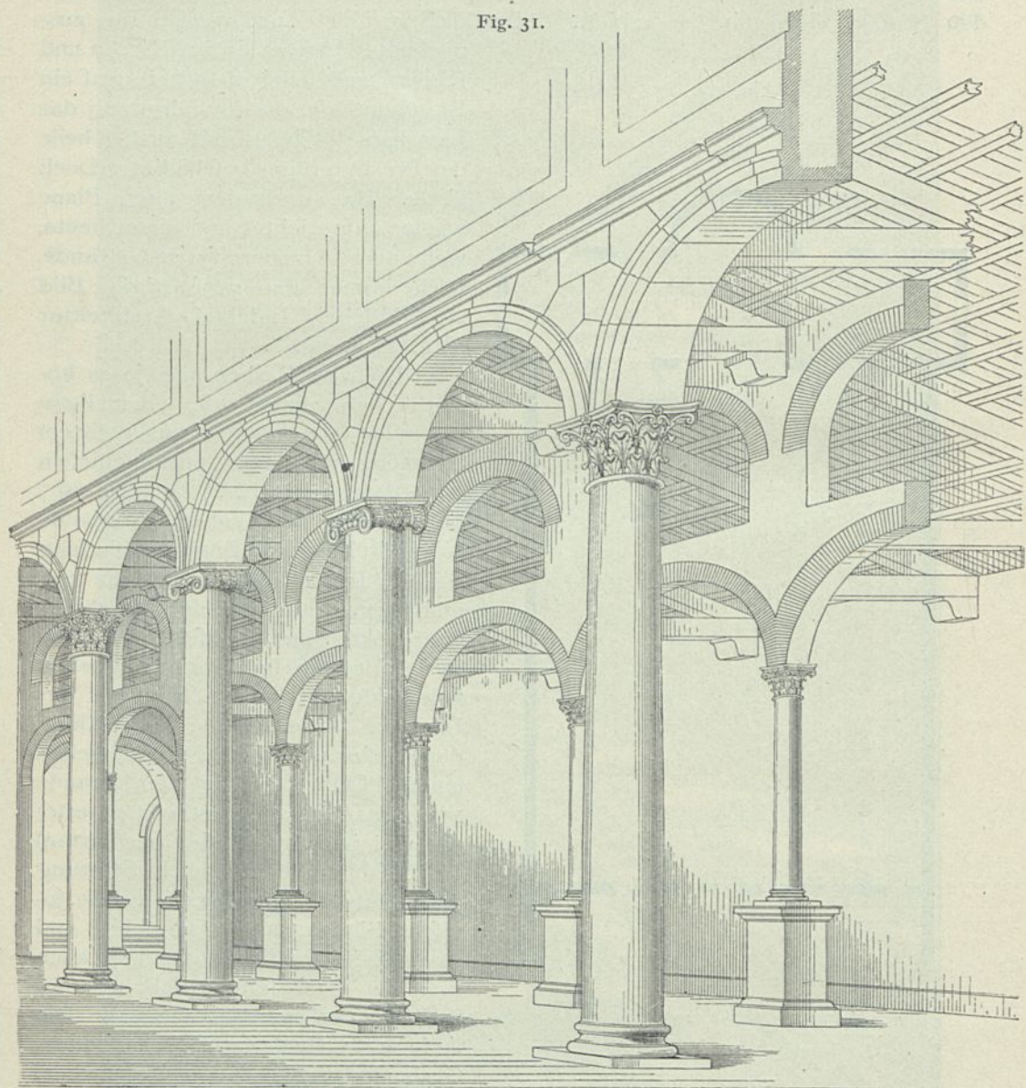
Lateran-Basilika zu Rom. System des Inneren 20) .
