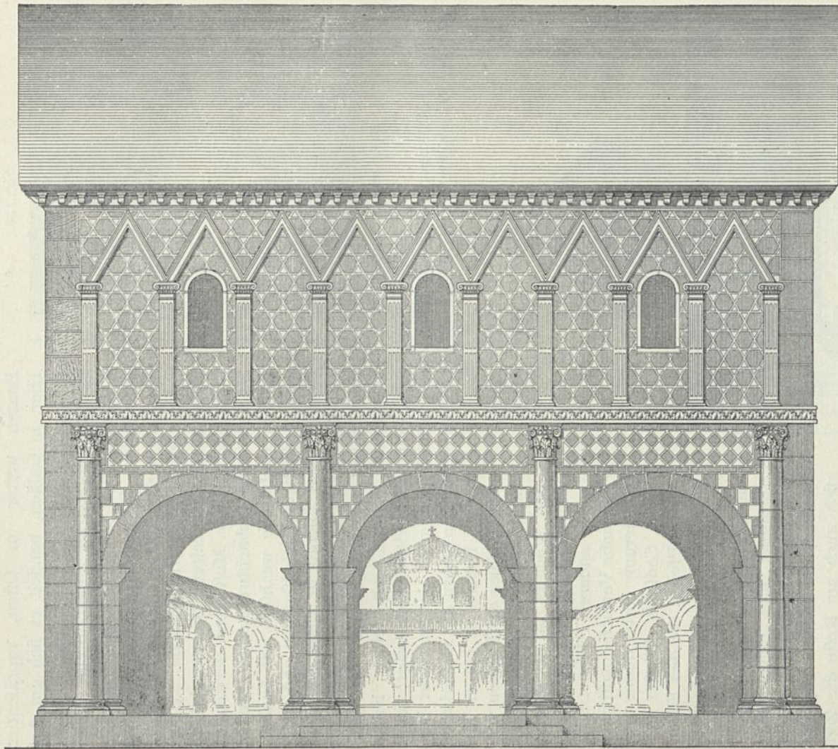
Atriums-Vorhalle zu Lorch (Ehemaliger Zustand 53 ).
