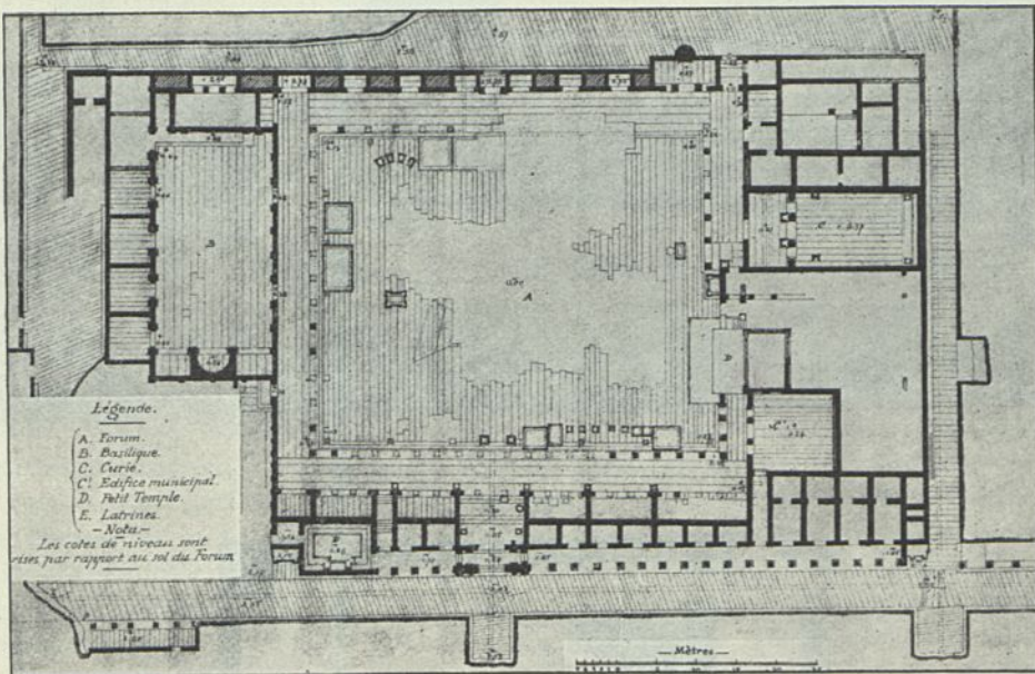
Forum und Basilika zu Timgad 10) .
