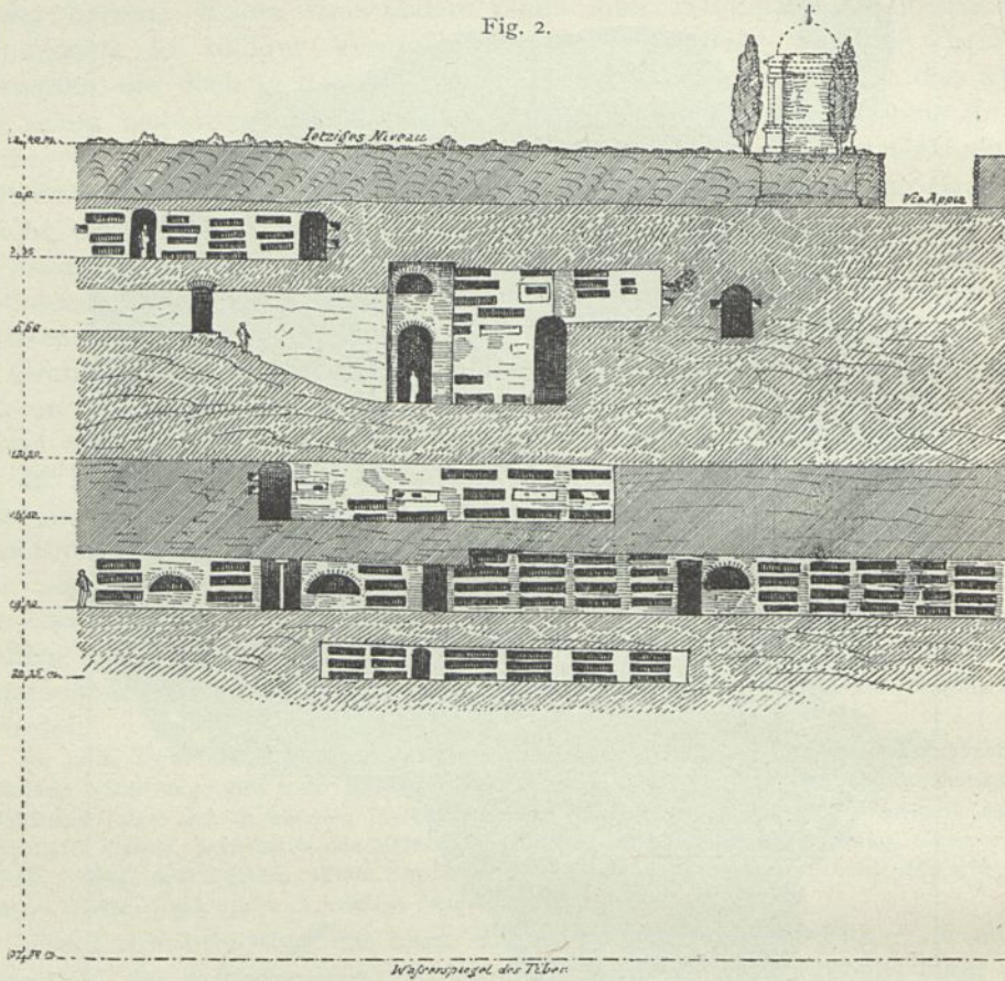
Durchschnitt der Katakomben von San Callisto 4) .
