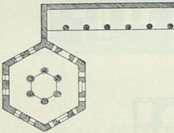
Centralbau zu Dér-Seta 78), 1/500 w. Gr.
