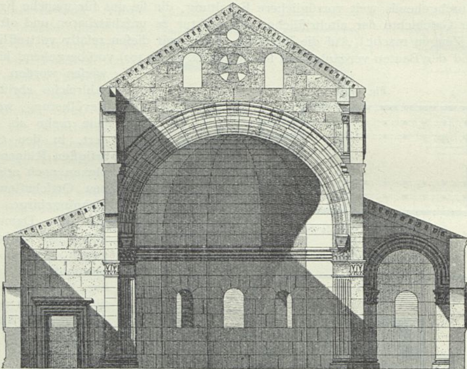
Querschnitt. — \frac{1}{200} w. Gr.
