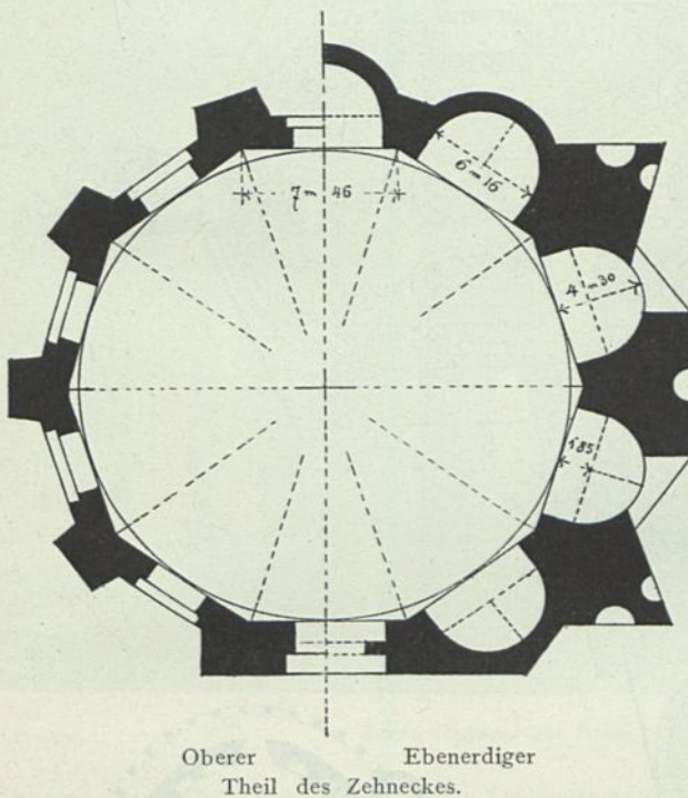
Fig. 53. Minerva medica - Rom.
