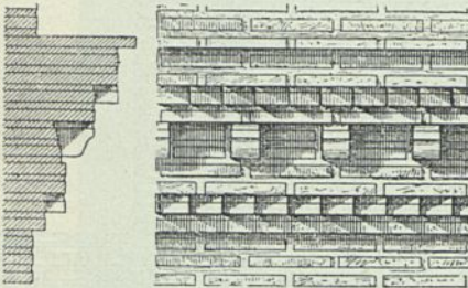
Gefimfe von Santa Balbina zu Rom 51) .
