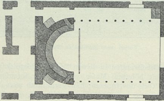
Basilika im Flavier-Palaft zu Rom.
