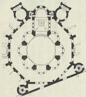
Grundriß. — \frac{1}{1000} w. Gr.
