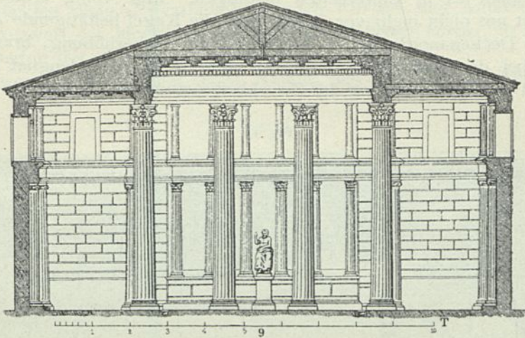
Querchnitt 16) .
