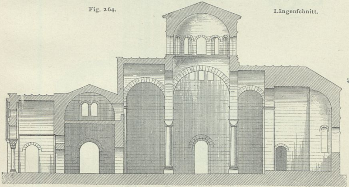
Sophien-Kirche zu Trapezunt.
