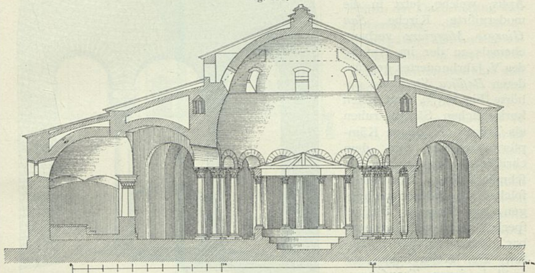
Durchschnitt.
