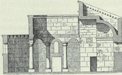
Fig. 192. Längenschnitt.
