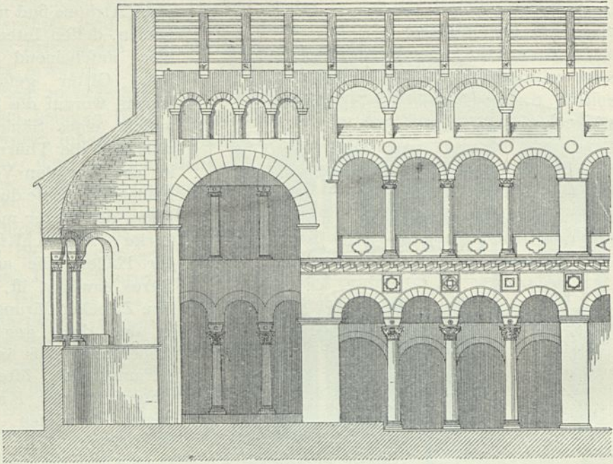
Längenschnitt.
