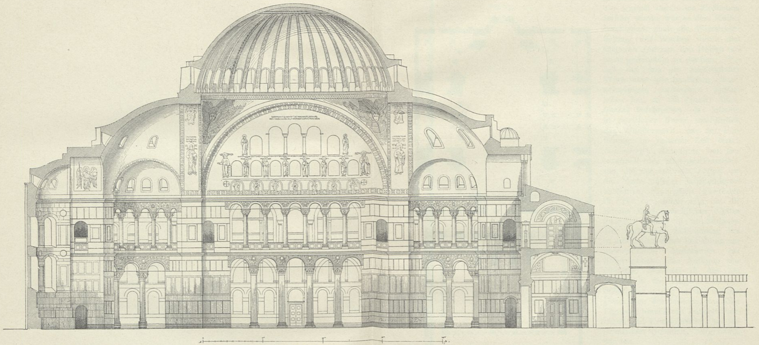
Sophien-Kirche zu Constantinopel.
