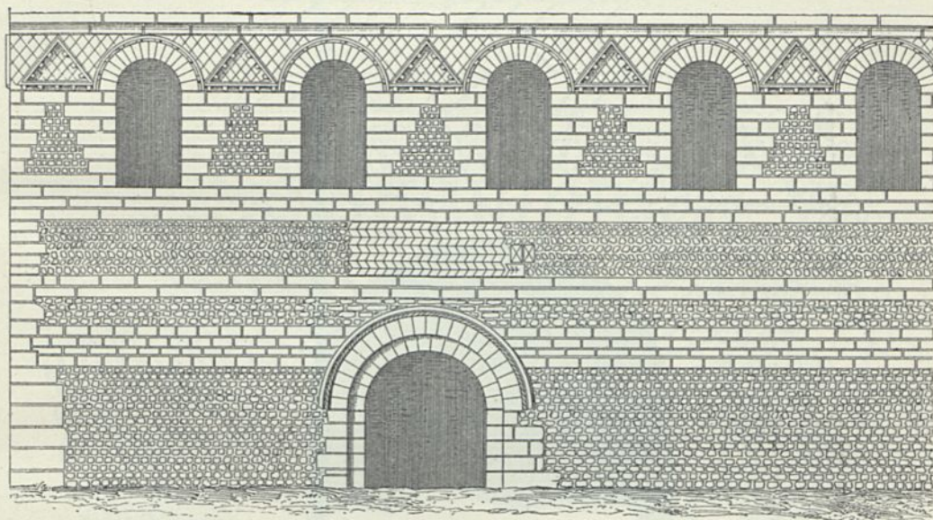
Südseite der Kirche zu Cravant 65 ).
