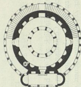
Grundriß. \frac{1}{1000} w. Gr.
