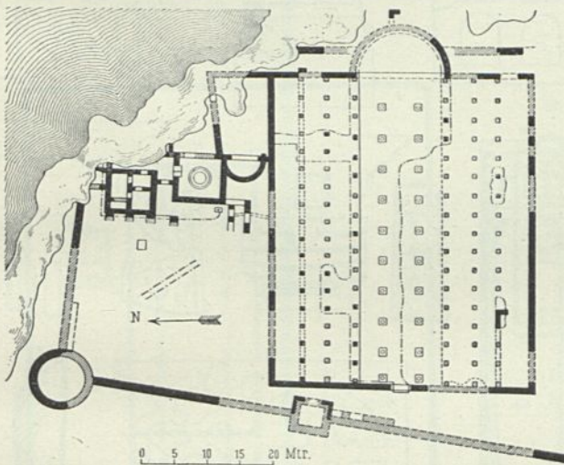
Bafilika zu Tipaſa 75) .
