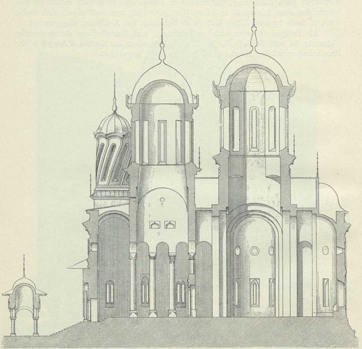
Längenschnitt.
