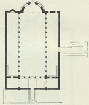
Eski Dschuma zu Theffalonich. Grundriß 71 ). — 1/1000 w. Gr.
