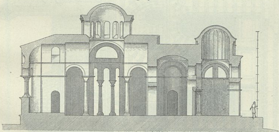
Längenschnitt.
