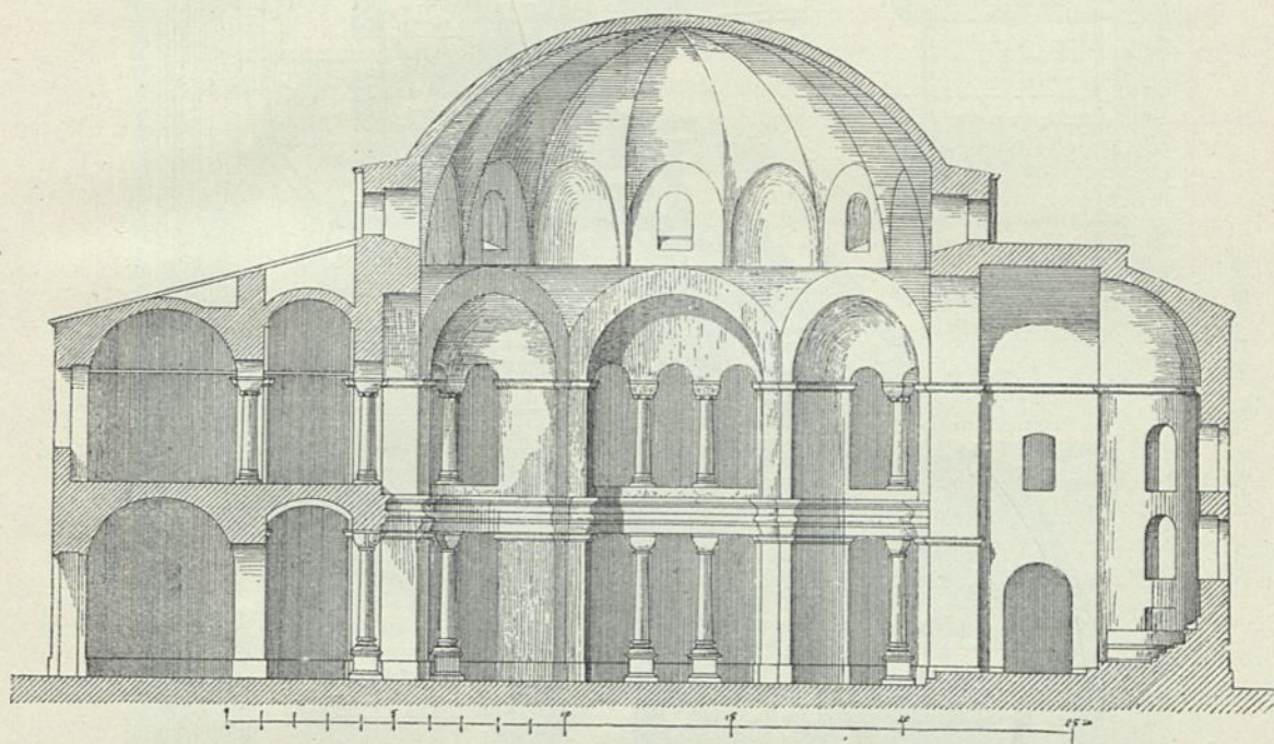
Längenschnitt.
