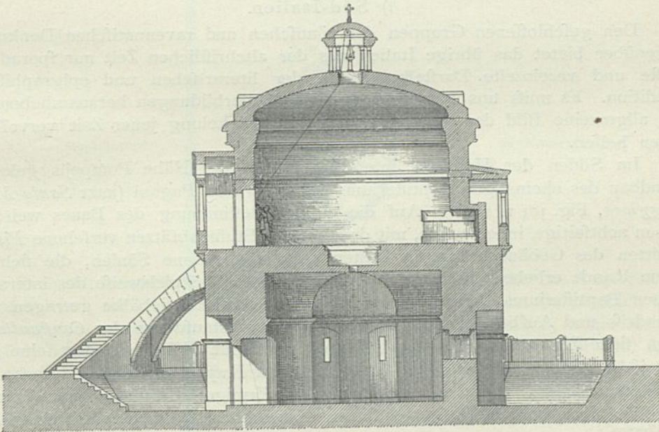
Durchschnitt.
