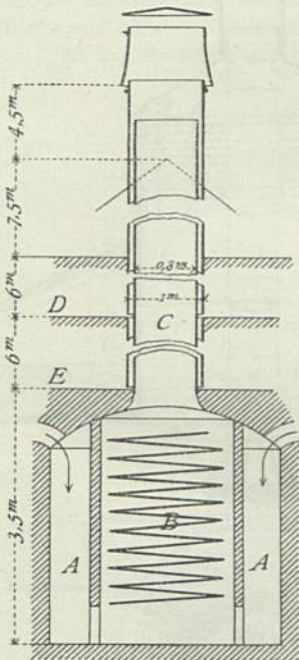
Lockschornstein im Krankenhause zu Amsterdamm. — \frac{1}{100} w. Gr.
