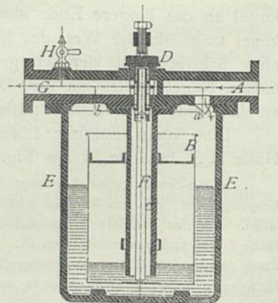
Selbstfleerer von Dreyer, Rosenkranz &amp; Droop in Hannover.
