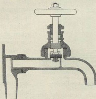
Niedererschraubhähne.
