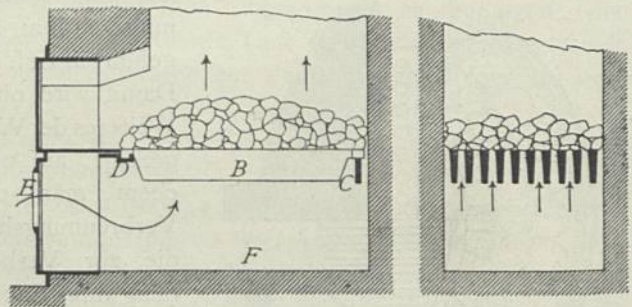
Feuerstelle mit Planrost. — \frac{1}{10} w. Gr.
