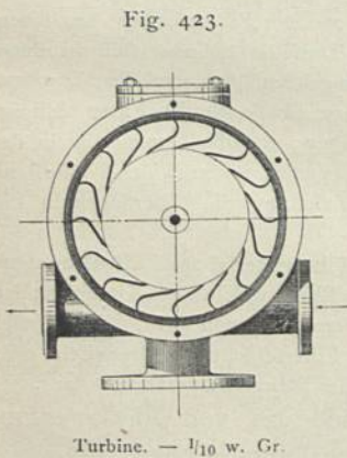
Turbine. — 1/10 w. Gr.
