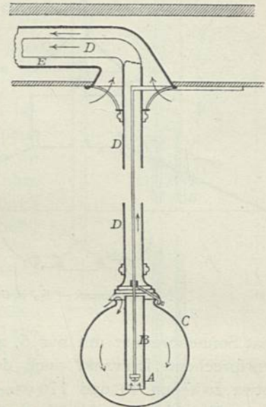
Ricketts' Kugellicht. (Benham & Sons in London.) 1/15 w. Gr.
