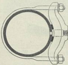
Rohrfchelle. — \frac{1}{10} w. Gr.
