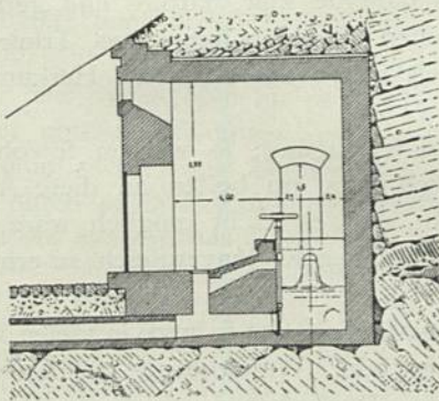
Einsteigekammern. — 1/150 w. Gr.
