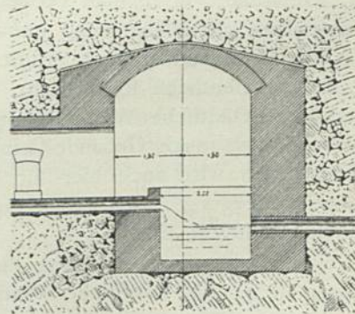
Einsteigekammern. — 1/150 w. Gr.
