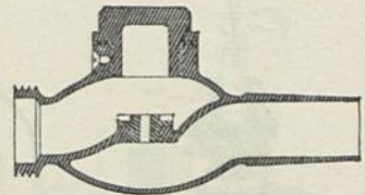
Kaliberhahn. — \frac{1}{3} w. Gr.
