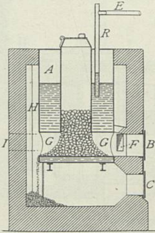
Niederdruck-Dampfkeessel von Bechem & Poß in Hagen.
