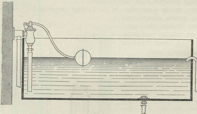
Dienstbehälter. — \frac{1}{20} w. Gr.
