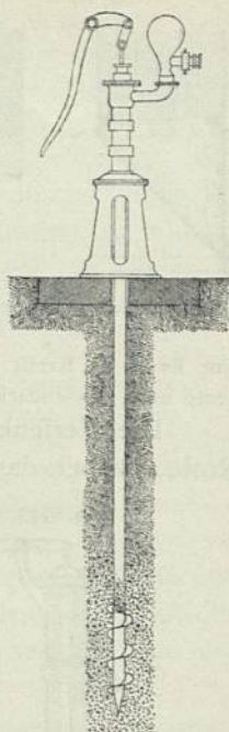
Abessinier-Brunnen. 1/60 w. Gr.
