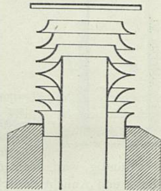
Saugkopf von Römheld.
