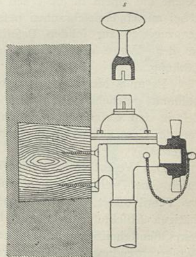
Feuerhahn. — \frac{1}{5} w. Gr.
