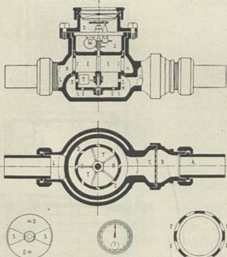
Wassermesser von Meinecke . — 1/10 w. Gr.
