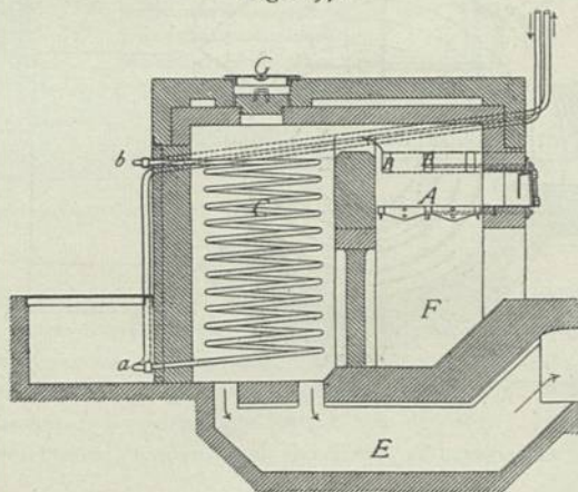
Feuerchlange für Hochdruck-Heizung. — 1/60 w. Gr.
