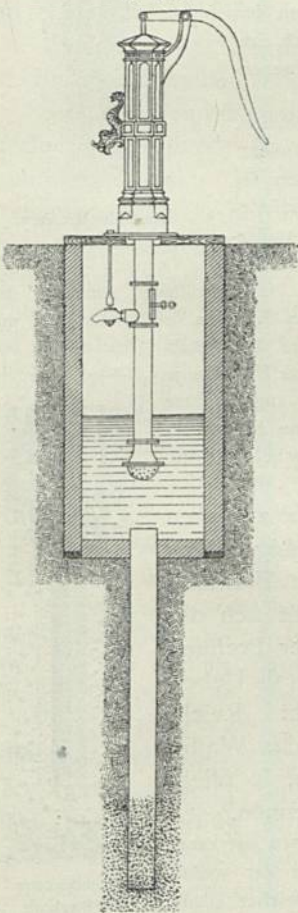
Röhrenbrunnen mit Saugschacht. \frac{1}{60} w. Gr.
