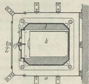
Halbfüllofen.
