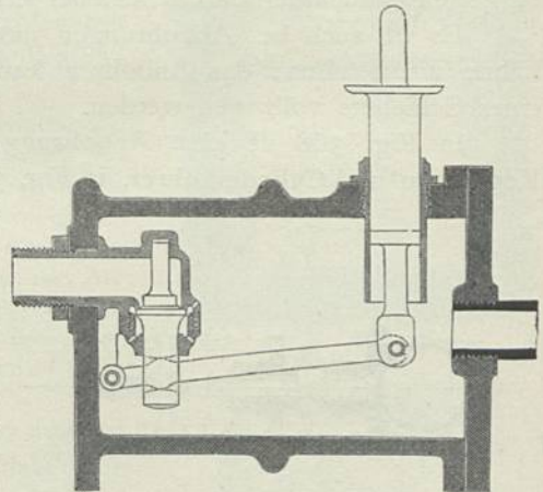
Druckverminderungs-Ventil. — 1/3 w. Gr.
