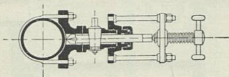
Anbohr-Werkzeug mit Hahn.
