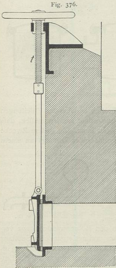
Einseitig schließender Schieber. — \frac{1}{25} w. Gr.
