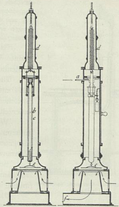
Selbstthätiger Regler von Bechem & Post .
