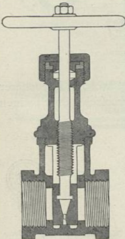
Peets-Ventil. — \frac{1}{3} w. Gr.
