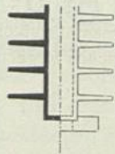
Heizkasten für Warmwasser-Heizung. \frac{1}{10} w. Gr.
