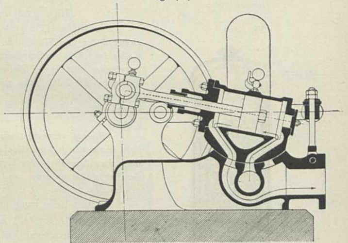
Schmid'scher Motor. — 1/35 w. Gr.
