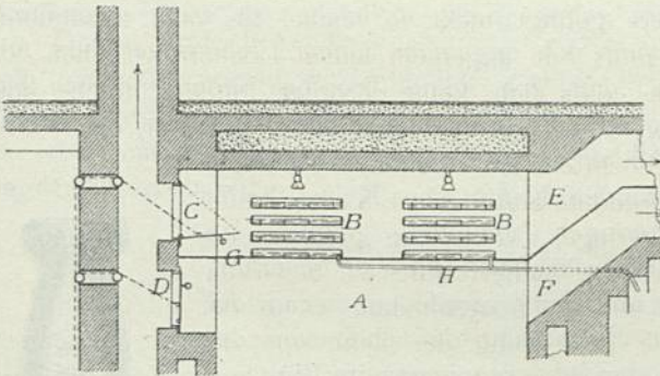
Luftanfeuchtungs-Apparat von Fischer &amp; Stiehl in Essen.
