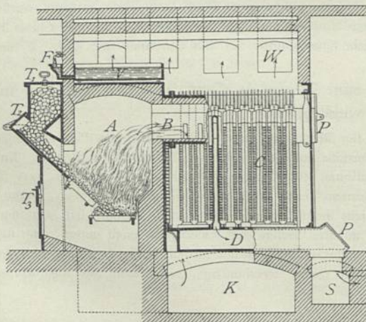
Luftheizungs-ofen von Gebr. Körting zu Hannover.
