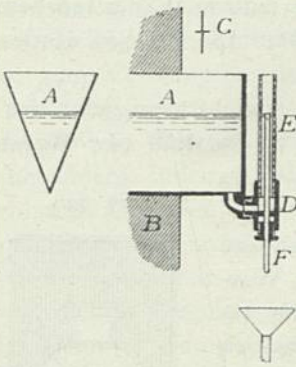
Luftanfeuchtungs-Schale von Hermann Fischer.
