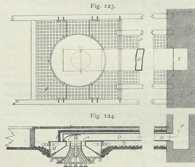
Lüftungs-Sonnenbrenner von Strode & Co. in London. — \frac{1}{35} w. Gr.
