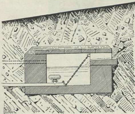
Einfachste Brunnenstube. — \frac{1}{100} w. Gr.
