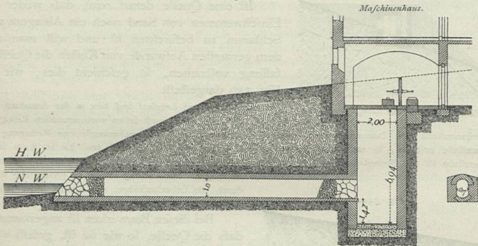
Wasserversorgung der Männer-Straf-Anstalt zu Pilsen aus dem Radbuza-Flusse. — \frac{1}{200} w. Gr.
