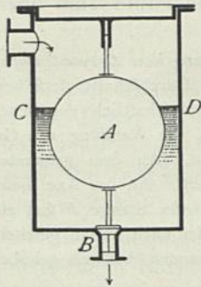
Selbstfleerer mit Schwimmkugel.
