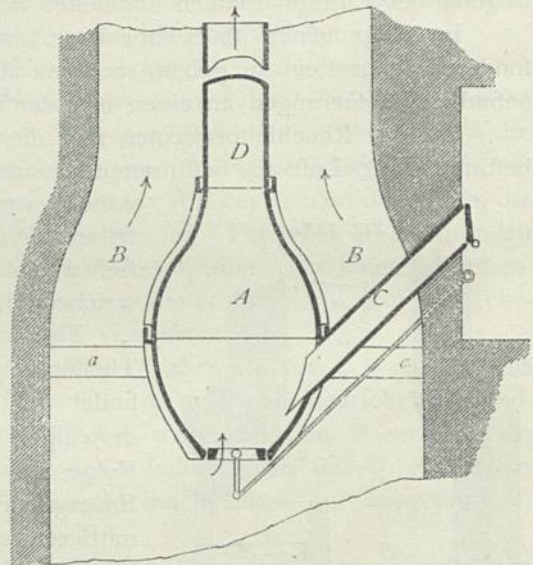
Lockschornstein mit Lockofen 146) . — \frac{1}{30} w. Gr.
