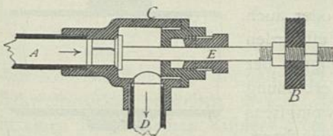
Selbstleerer.
