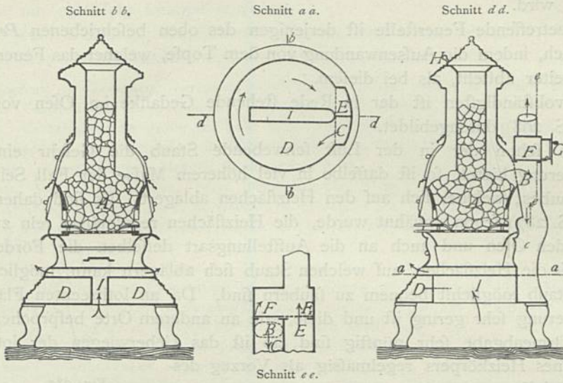
Perry's amerikanischer Ofen.
