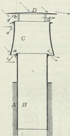
Luftfauher von Wolpert.
