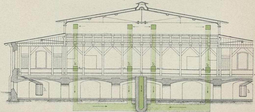
Schnitt durch den Speise, bezw. Gesellschaftssaal.
