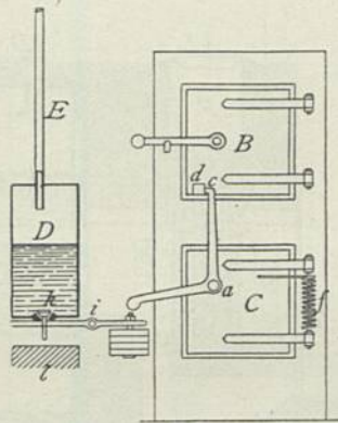
Niederdruck-Dampfkeessel von Bechem & Poß in Hagen.
