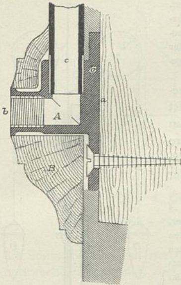
Wandfcheibe. — 1/2 w. Gr.
