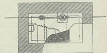
Privat-Hauptventil und Wassermesser. 1/50 w. Gr.
