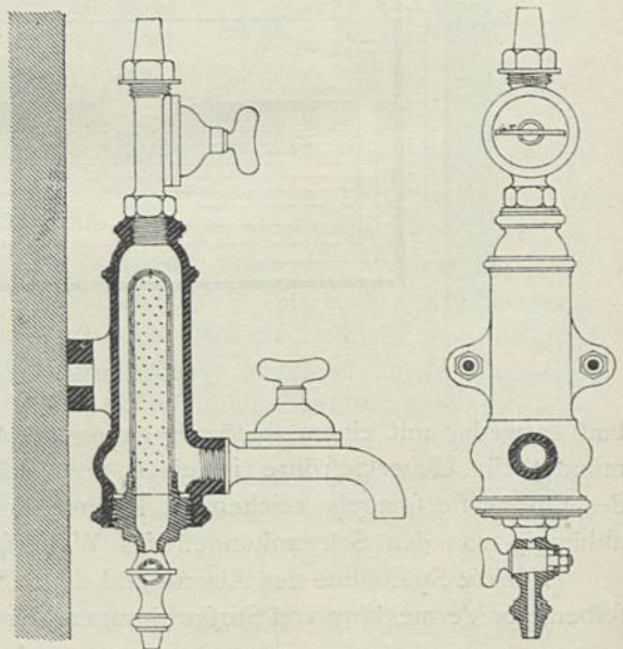
Filter von Salbach . — \frac{1}{5} w. Gr.
