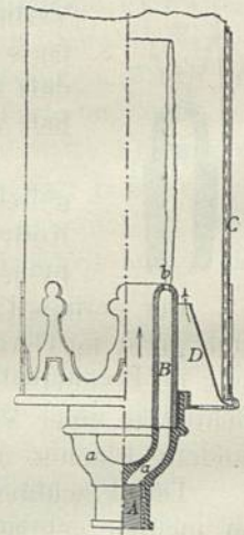
Argand-Brenner. — 1/2 w. Gr.
