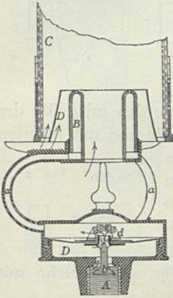
Argand-Brenner mit Druckregler. — \frac{1}{2} w. Gr.
