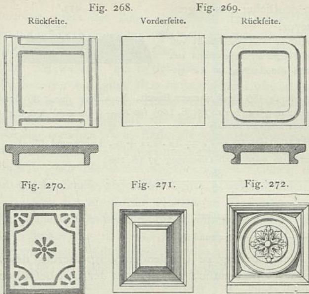
Kacheln. — \frac{1}{10} w. Gr.
