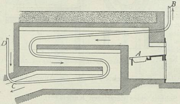
Wassererwärmer für Hochdruck-Heizung von Schinz . — \frac{1}{50} w. Gr.
