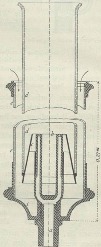
Brenner von Chauffenet . ½ w. Gr.
