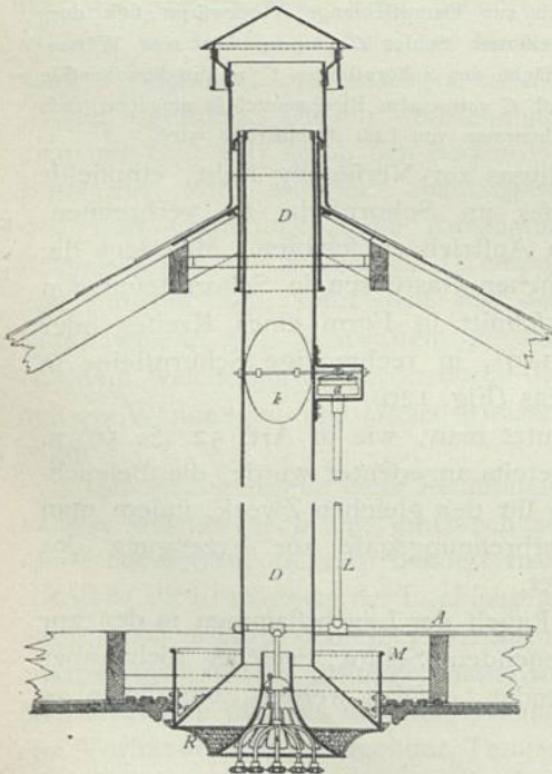
Lüftungs-Sonnenbrenner von Strode & Co. in London.
