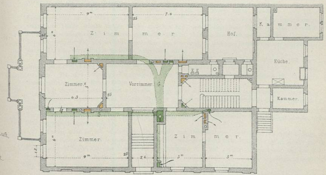
Erd - Geschoss.
