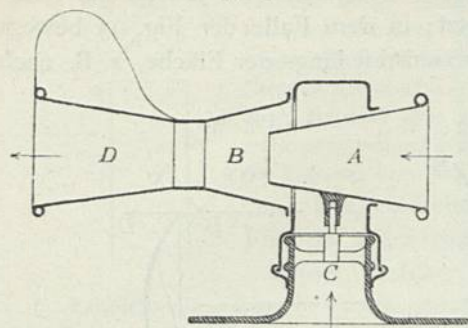
Luftfauger von Körting.
