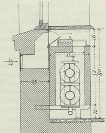
Regelungs-Einrichtung von Bechem & Post .
