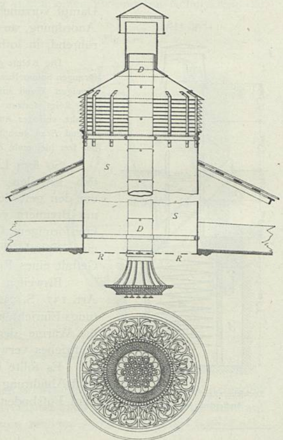
Lüftungs-Sonnenbrenner von Strode & Co. in London.
