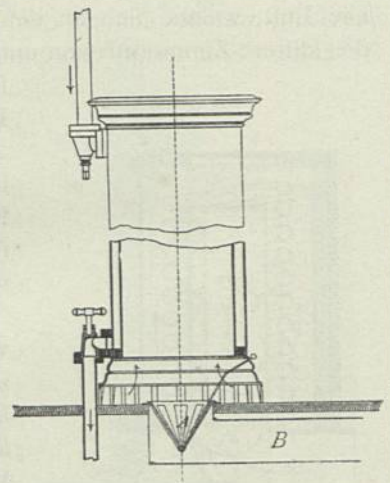
Ofen für Warmwasser-Heizung. — 1/20 w. Gr.
