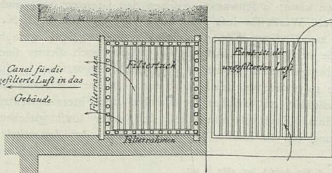
Filter von Möller in Brackwede bei Bielefeld.
