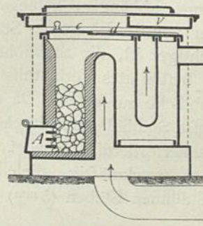
Irischer Ofen. — 1/30 w. Gr.
