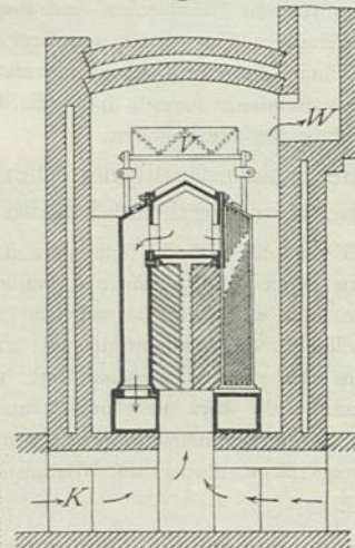
Luftheizungs-ofen von Gebr. Körting zu Hannover.
