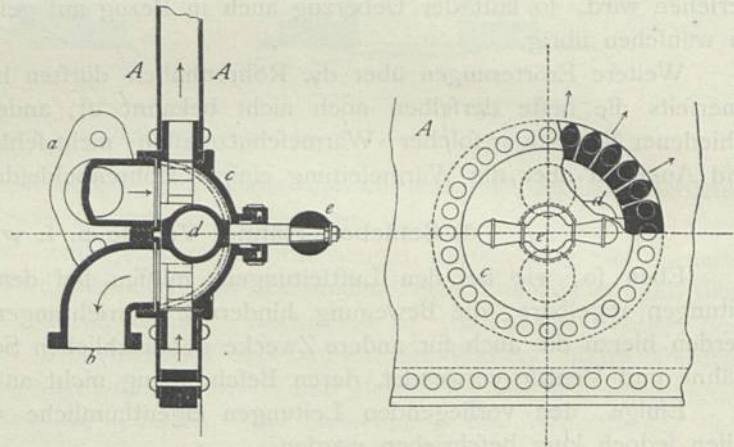
Wechselhahn von Hermann Fischer. — \frac{1}{5} w. Gr.
