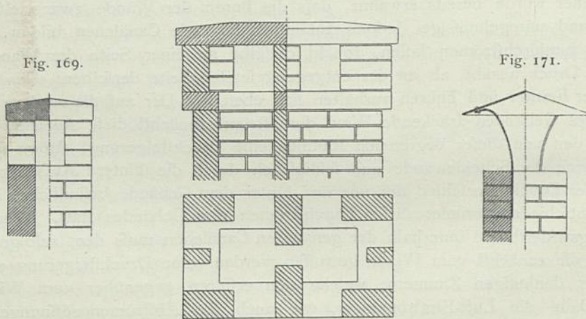
Schornsteinkappen. — \frac{1}{25} w. Gr.
