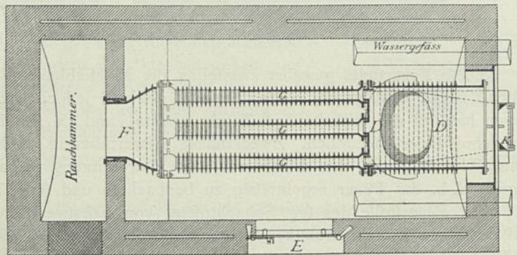
Schachtofen des Eisenwerkes Kaiserslautern. — \frac{1}{40} w. Gr.
