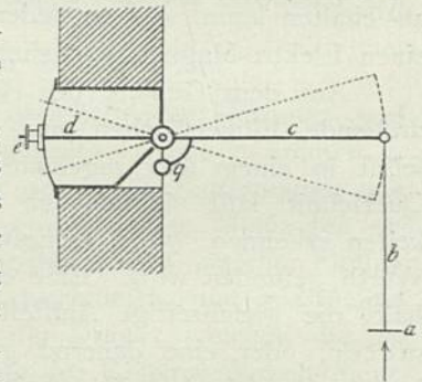
Luftgeschwindigkeitszeiger.
