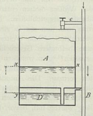
Regelungs-Einrichtung von Schweer.
