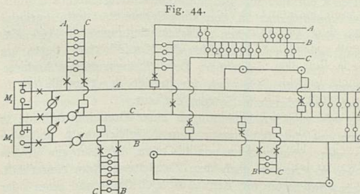
Schaltung im Dreileiter-System.
