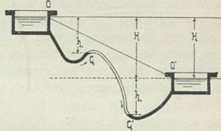
Längen-Profile von Druckleitungen.
