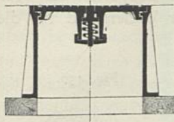
Deckel für Hydrantenröhren. — \frac{1}{25} w. Gr.
