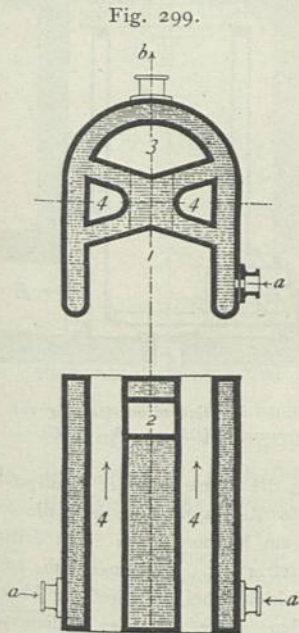
Heizkeffel für Niederdruck-Heizung von Hartly & Sugden .
