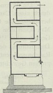
Zickzack-Ofen.
