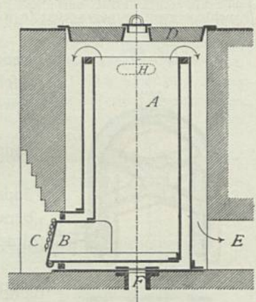
Heizkessel für Niederdruck-Heizung von Hermann Fischer. — 1/30 w. Gr.
