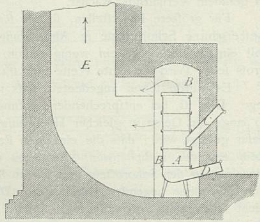
Lockschornstein mit Lockofen. — \frac{1}{100} w. Gr.
