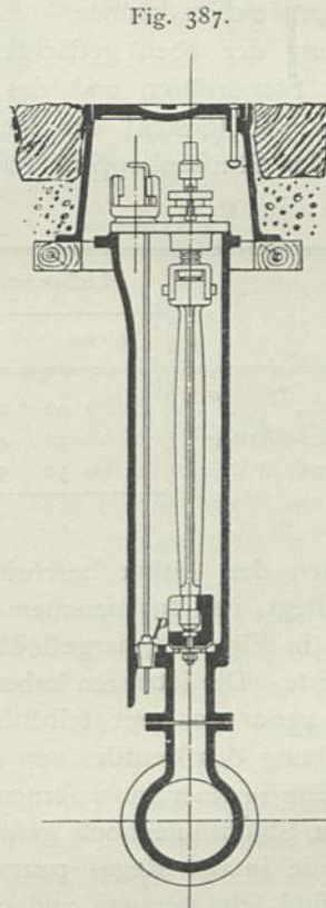
Hydrant ohne Selbstentleerung. \frac{1}{25} w. Gr.
