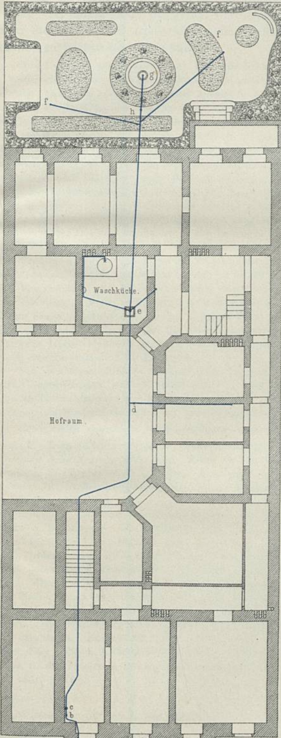
Grundriss des Kellergeschosses.
