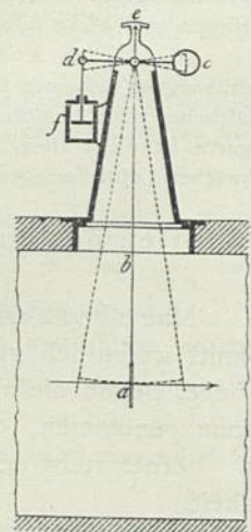
Luftgeschwindigkeitszeiger.
