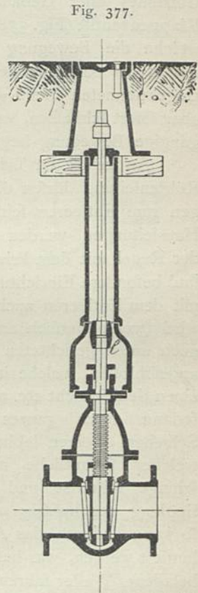
Doppelt schließender Schieber. — \frac{1}{25} w. Gr.
