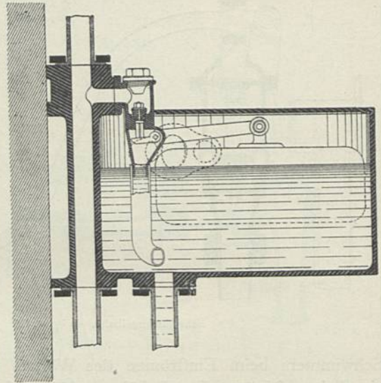
Behälter für Selbstschluß-Ventile von Fortin . — \frac{1}{5} w. Gr.
