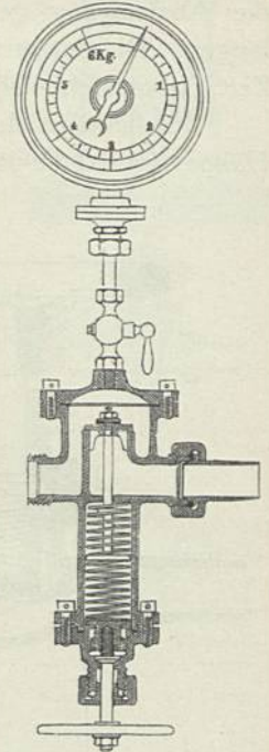
Druckverminderungs-Ventil. 1/5 w. Gr.
