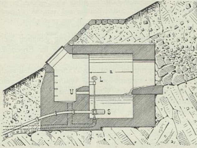
Einfache Brunnenstube. — \frac{1}{100} w. Gr.
