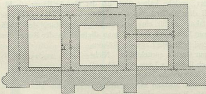
Haupt-Gasleitung im Gebäude der technischen Hochschule zu Hannover. 1/2000 w. Gr.
