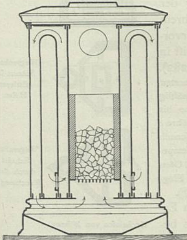
Ofen von Wehrenbold in Lühnen a. d. Lippe.
