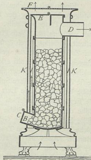
Meidinger-Ofen. — 1/20 w. Gr.
