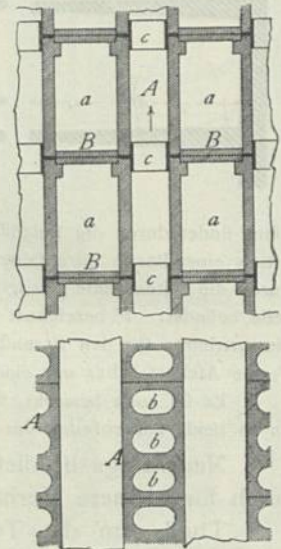
Luftheizungs-Ofen von Gaillard, Hailot &amp; Co. — 1/20 w. Gr.
