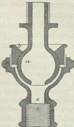
Kugelgelenk. — 1/2 w. Gr.
