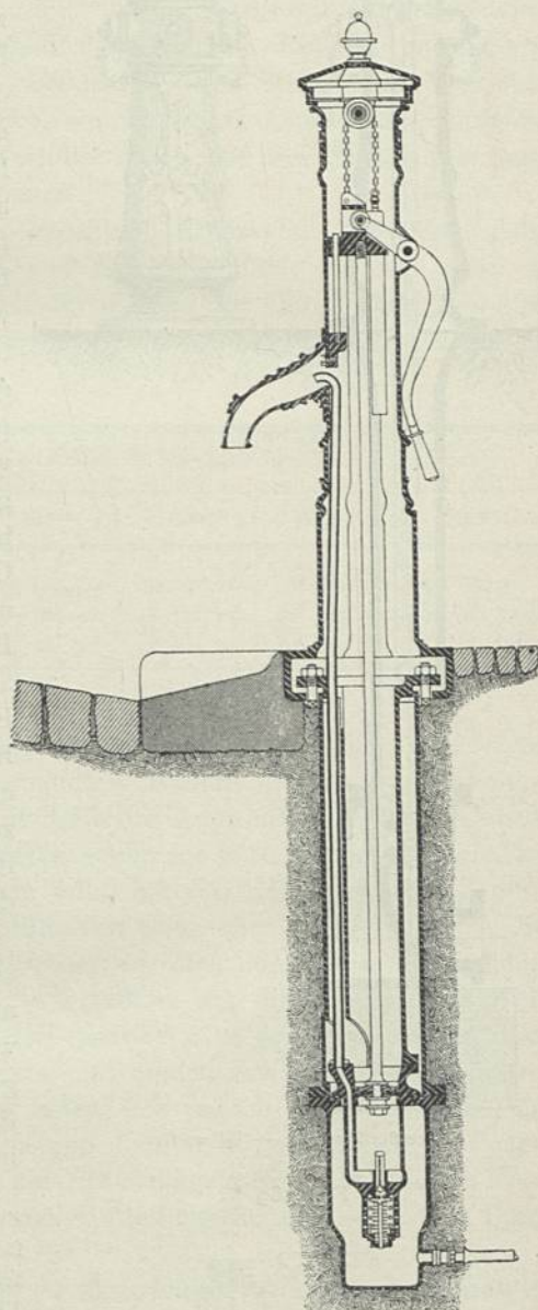
Auslaufftänder. — \frac{1}{20} w. Gr.
