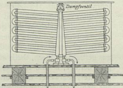
Warmwasser-Ofen von Käuffer &amp; Co. in Mainz.
