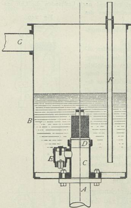
Ausdehnungsgefäß. — \frac{1}{10} w. Gr.
