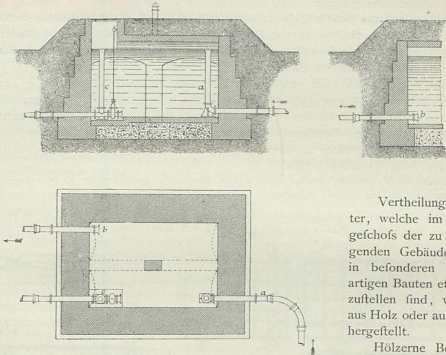
Gemauerter Vertheilungsbehälter. — 1/200 w. Gr.
