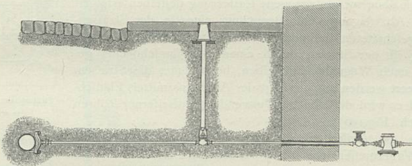
Abzweigungen von der Strafenleitung. — \frac{1}{50} w. Gr.
