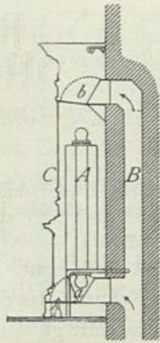
Heizkörper für Warmwasser-Heizung von Aird & Marc in Berlin. \frac{1}{60} w. Gr.
