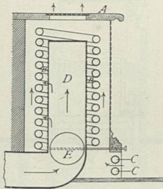
Wärmestrahler für Hochdruck-Heizung. 1/20 w. Gr.
