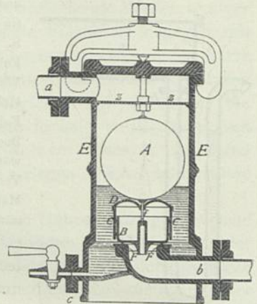
Selbstfleerer von Dehne in Halle a. S.
