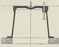
Deckel für Hydrantenröhren. — \frac{1}{25} w. Gr.
