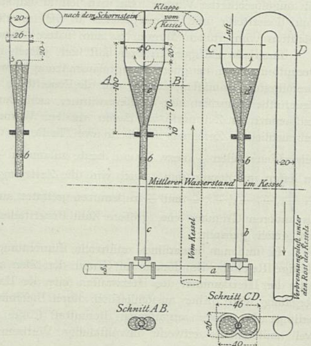
Selbstthätiger Regler von Käufer & Co. in Mainz.
