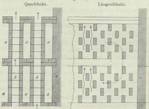
Luftheizungsöfen von Wiman. — 1/30 w. Gr.
