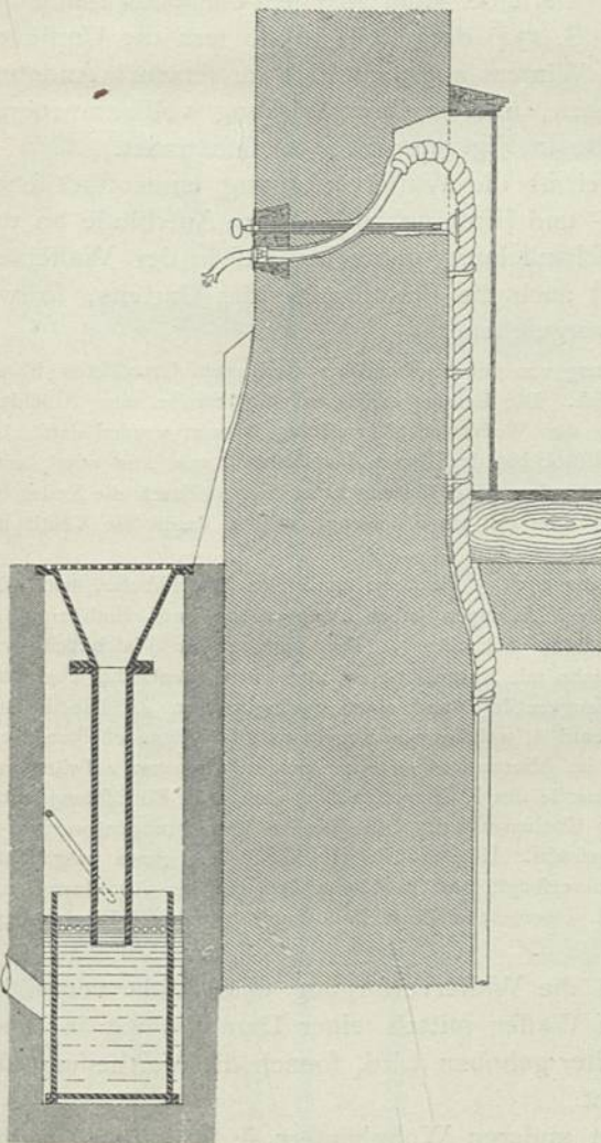
Wandbrunnen im Hofe. — \frac{1}{25} w. Gr.
