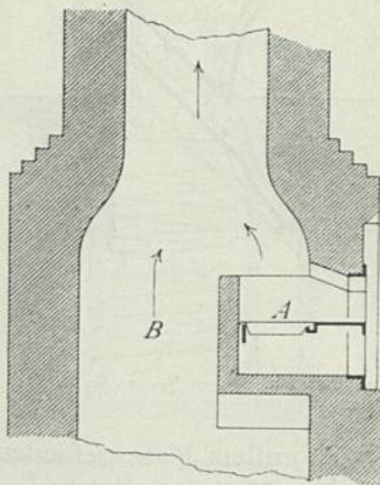
Lockschornstein mit Lockfeuer. 1/100 w. Gr.
