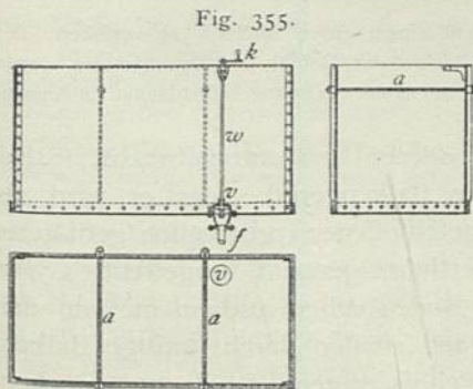
Gusseiserner Vertheilungsbehälter. — 1/100 w. Gr.
