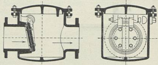
Klappenventil. — 1/25 w. Gr.
