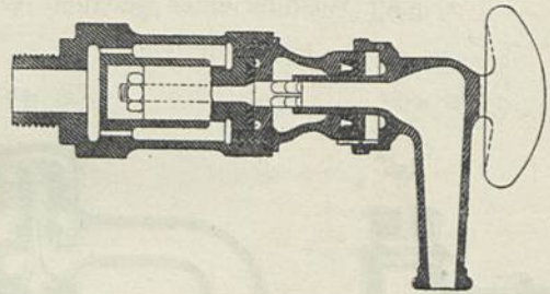
Selbstschlufs-Ventil von Knauff . — \frac{1}{3} w. Gr.
