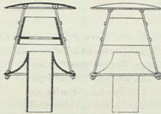
Saugkappe von Brüning.
