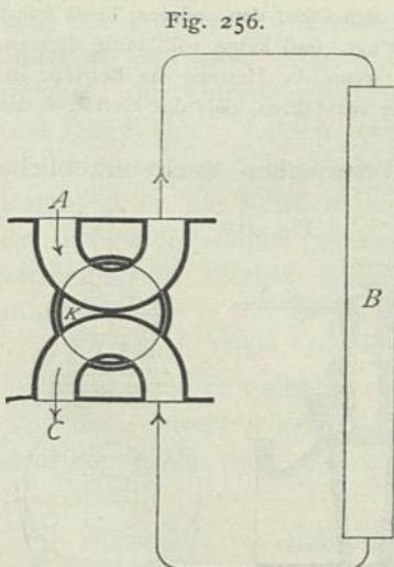
Wechselhahn von Wiman-Klein .
