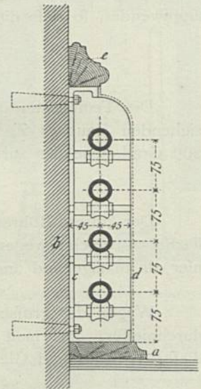
Röhrenanordnung für eine Hochdruck-Wasserheizung.
