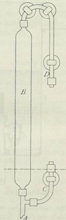
Ausdehnungsflasche. — \frac{1}{10} w.Gr.
