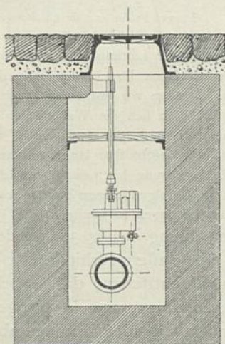
Im Schachte eingebauter Hydrant. \frac{1}{50} w. Gr.
