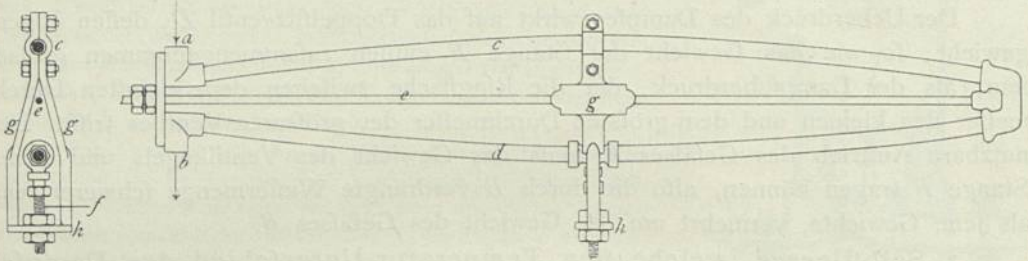
Selbstfleerer von Kufenberg.
