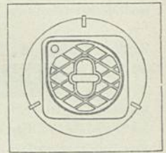
Strafenhahn mit Kappe. 1/10 w. Gr.
