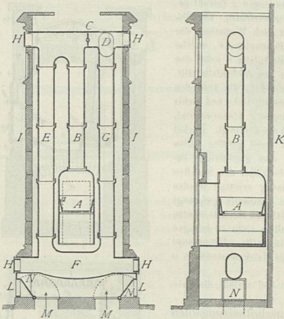
Ofen nach Rafsch. — \frac{1}{35} w. Gr.
