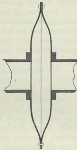
Längenausgleicher.
