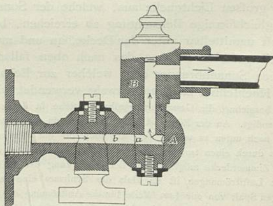
Gelenkrohr. — 2/3 w. Gr.
