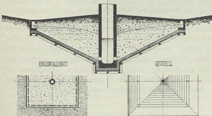
Venetianische Cisterne. — \frac{1}{150} , bzw. \frac{1}{450} w. Gr.
