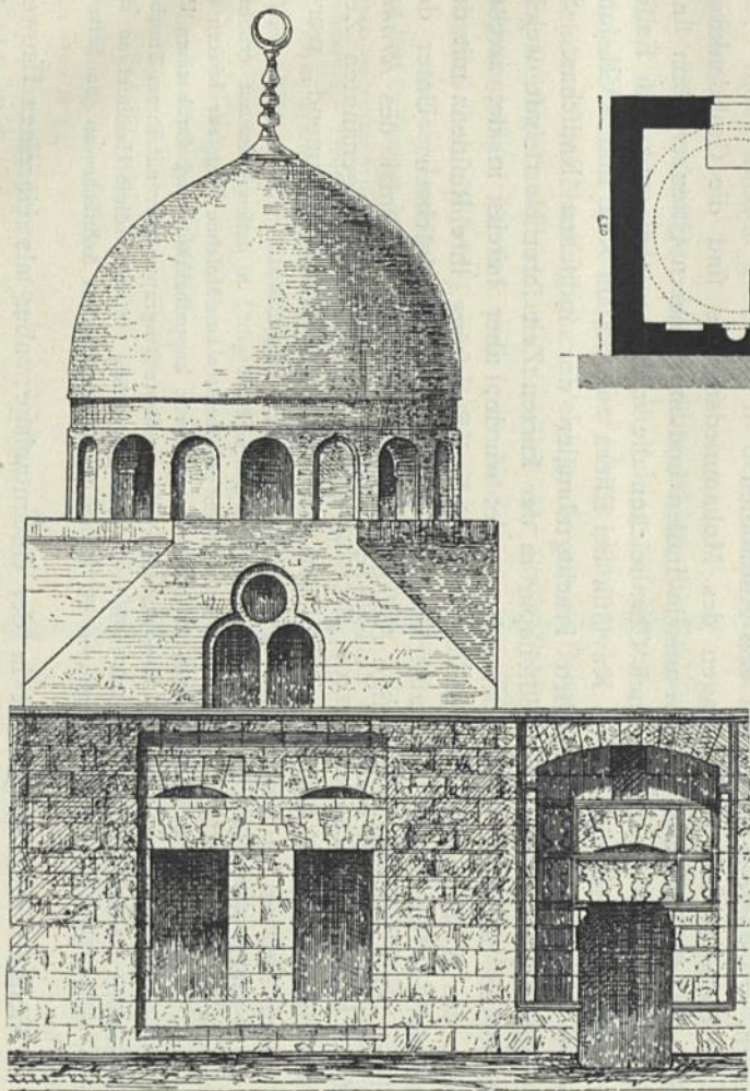
Mausoleum des Schech Ru'ey zu 'Kairo.
