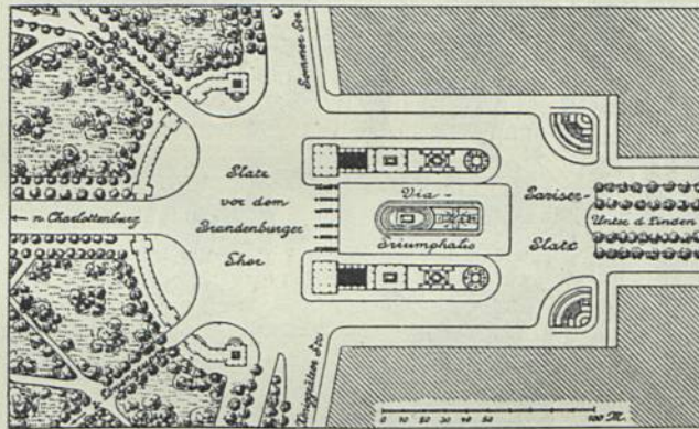
Entwurf für die Ausgestaltung des Platzes vor dem Brandenburger Thor zu Berlin von Ende & Föckmann , sowie Hartung .
