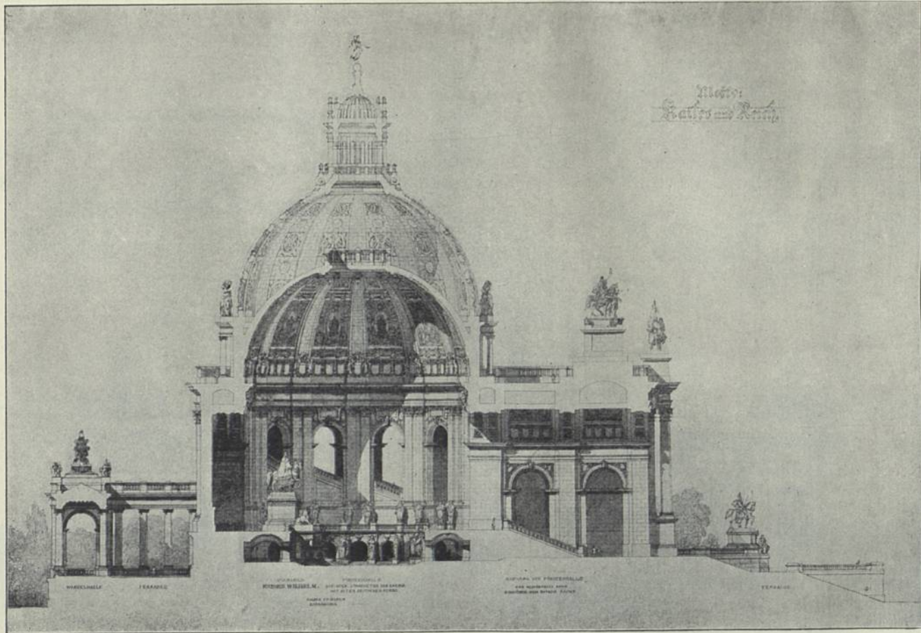
Querschnitt zu Fig. 498, 500 u. 501.
