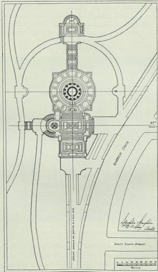
Lageplan und Grundriß zu Fig. 327 305 ).
