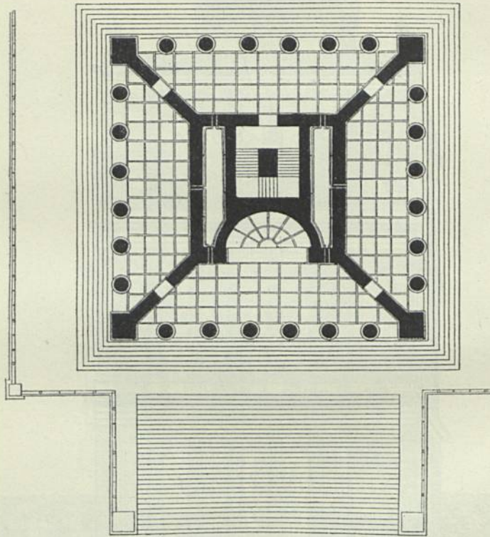
Grundriis zu Fig. 343.
