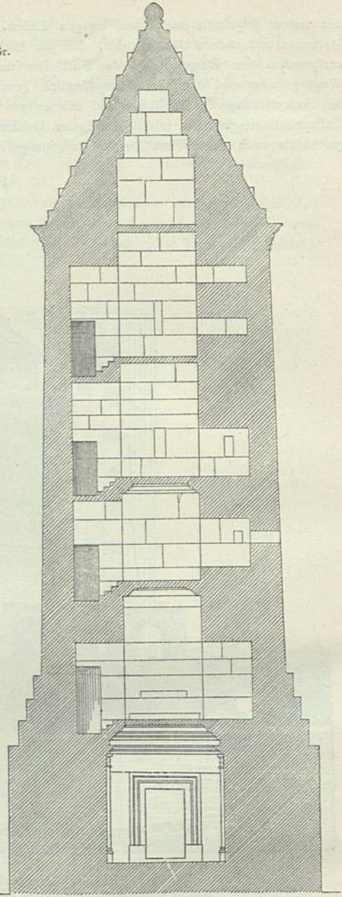
Lotrechter Schnitt.
