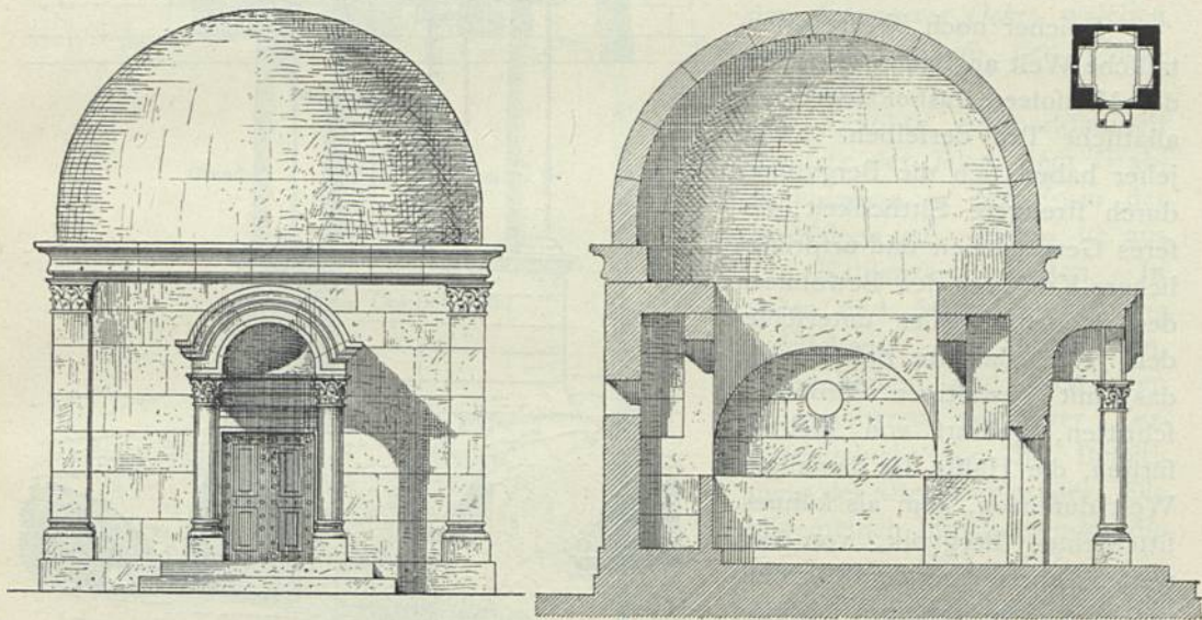
Grabmal des Bizzos zu Ruweha.
