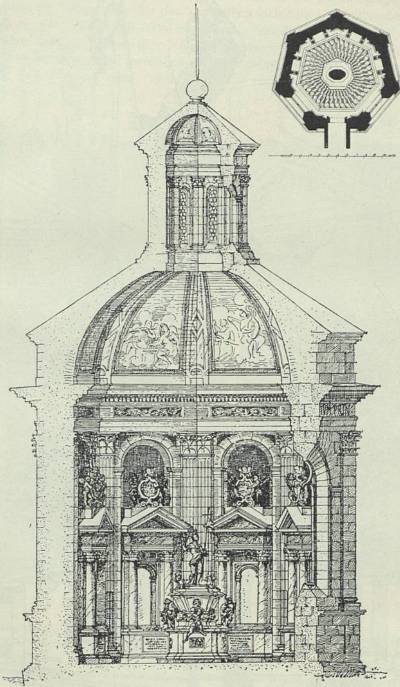
Mausoleum des Fürsten Ernst von Schaumburg zu Stadthagen 270 .
