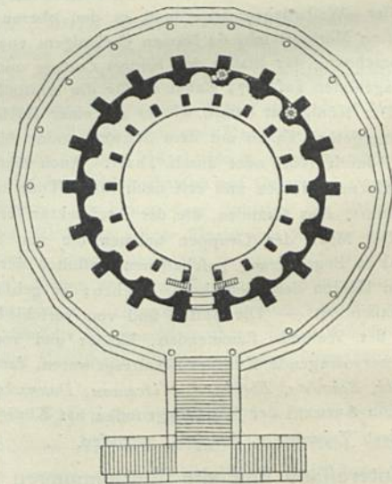
Befreiungshalle bei Kelheim. 1/1000 w. Gr.
