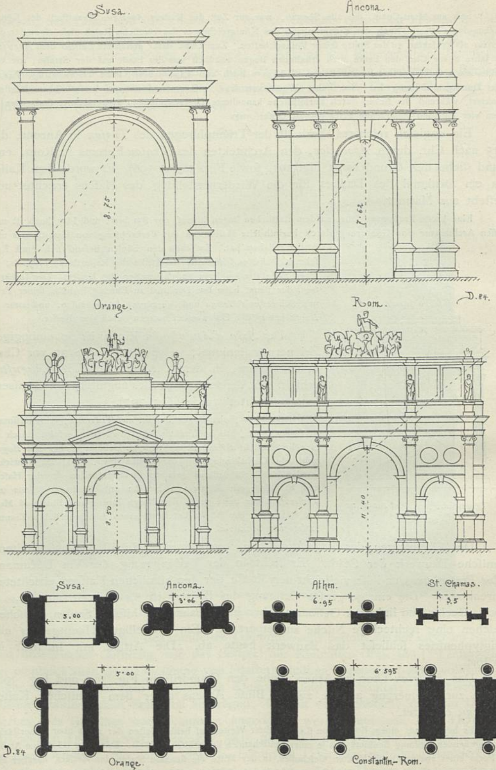
Zusammenstellung einiger römischer Triumphbogen-Systeme.
