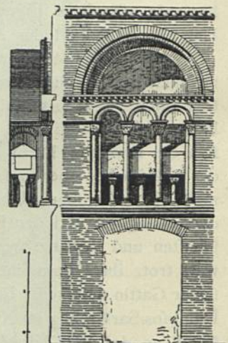
Von der Kirche der Chartreuse zu Toulouse.
