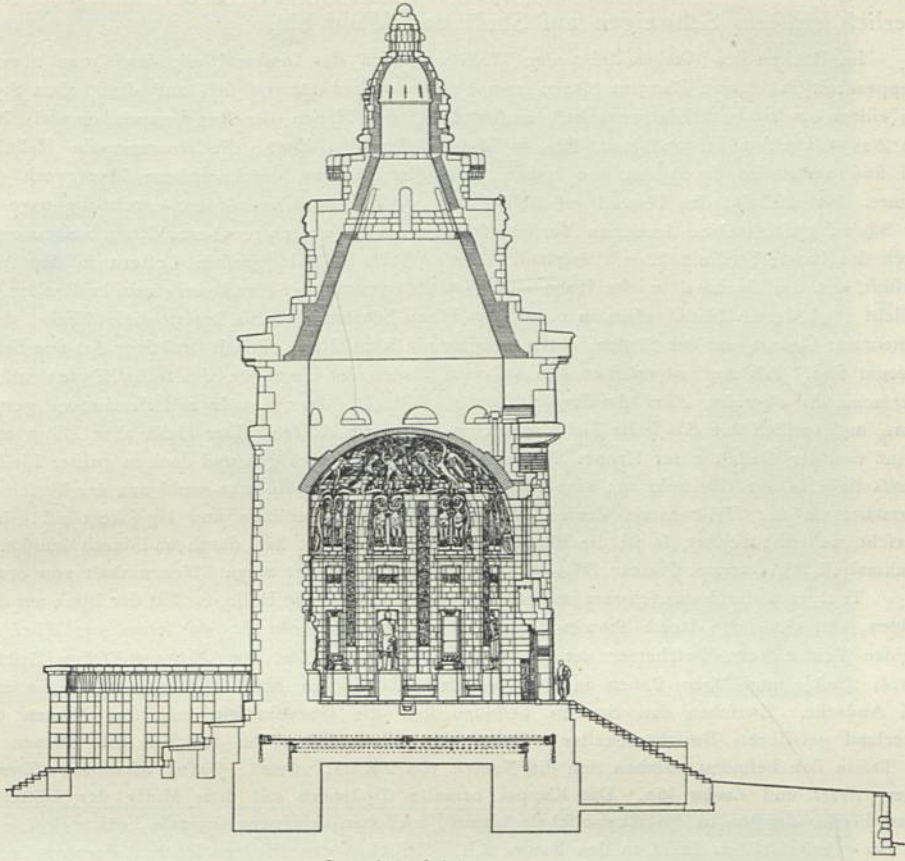
Lotrechter Schnitt.
