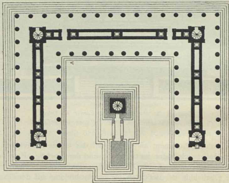
Grundrifs.
