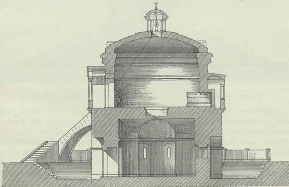
Grabmal des Theodorich bei Ravenna nach dem Wiederherstellungsversuch von A. v. Effenwein .
