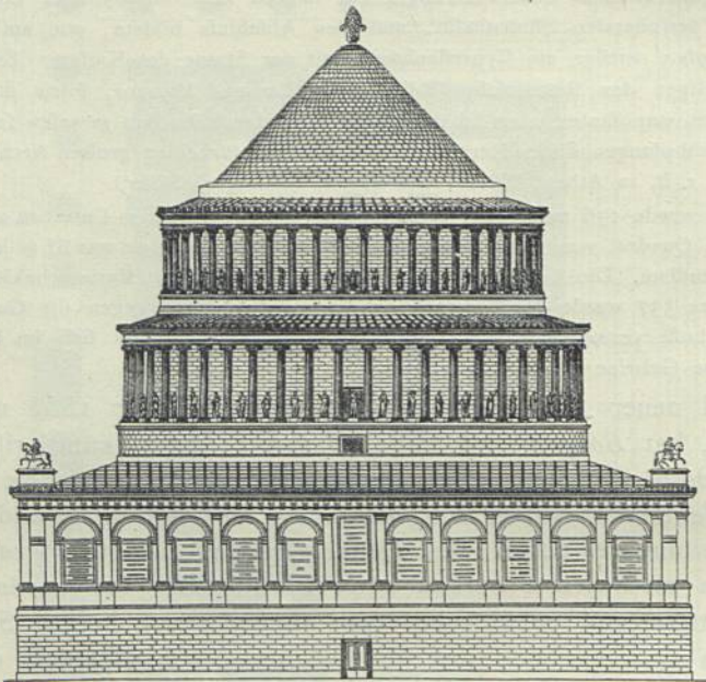
Grabdenkmal des Kaisers Hadrian zu Rom. Wiederherstellungsversuch von Canina 258).
