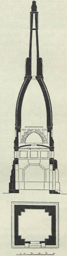
Lotrechter und wägrechter Schnitt.
