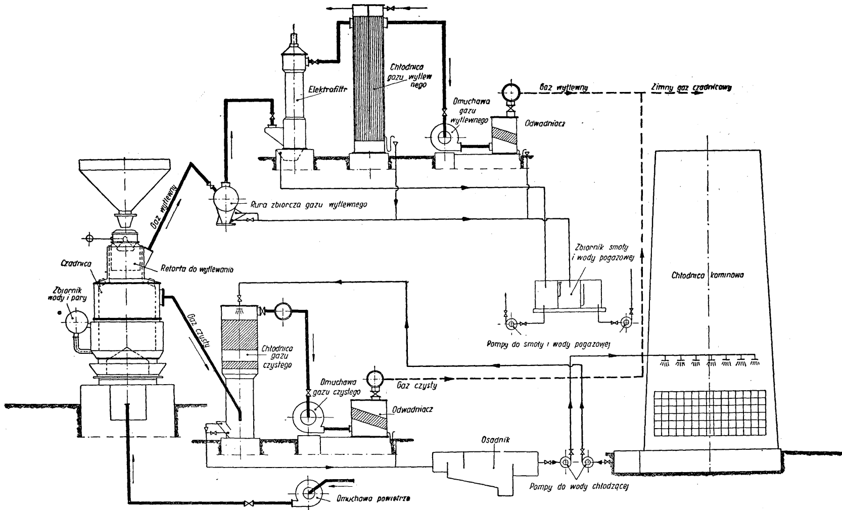
Rys. 1. Typowy układ czadnicy z otrzymywaniem gazu wylewnego
