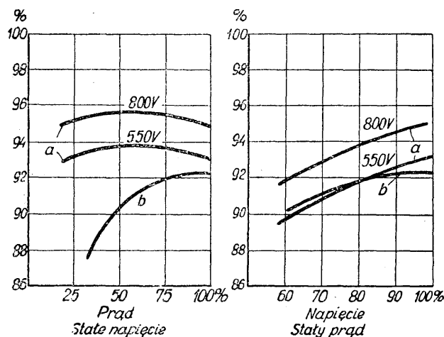
Rys. 4. Sprawność przetwornicy b i prostownika dużej mocy a
