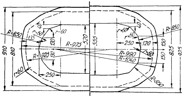
Rys. 3. Próbnny, nowy kształt wlewnicy dla wlewka o ciężarze 6 t
