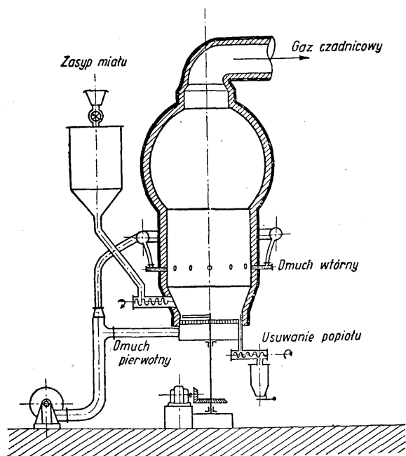
Rys. 3. Czadnica Winklera
