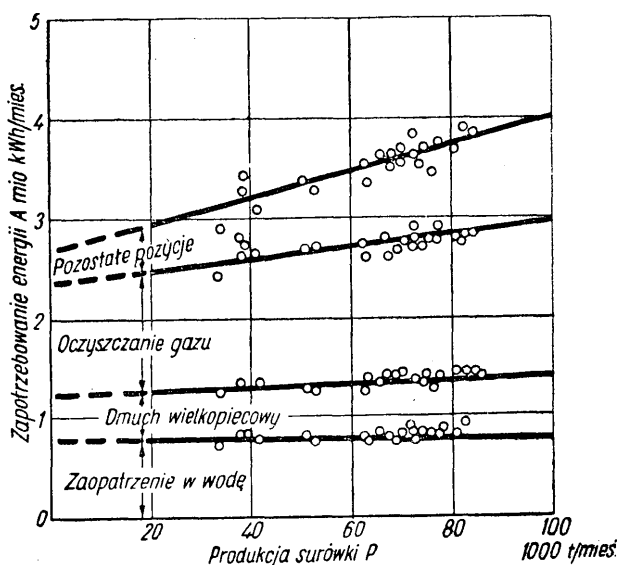
Rys. 3. Charakterystyka elektryczna wydziału wielkopieczowego
