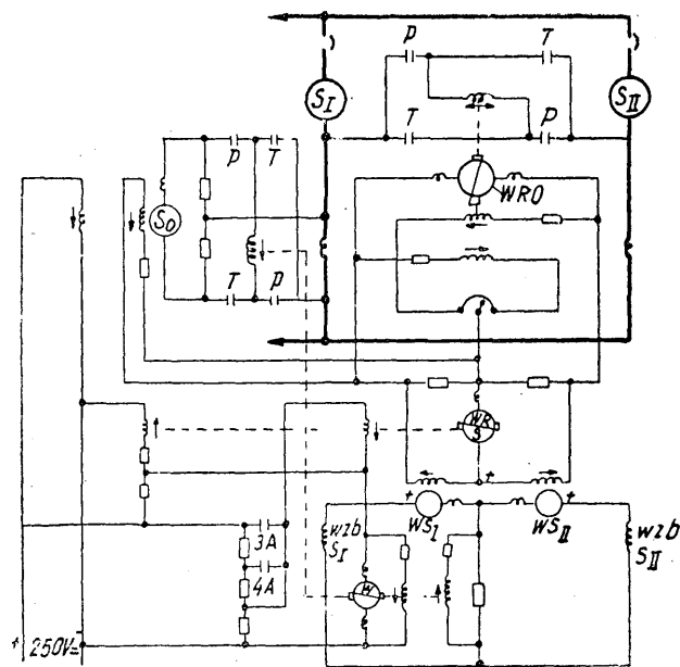
Rys. 4. Układ amplidynowy wzbudzenia pól w silnikach zespolonych
