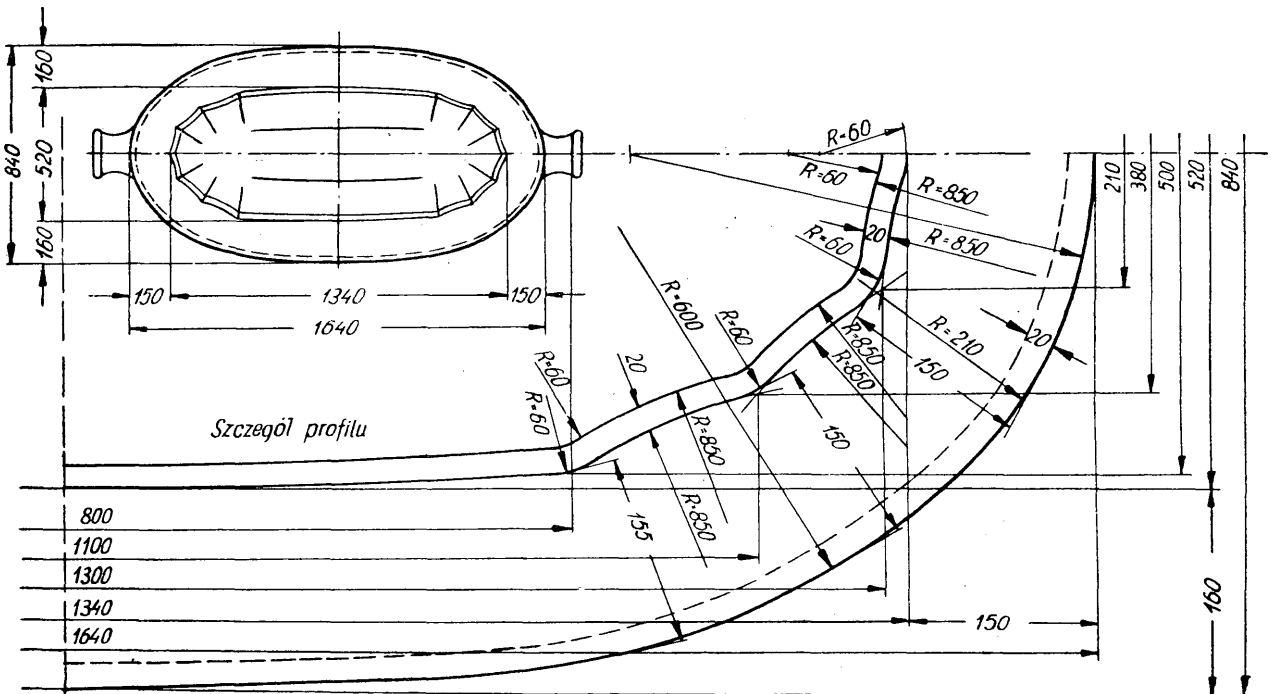
Rys. 4. Ostateczny kształt wlewnicy dla wlewków płaskich o ciężarze 7,2 t
