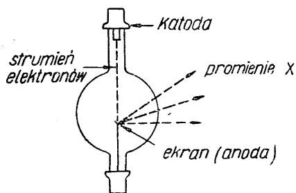
lampa Roentgena
