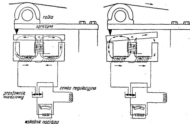
Rys. 7. Schemat obrazujący zasadę działania tensjometru
