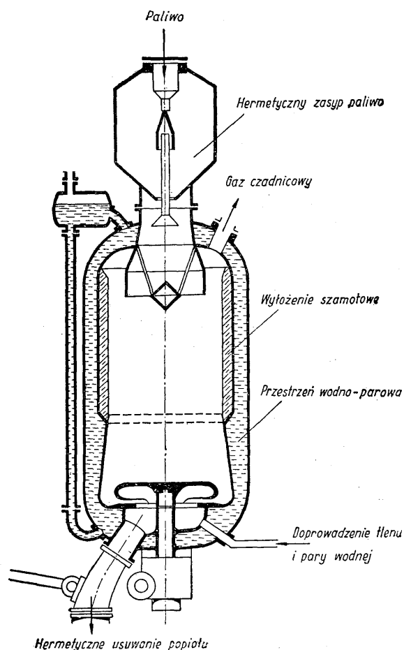
Rys. 2. Czadnica firmy Lurgi
