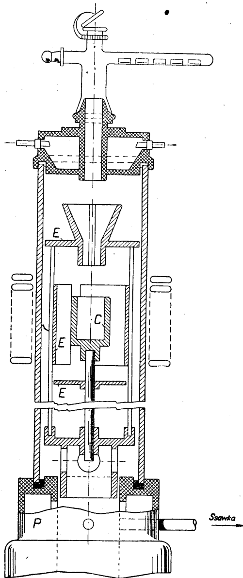
Rys. 3 Aparatura L. Morcau do określenia tlenu w stali.
